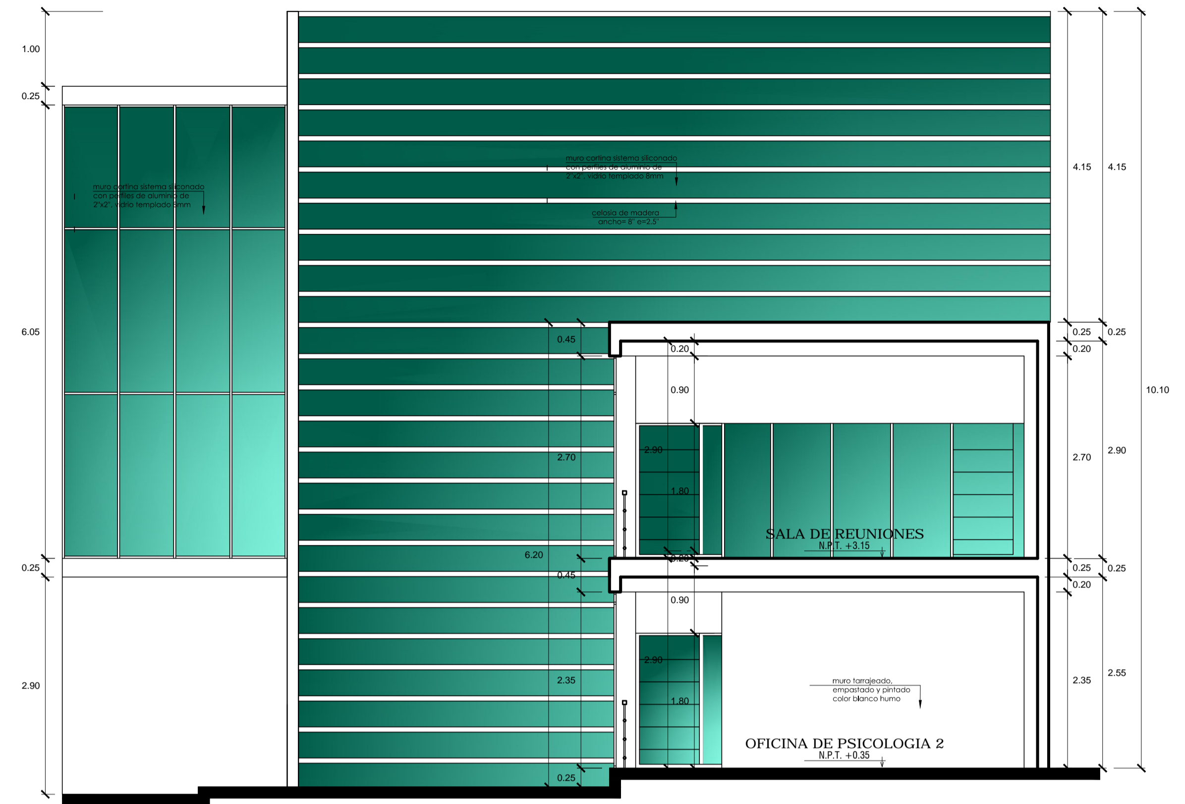
CORTE E - E esc:1/50
