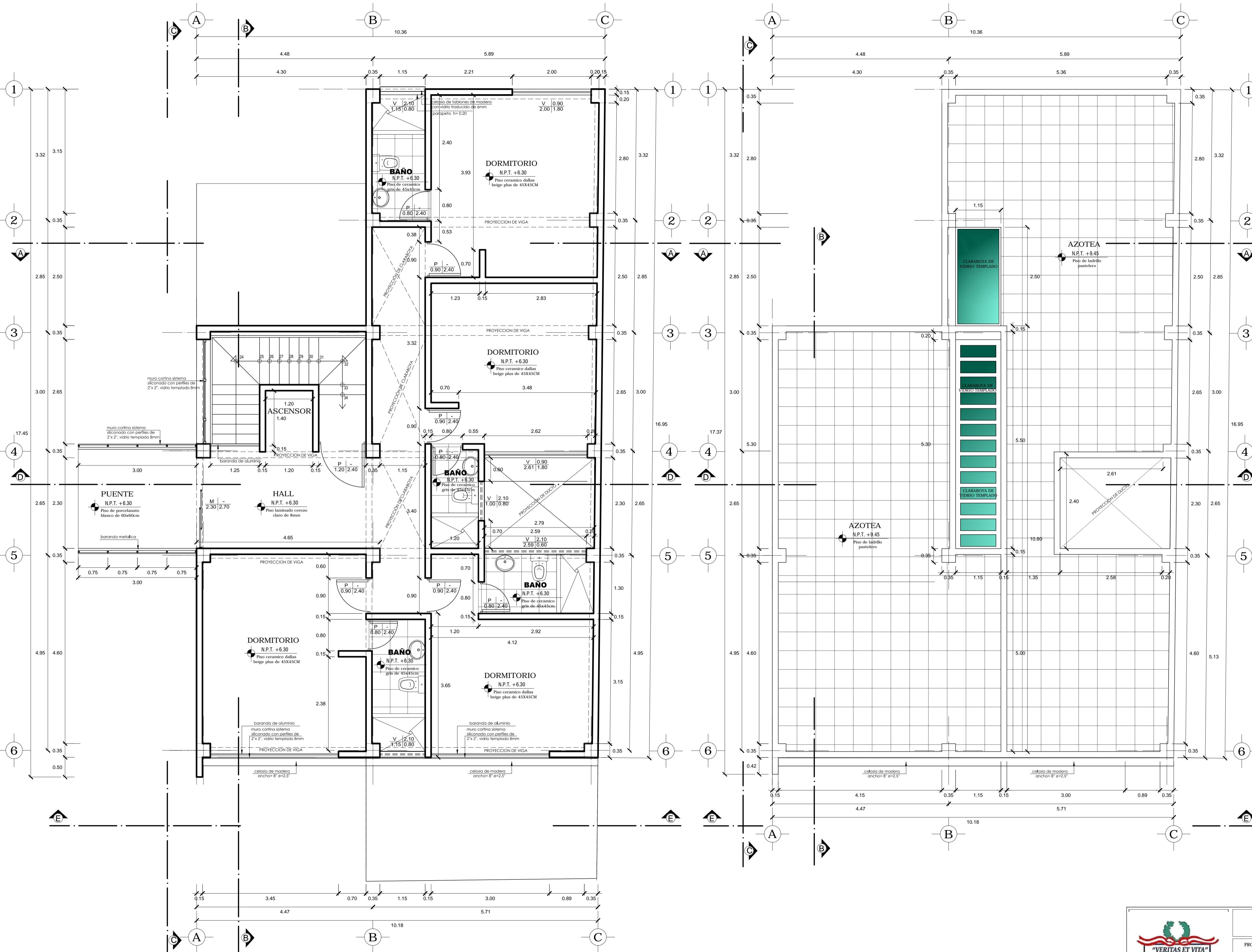
TERCERA PLANTA esc:1/50
