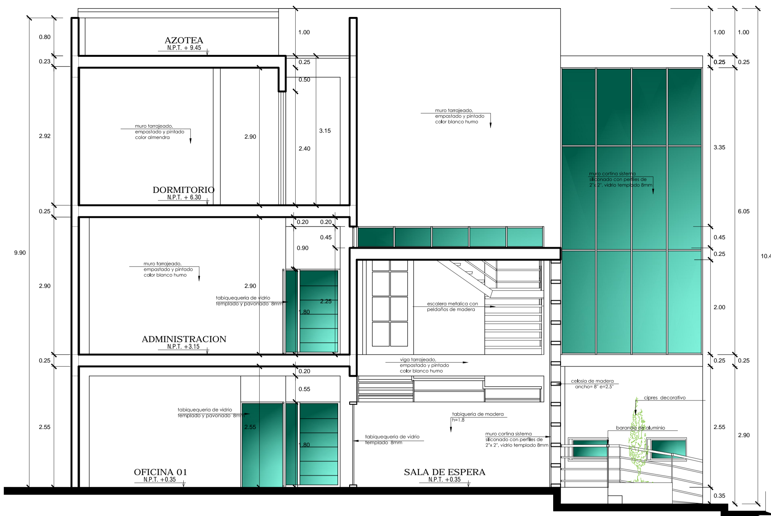
CORTE A - A esc:1/50
