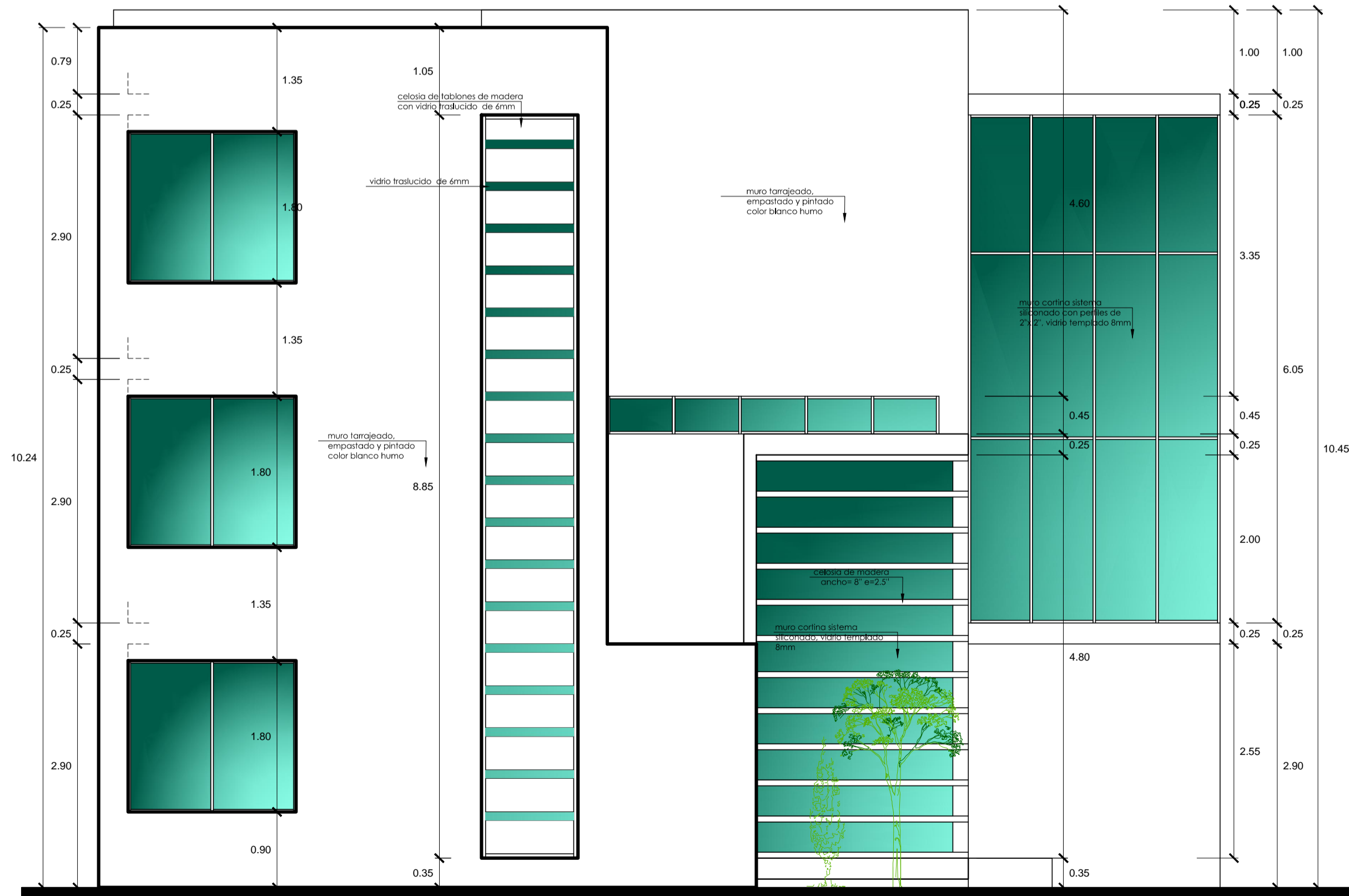
ELEVACION PRINCIPAL esc:1/50
