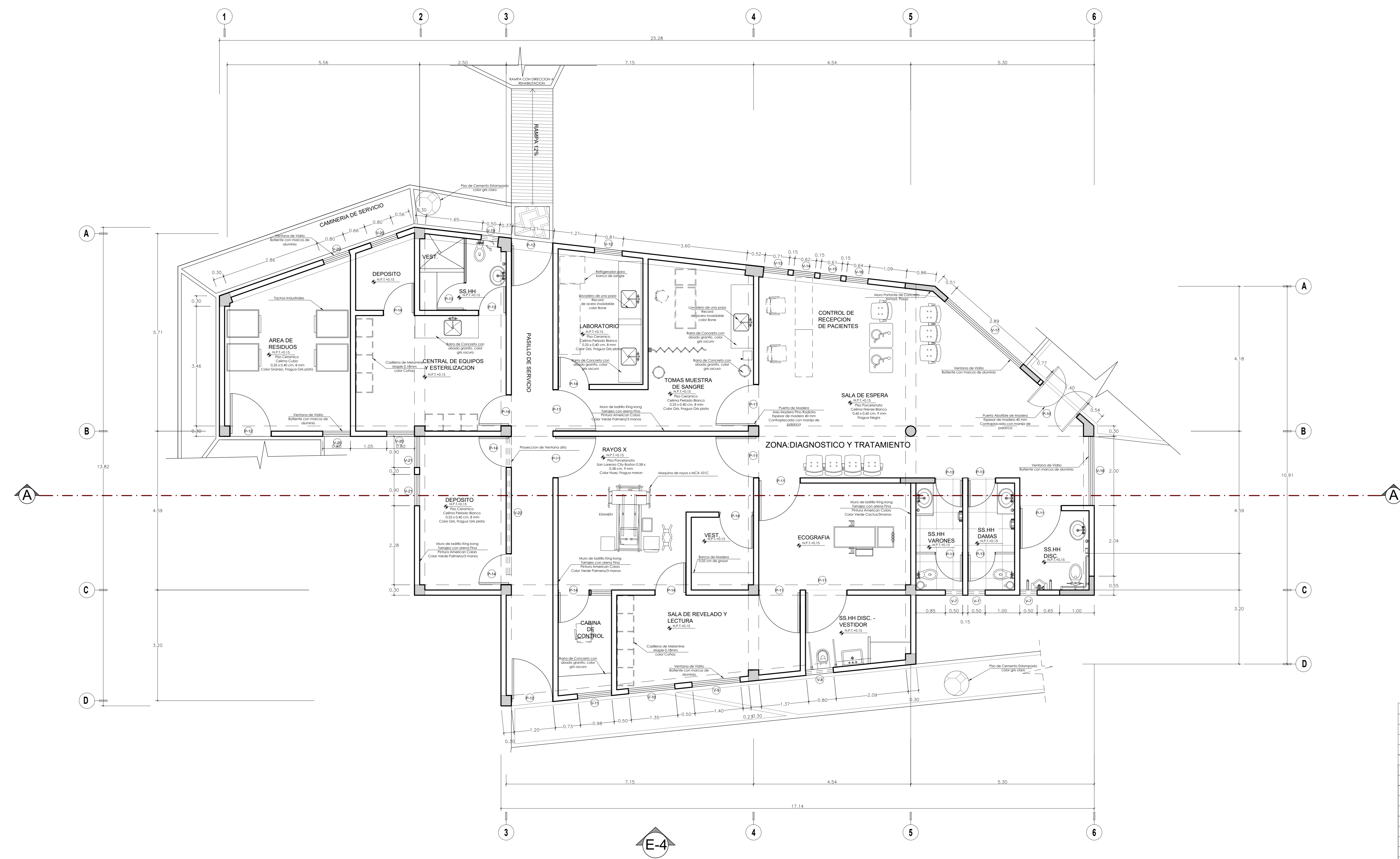
PLANTA PRIMER NIVEL-DIAGNOSTICO Y TRATAMIENTO ESC.1/50
