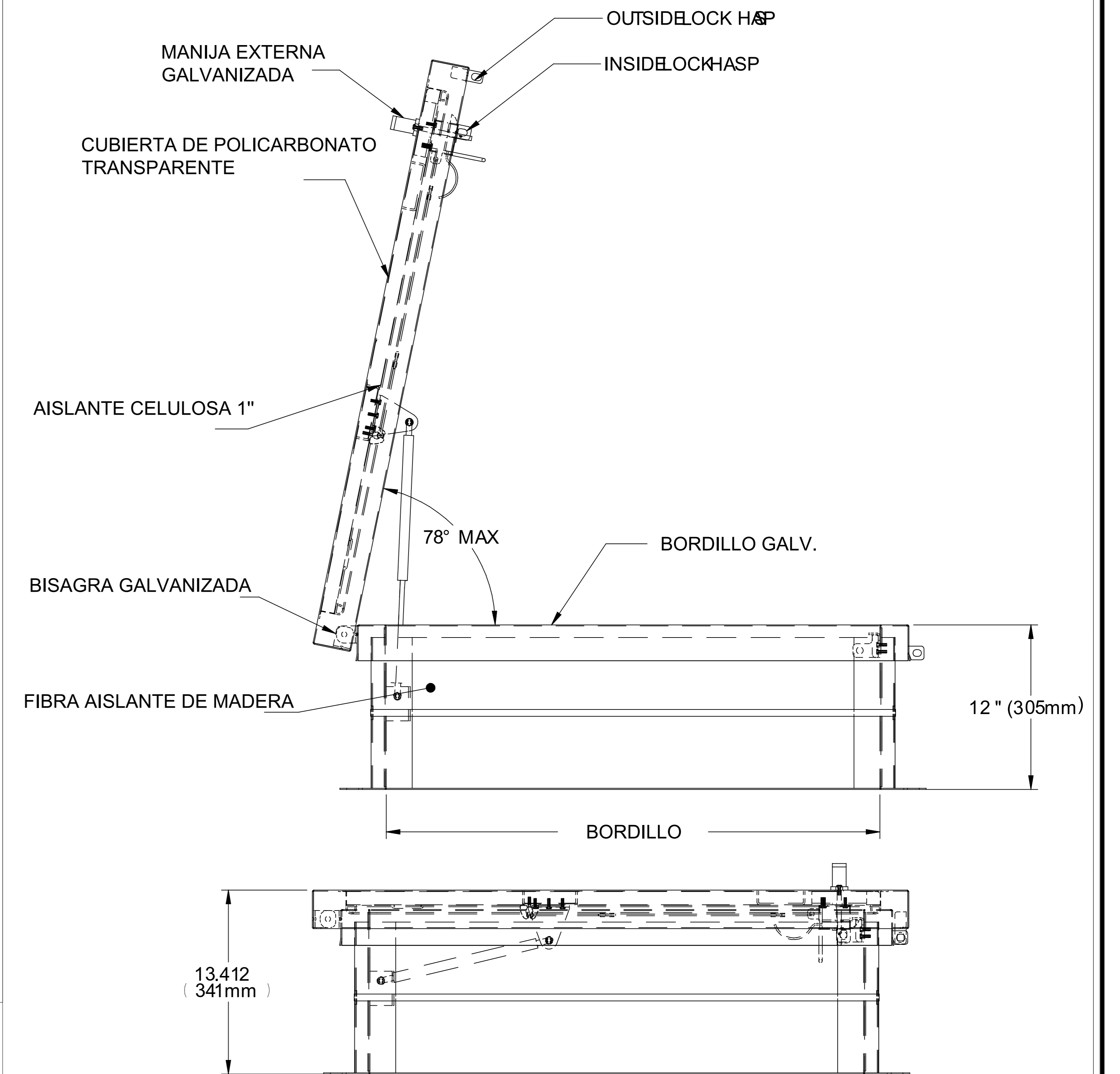
DETALLE 02 ESC.1/5
