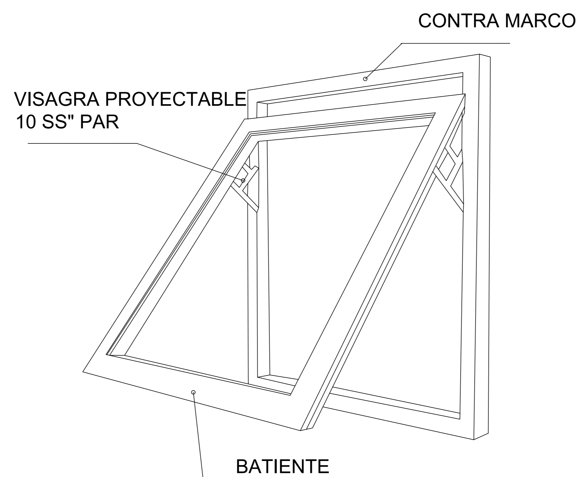
ISOMETRICO DE VENTANA BATIENTE
