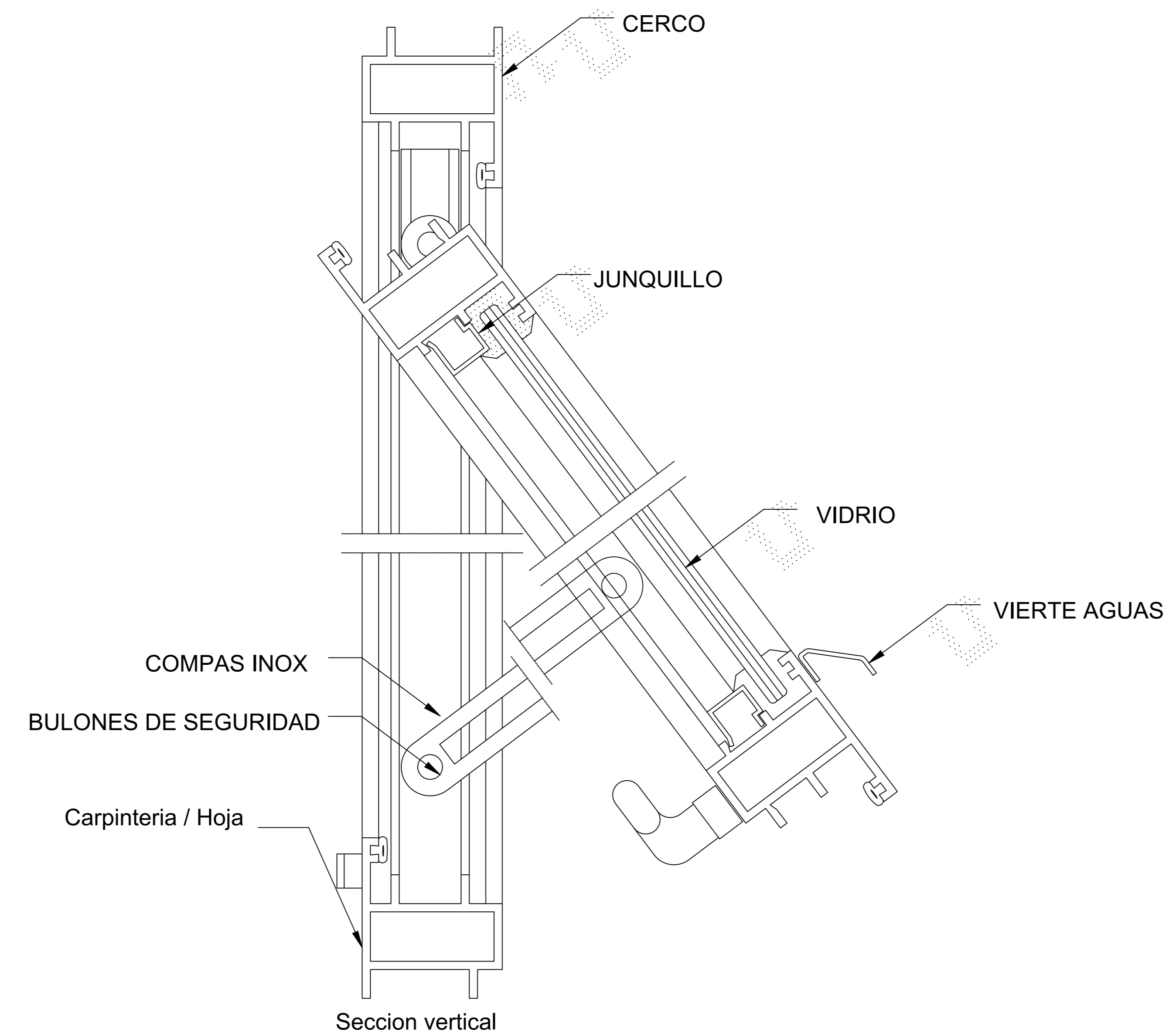
DETALLE 01 ESC.1/5
