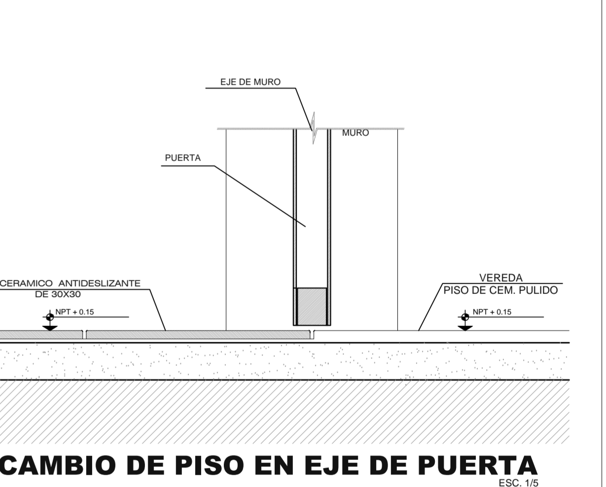
CAMBIO DE PISO EN EJE DE PUERTA ESC: 1/5
