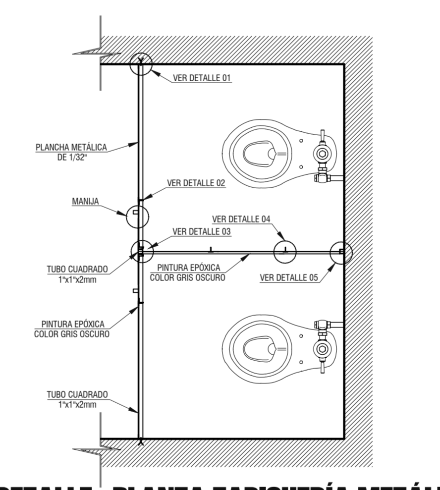
DETALLE: PLANTA TABIQUERIA METALICA ESC: 1/20
