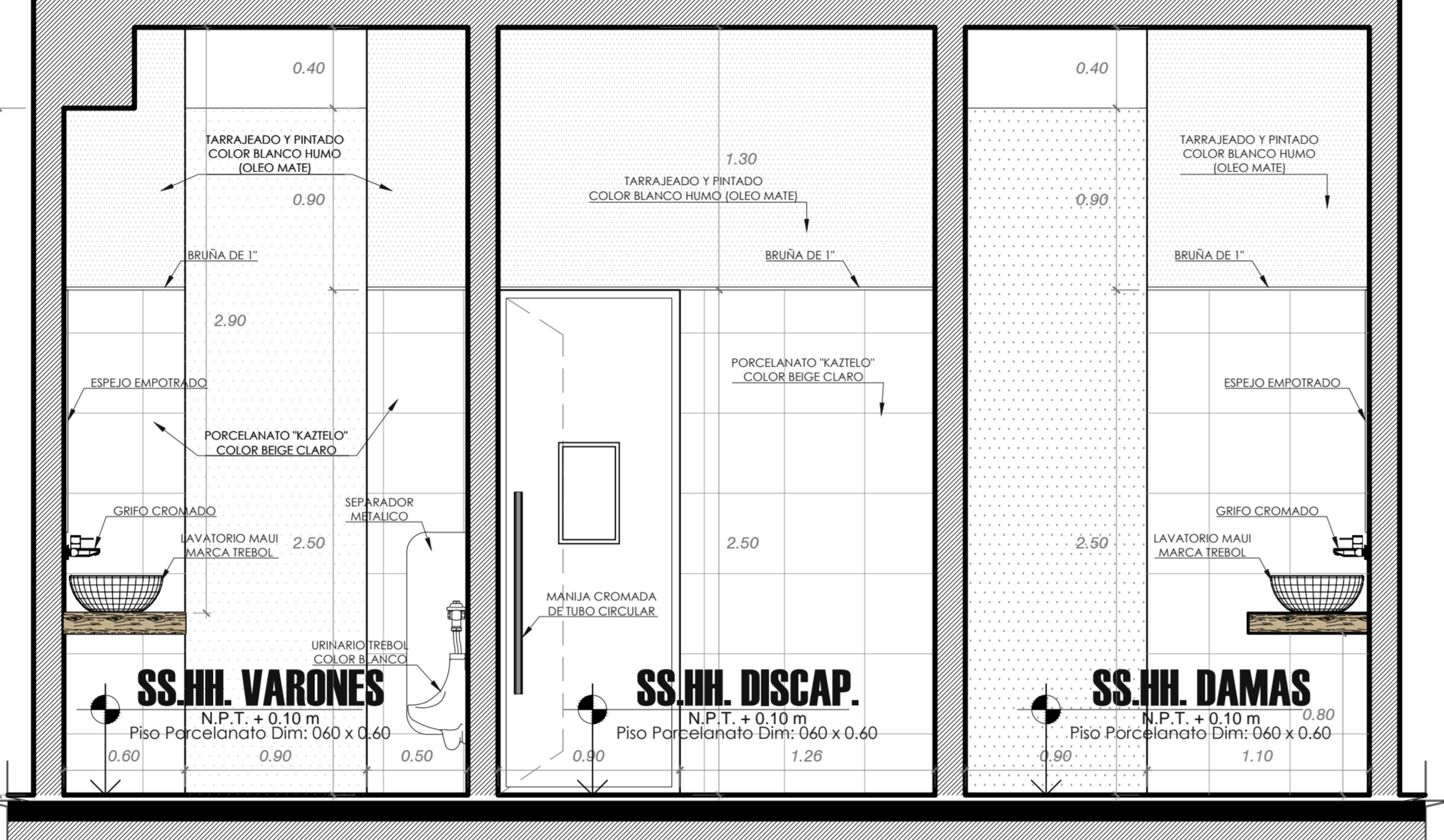
BATERIA DE BAÑOS TIPO A: CORTE B-B ESC: 1/25
