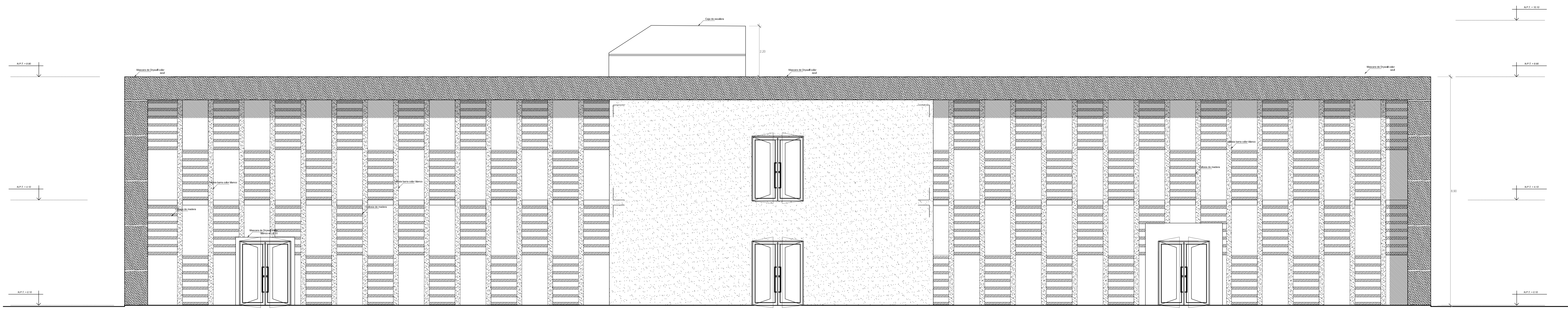
ELEVACION POSTERIOR E-4 Escala: 1:50
