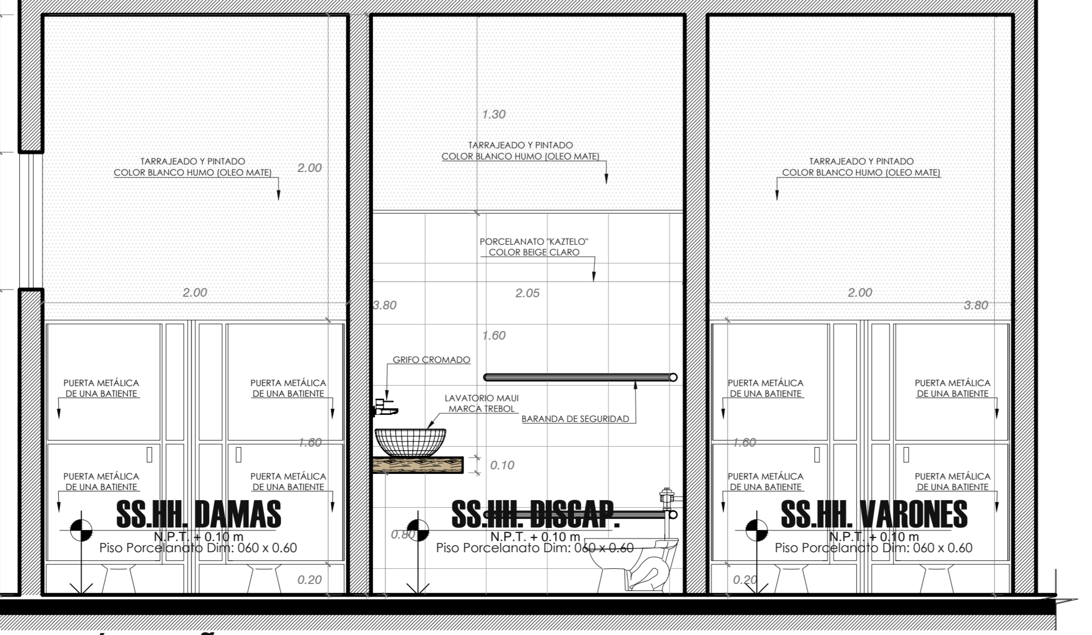
BATERIA DE BAÑOS TIPO B: CORTE B-B ESC: 1/25
