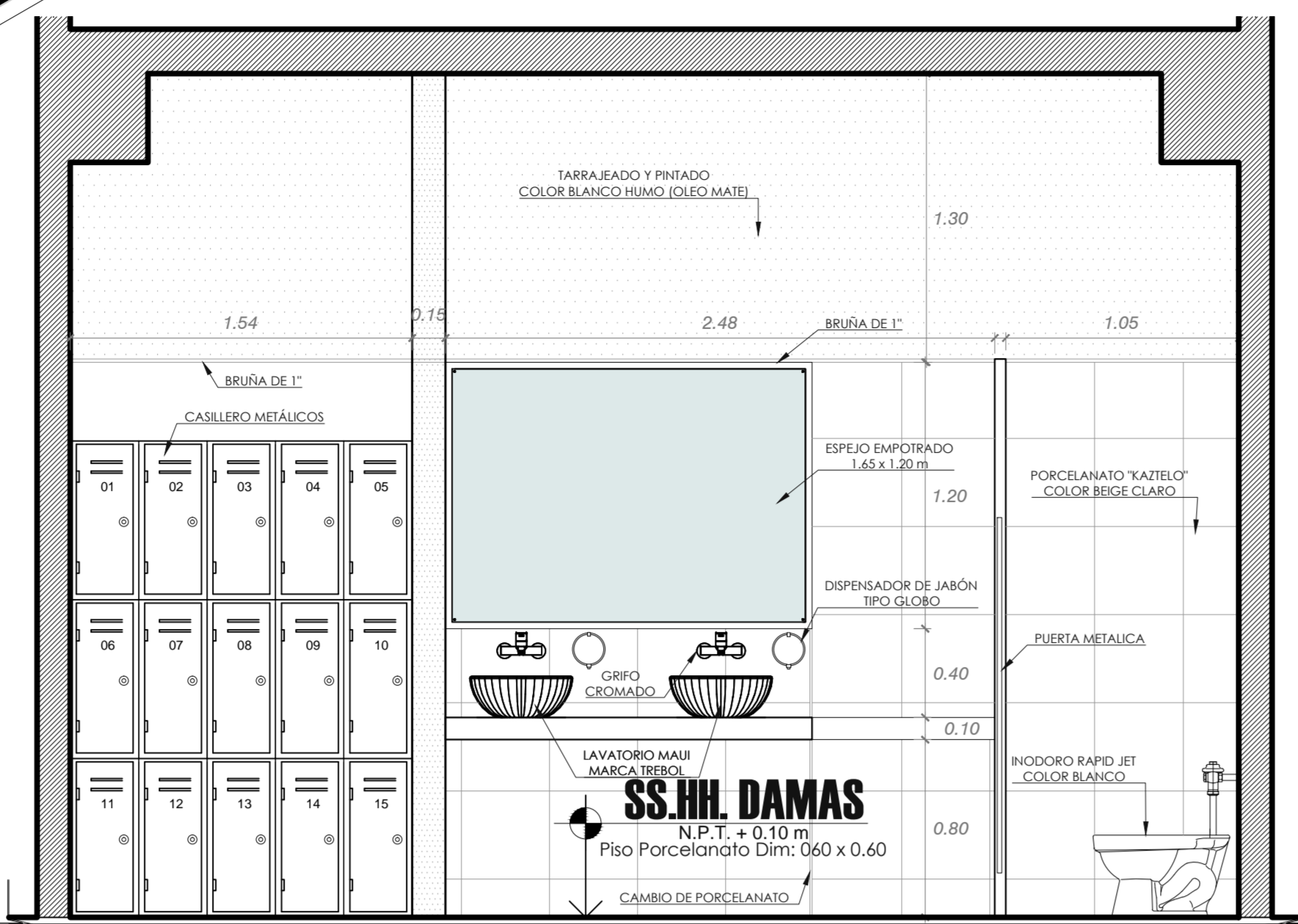
BATERIA DE BAÑOS TIPO A: CORTE A-A ESC: 1/25
