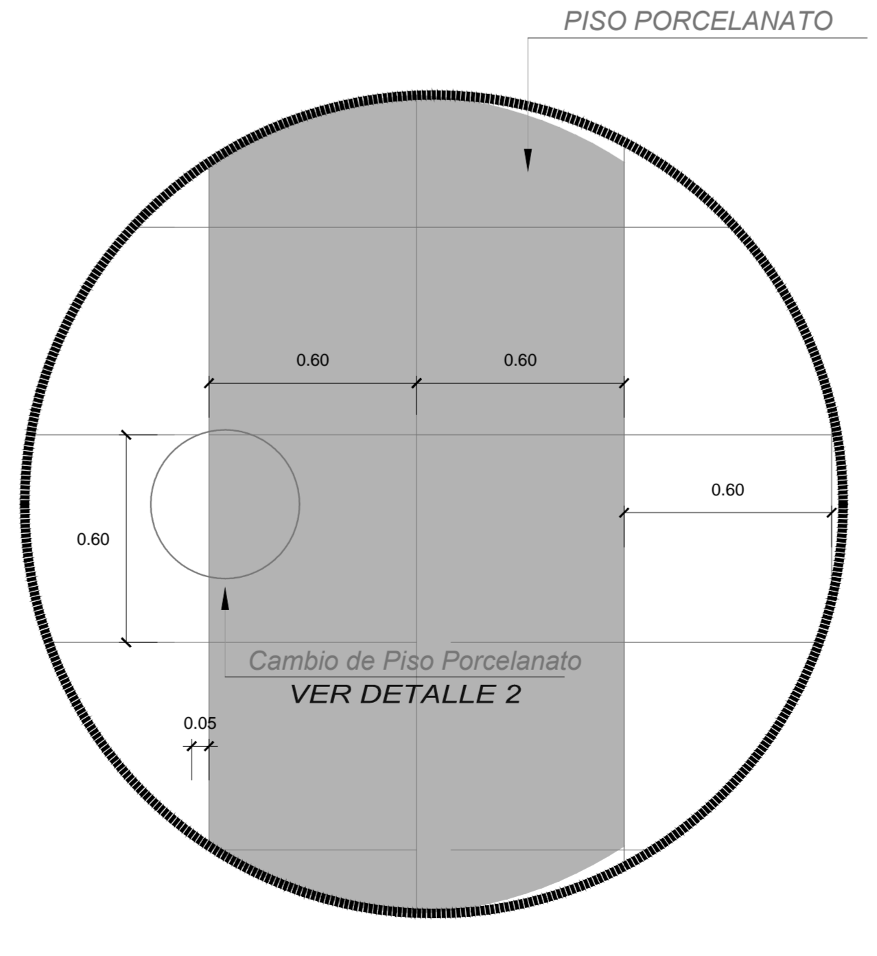
DETALLE 01 ESC: 1/5 PISO DE PORCELANATO 0.60 x 0.60
