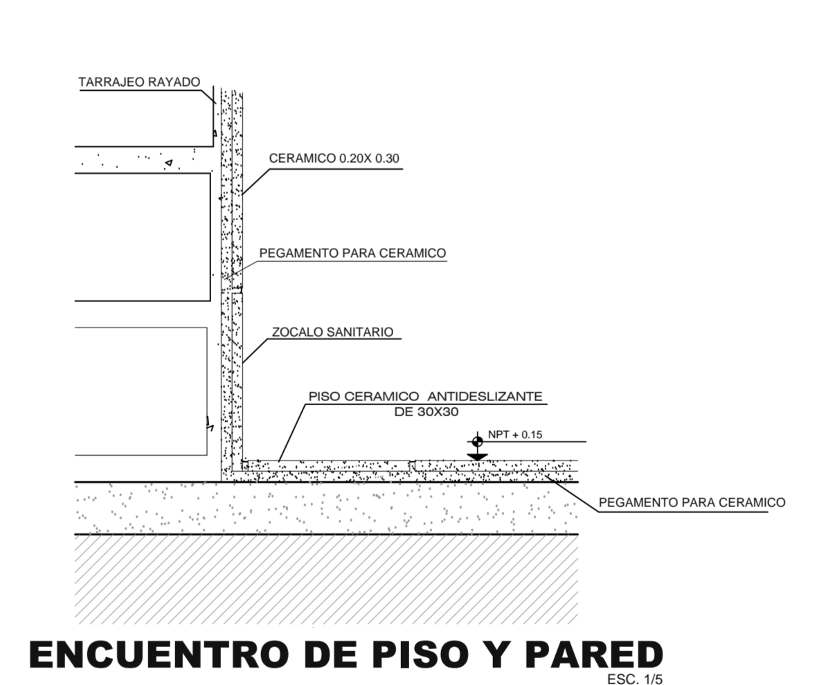
ENCUENTRO DE PISO Y PARED ESC: 1/5
