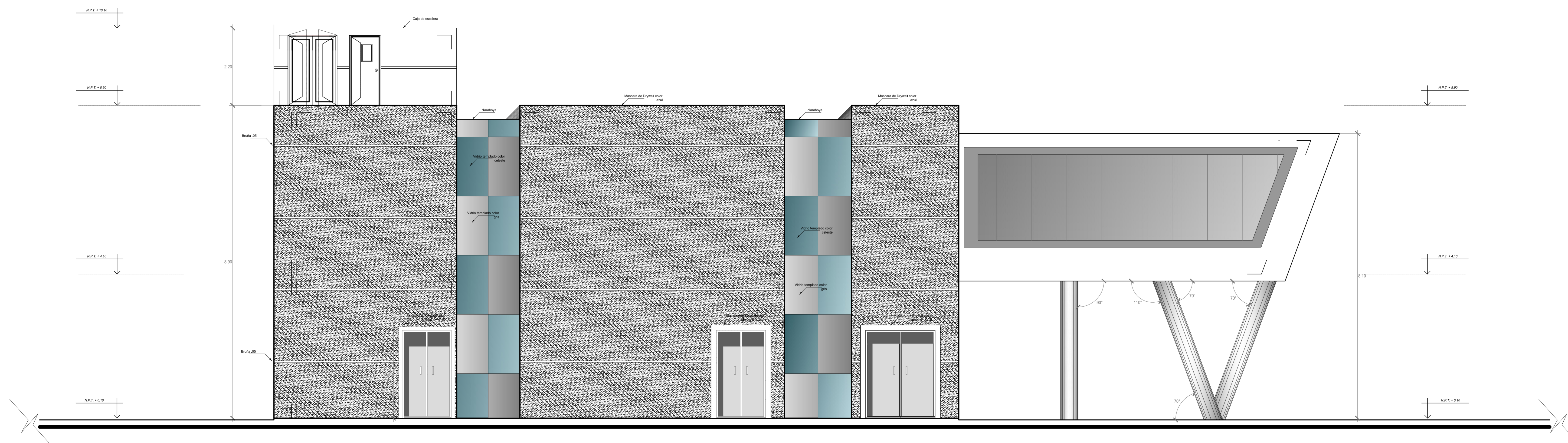
ELEVACION LATERAL E-2 Ebc: 1/50
