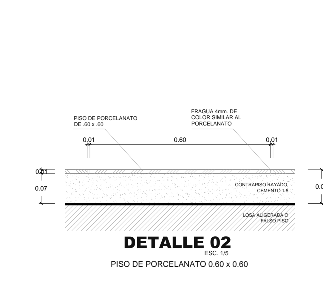
DETALLE 02 ESC: 1/5 PISO DE PORCELANATO 0.60 x 0.60
