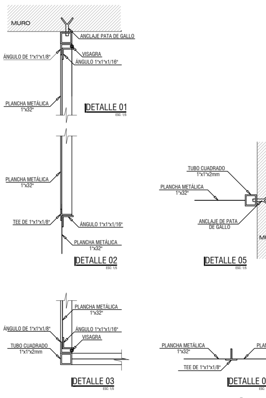
DETALLE DE ANCLAJES METALICOS ESC: 1/5
