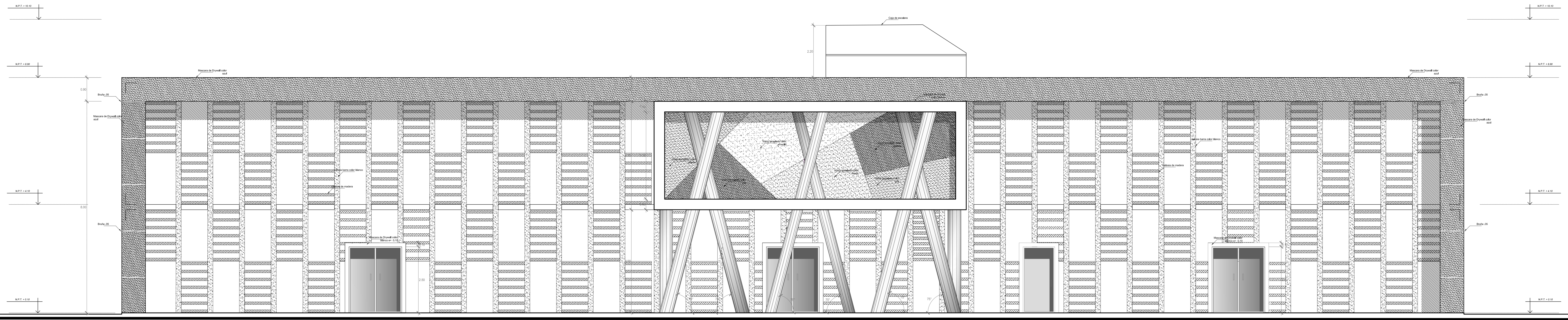
ELEVACION FRONTAL E-1 Ebc: 1/50
