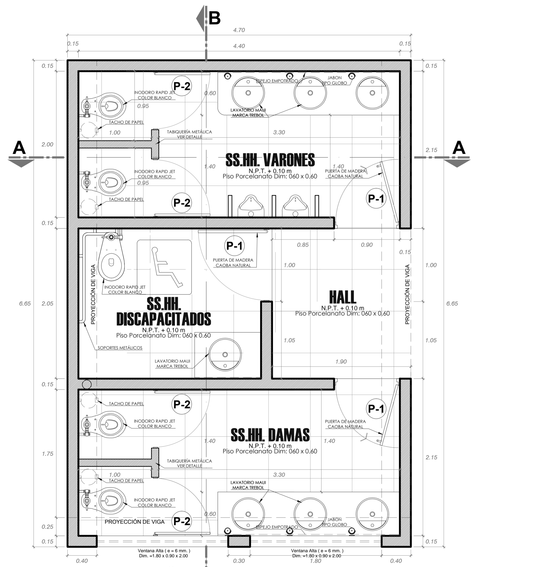
DETALLE DE BATERIA DE BAÑOS TIPO B ESC: 1/25
