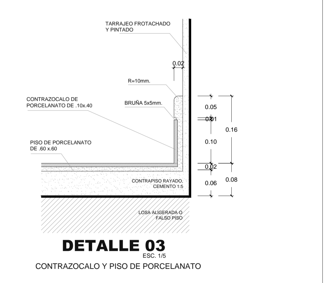
DETALLE 03 ESC: 1/5 CONTRAZOCALO Y PISO DE PORCELANATO
