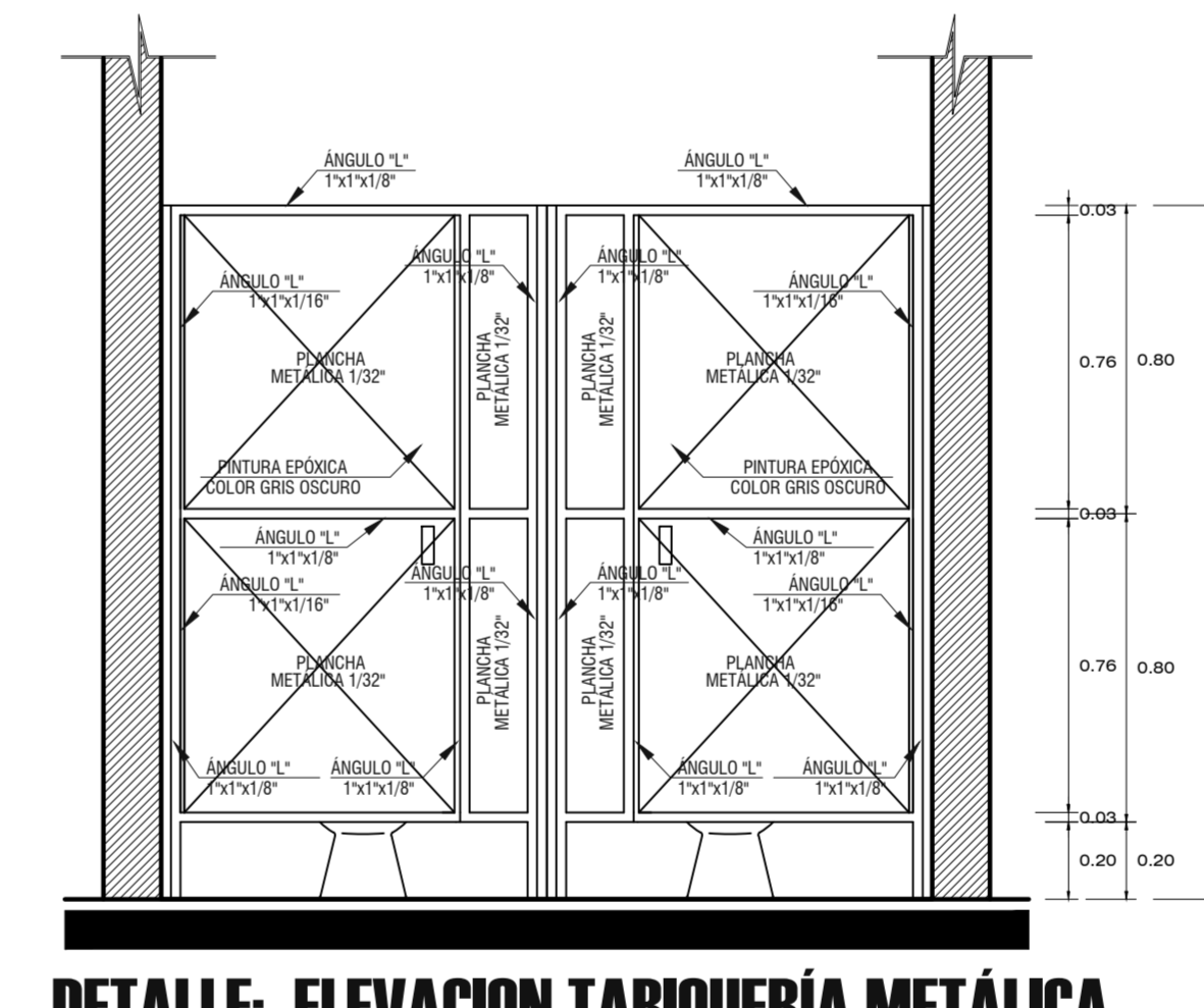
DETALLE: ELEVACION TABIQUERIA METALICA ESC: 1/20
