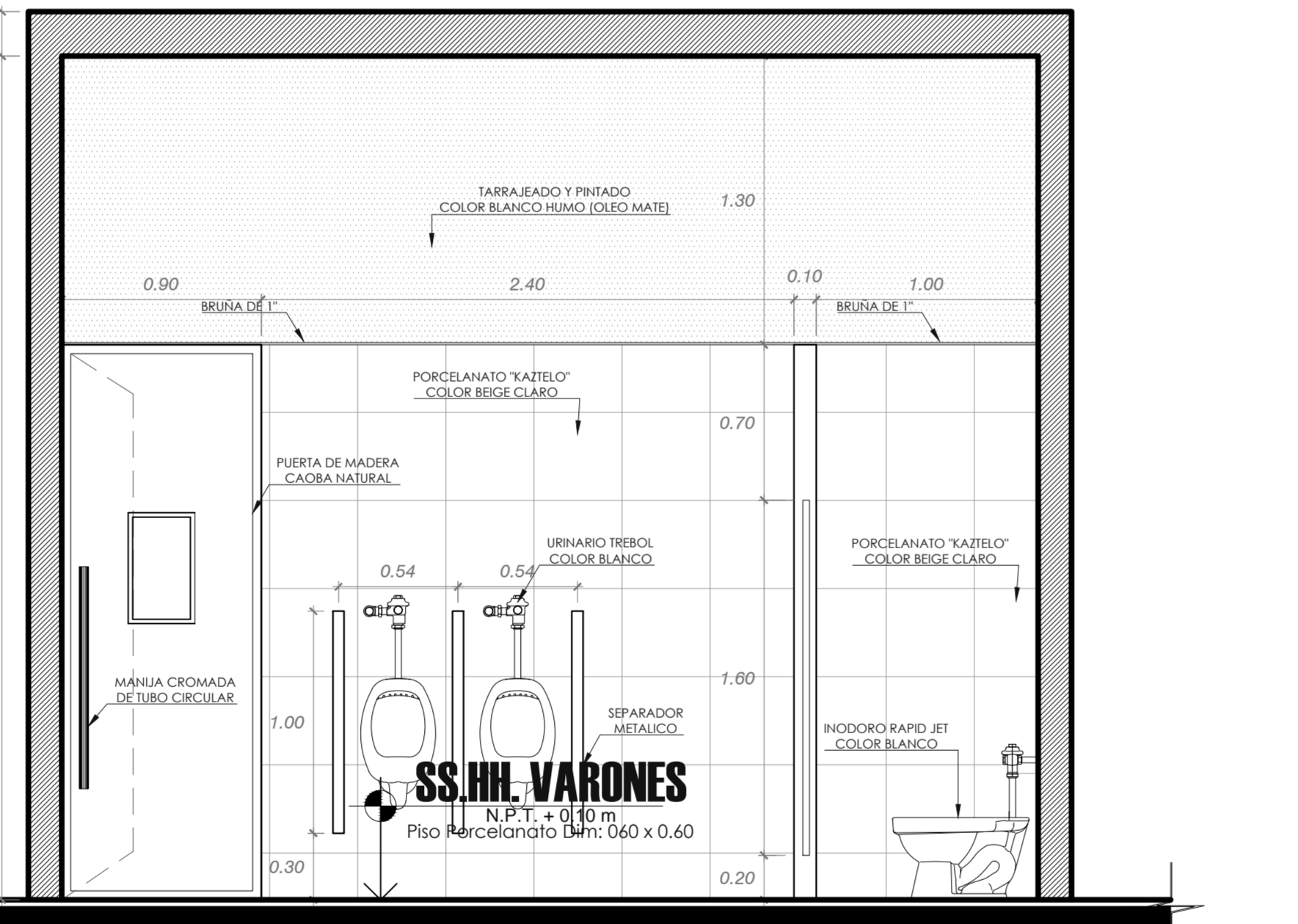
BATERIA DE BAÑOS TIPO B: CORTE A-A ESC: 1/25
