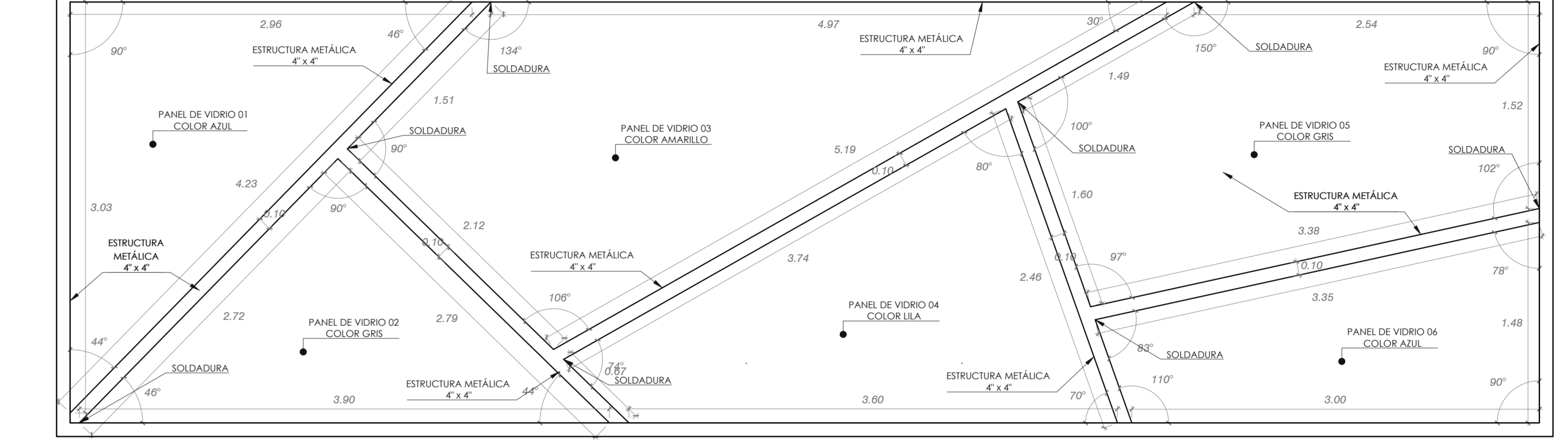
MURO CORTINA : ESTRUCTURA METALICA ESC: 1/25
