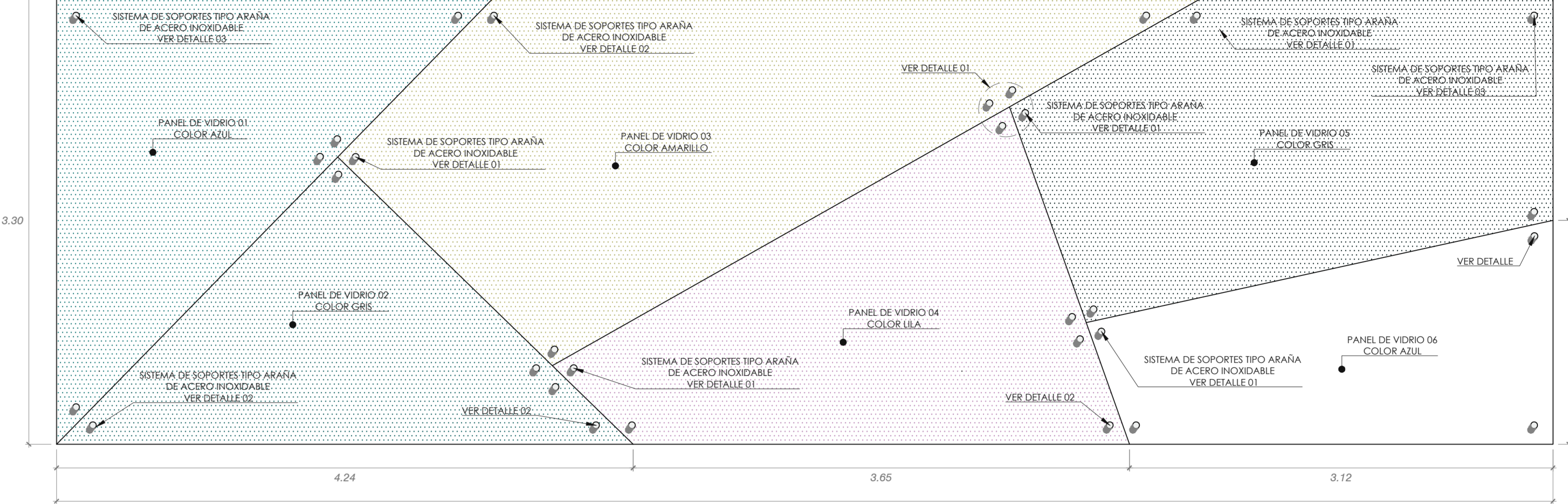
MURO CORTINA : ELEVACION ESC: 1/25
