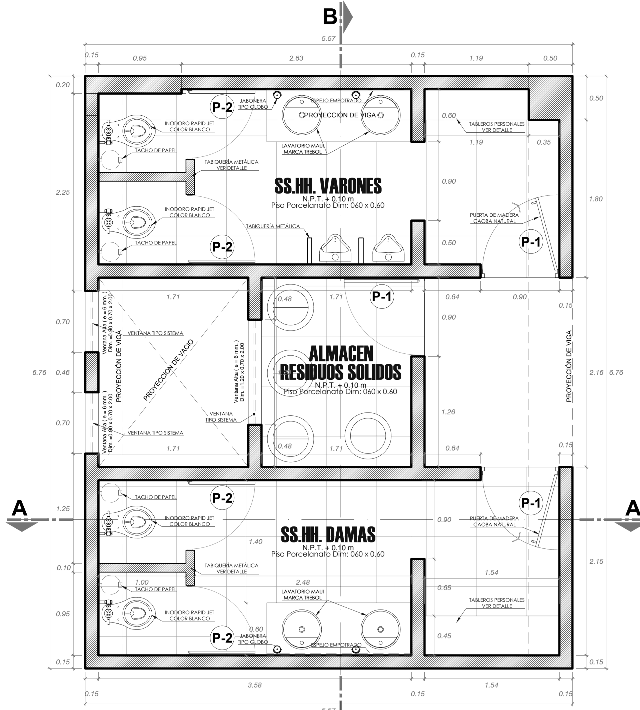
DETALLE DE BATERIA DE BAÑOS TIPO A ESC: 1/25
