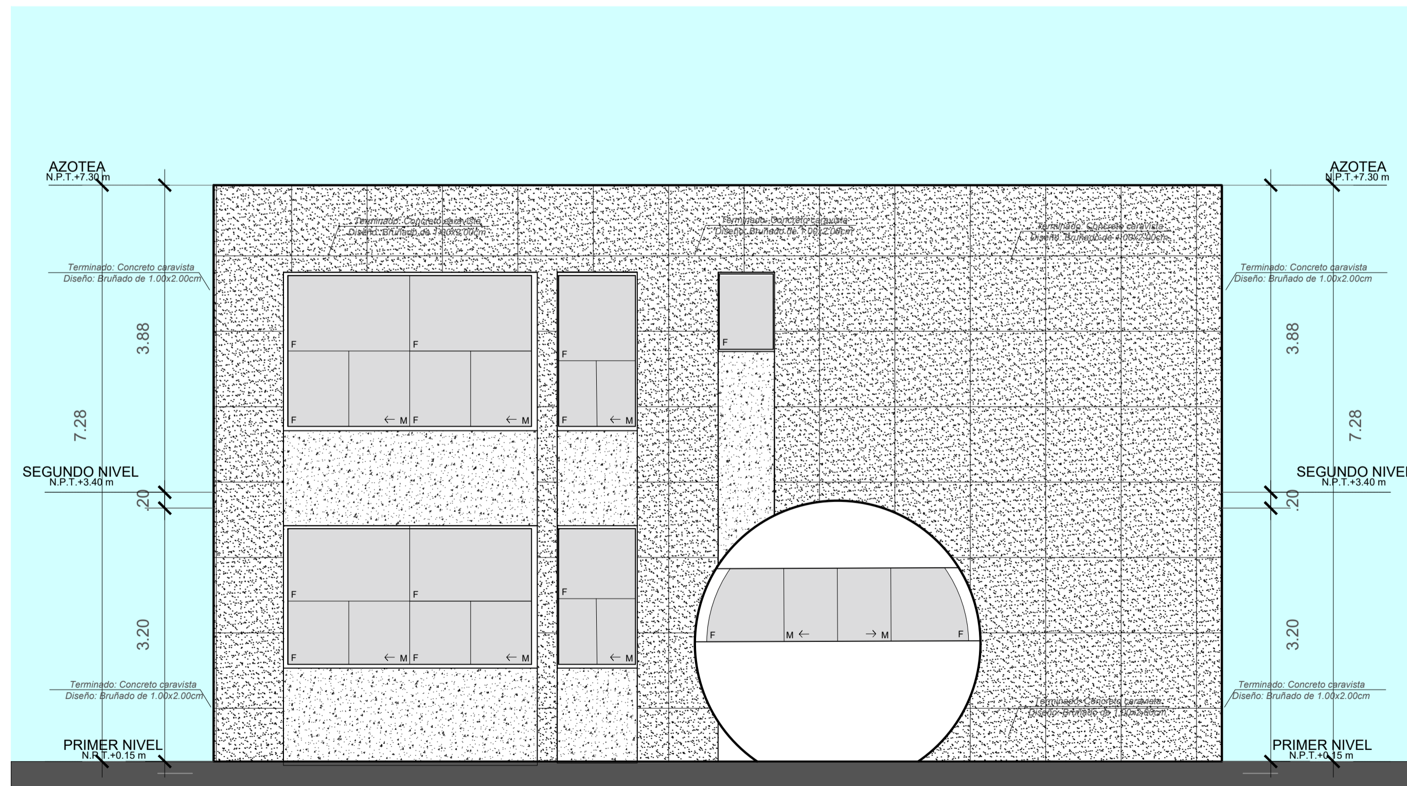
PROYECTO - BLOQUE B - ELEVACIÓN E2 ESC 1:50
