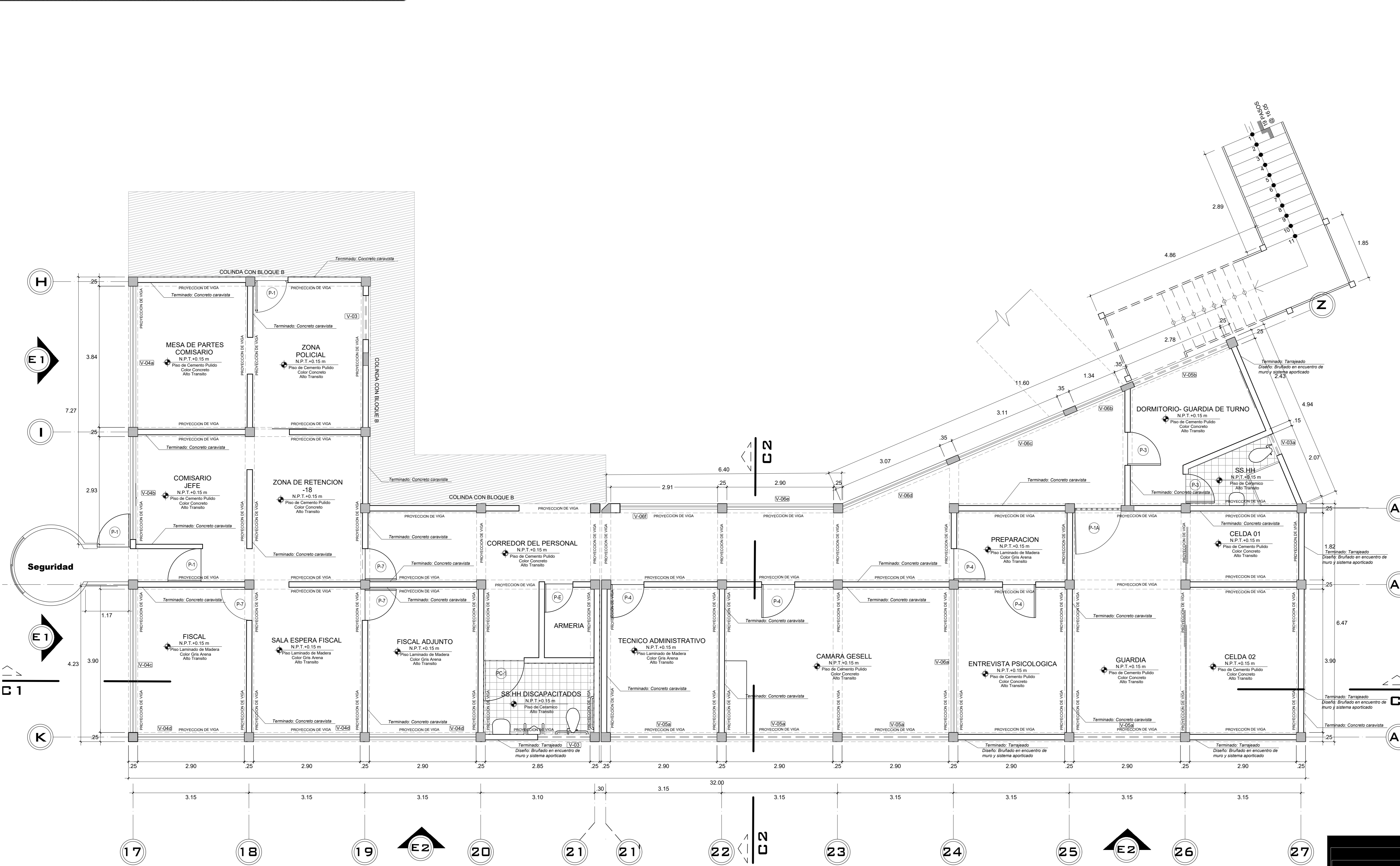
PRIMER PISO BLOQUE C PROYECTO ESC1:50
