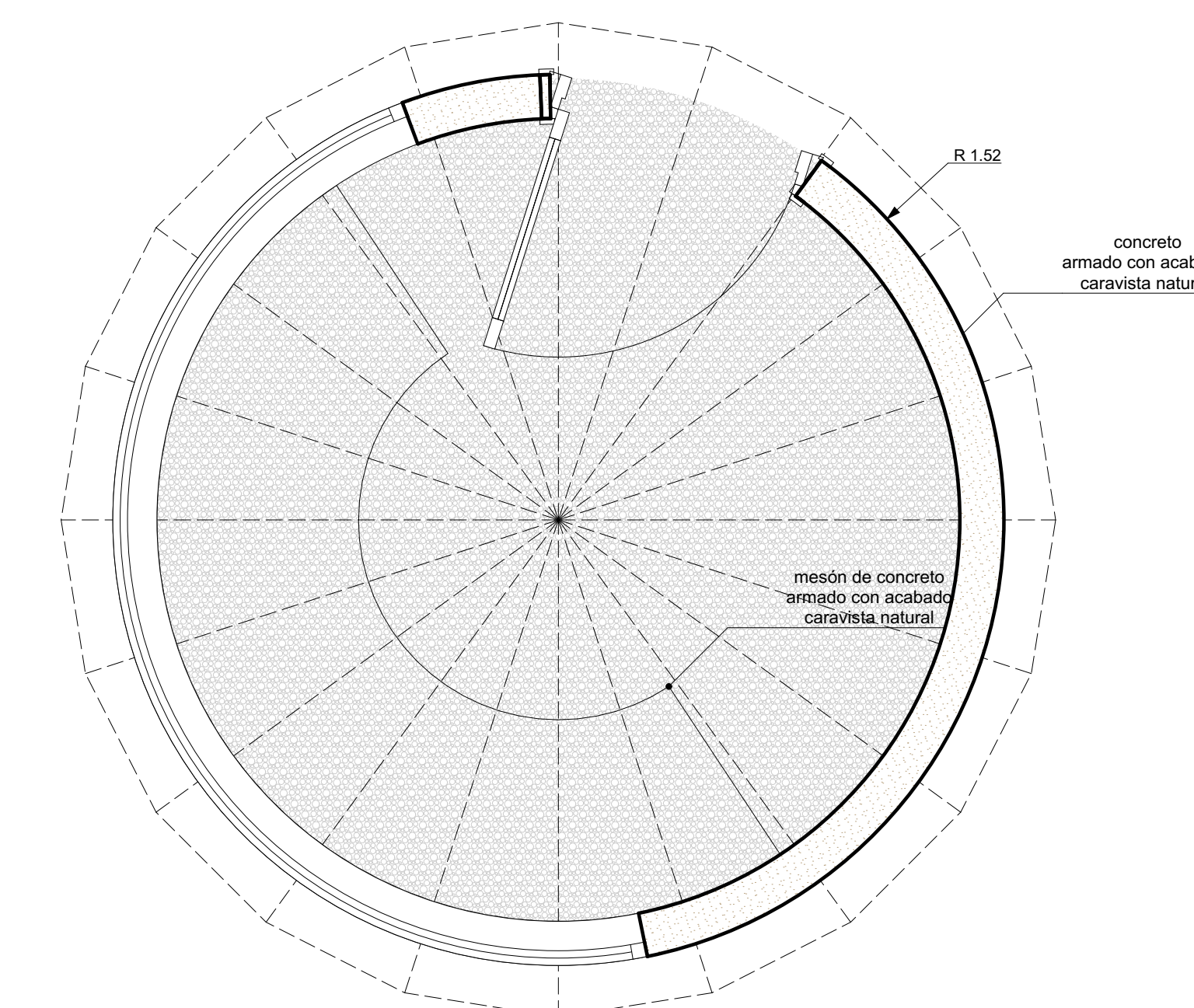
VISTA EN PLANTA
