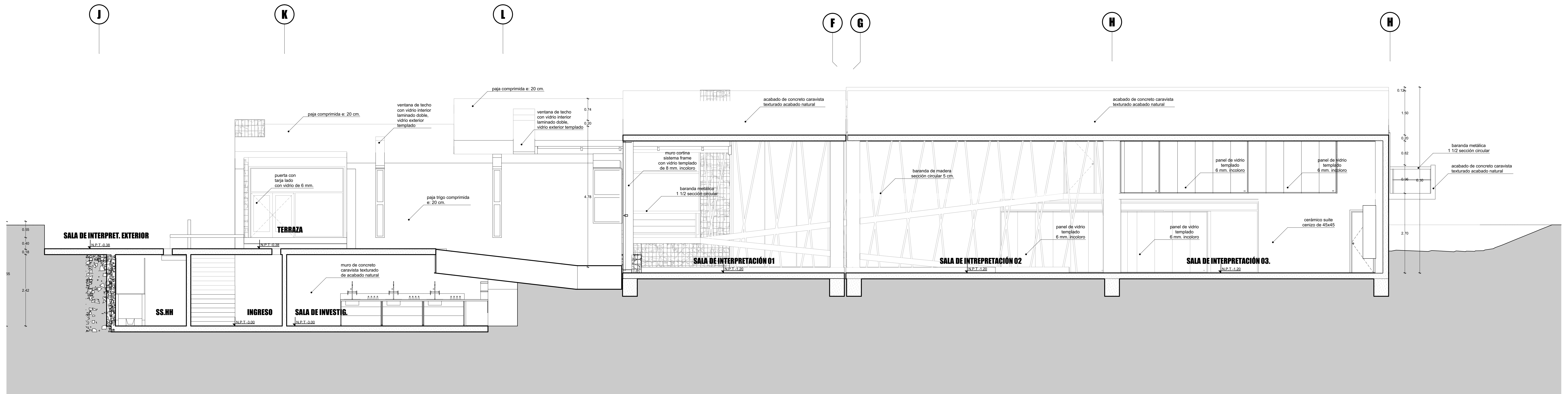
A CORTE A-A
