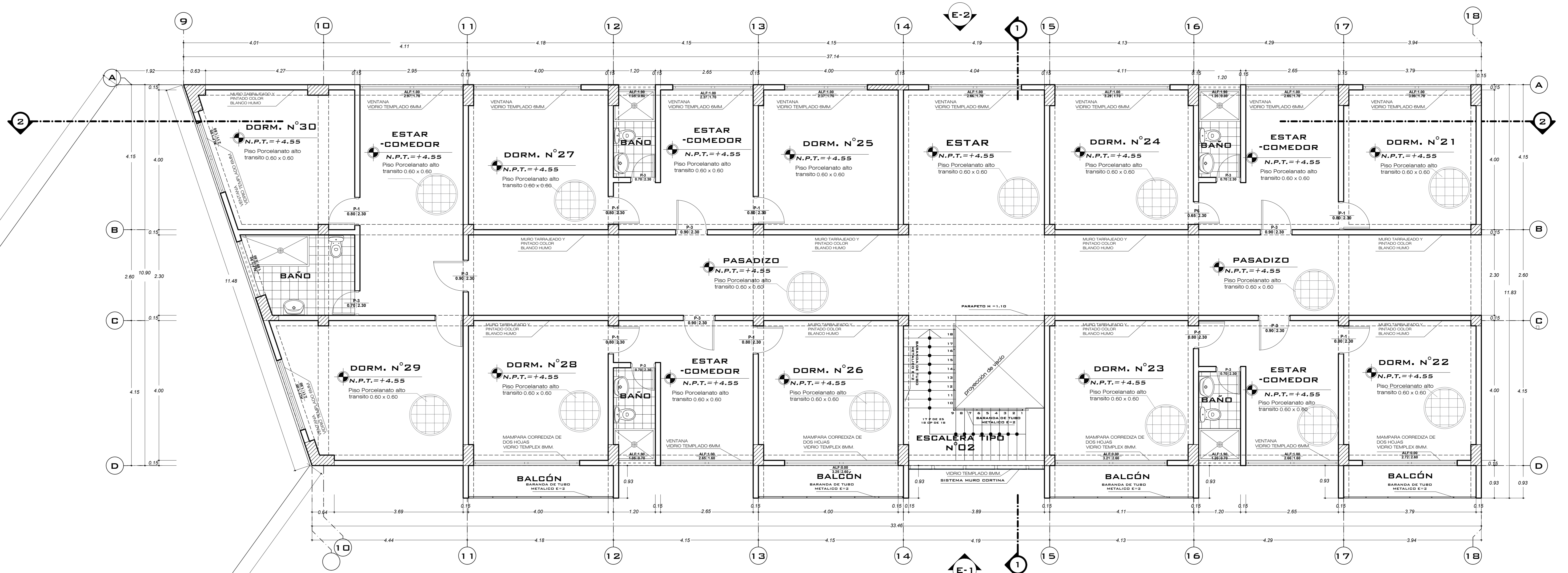
SEGUNDO NIVEL MODULO - E ESC: 1/50
