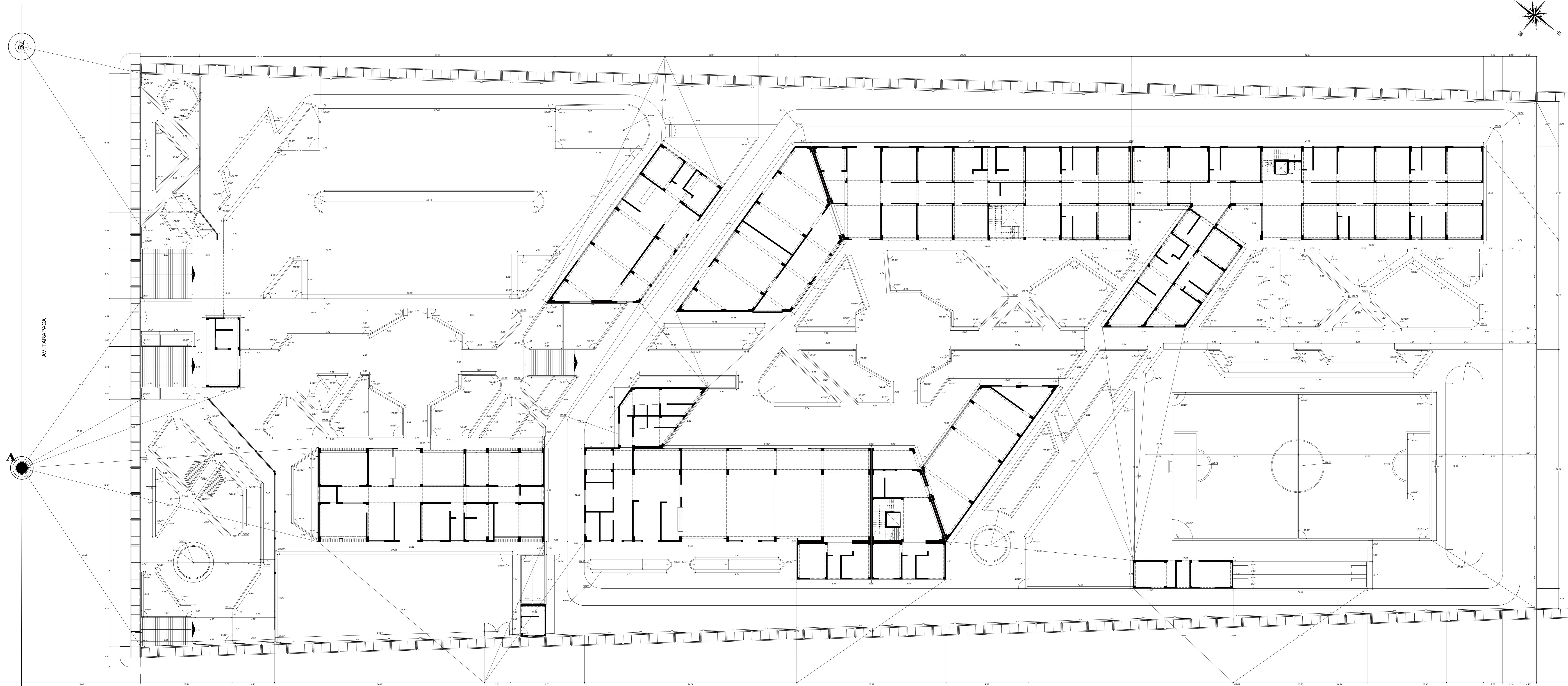
PLANIMETRIA GENERAL- TRAZADO ESC: 1/125
