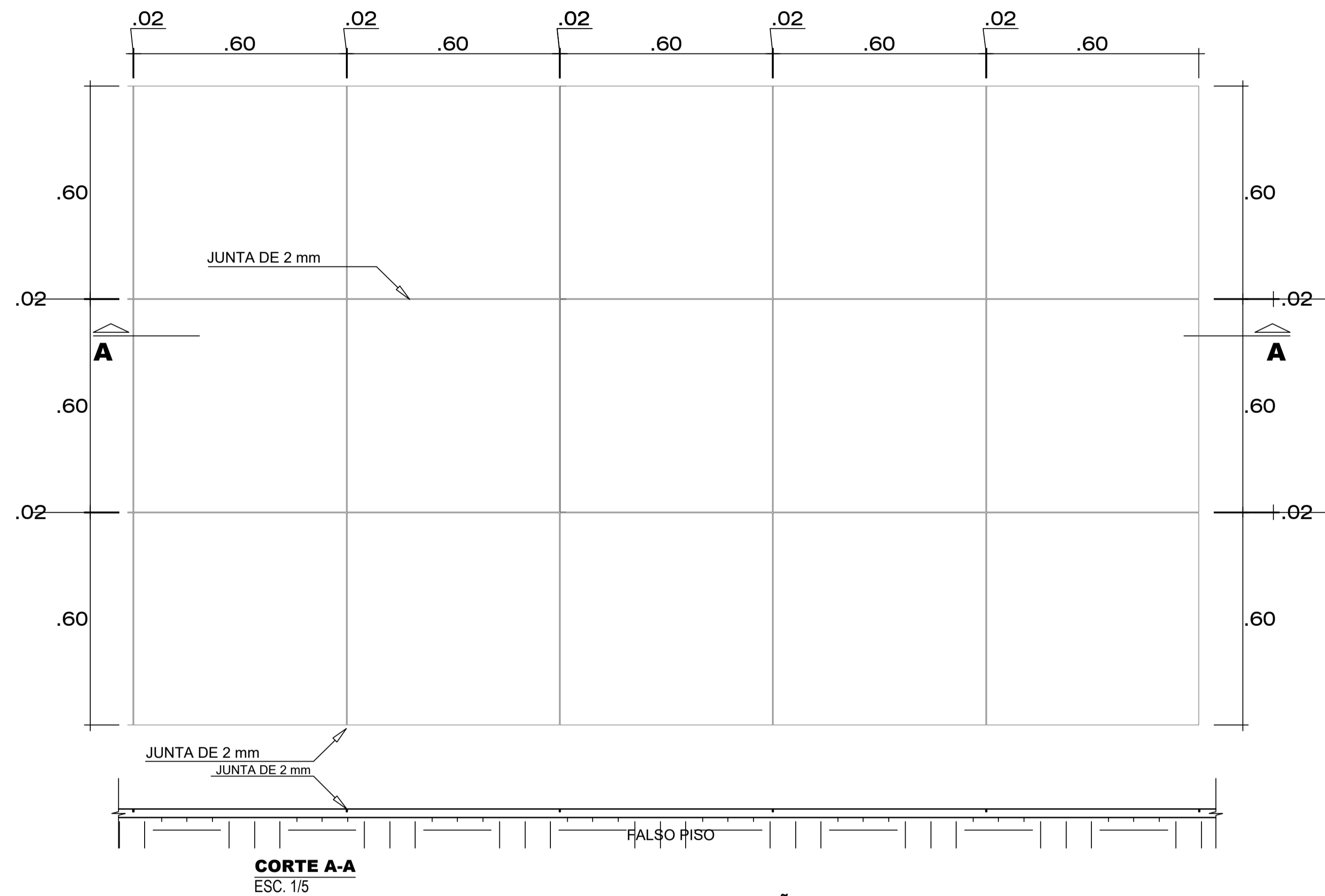
DETALLE DE PISO EN BAÑOS ESC. 1/10
