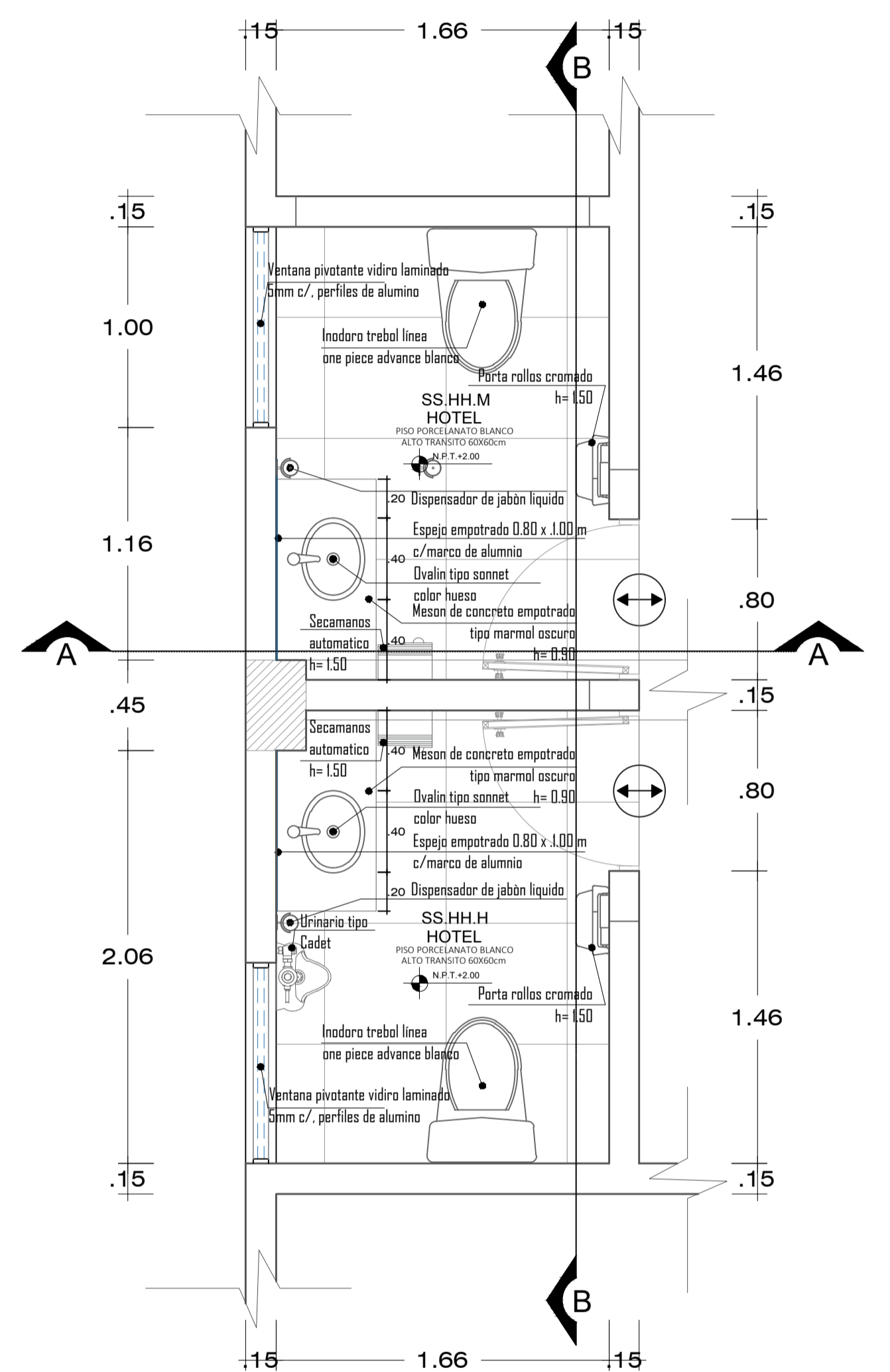
PLANO BAÑO HOTEL ESC. 1/25
