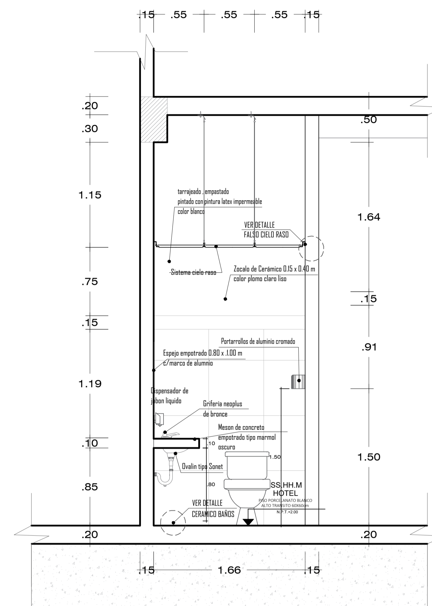
CORTE A-A DAMAS ESC. 1/25
