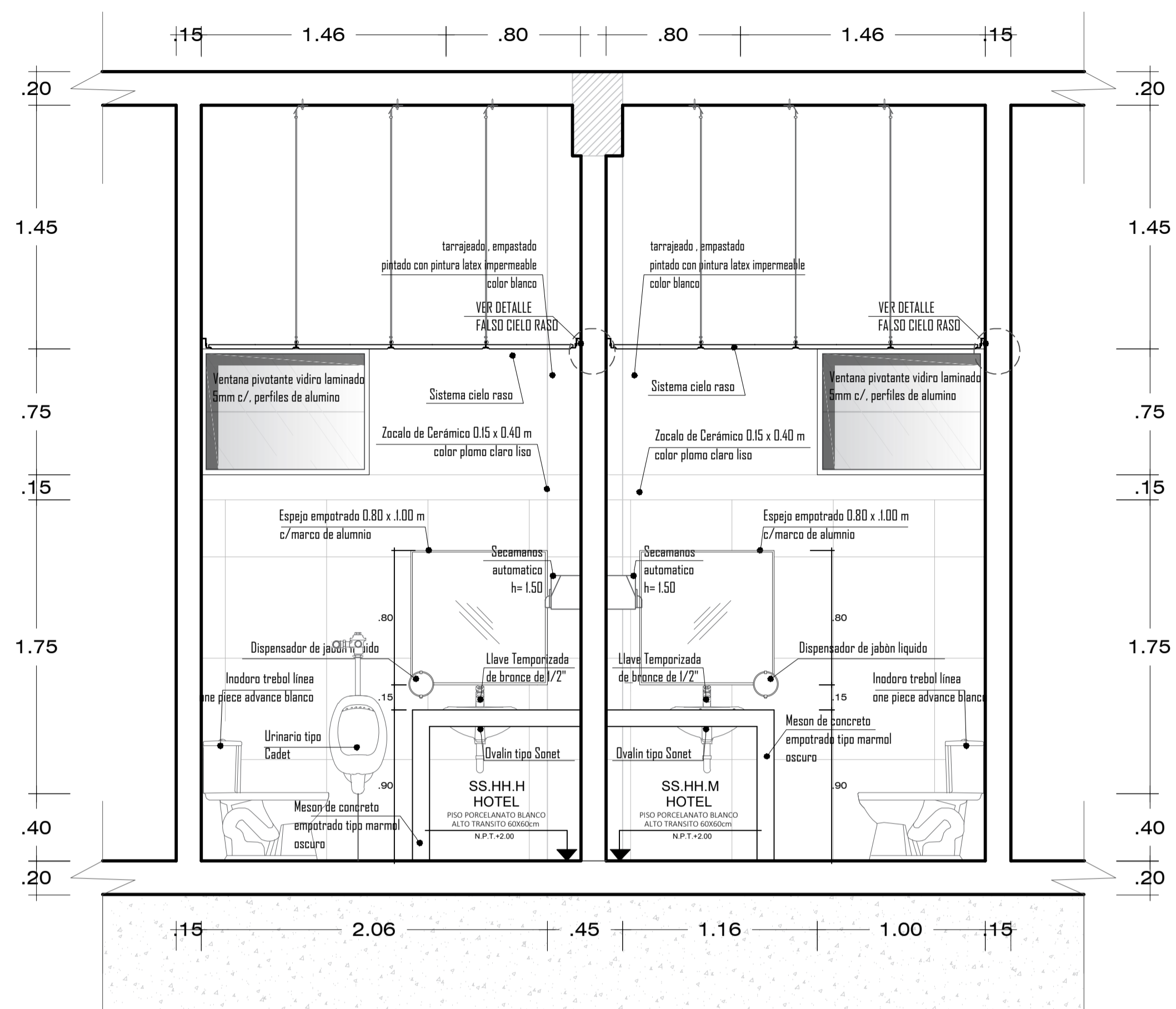
CORTE B-B VARON - DAMAS ESC. 1/25
