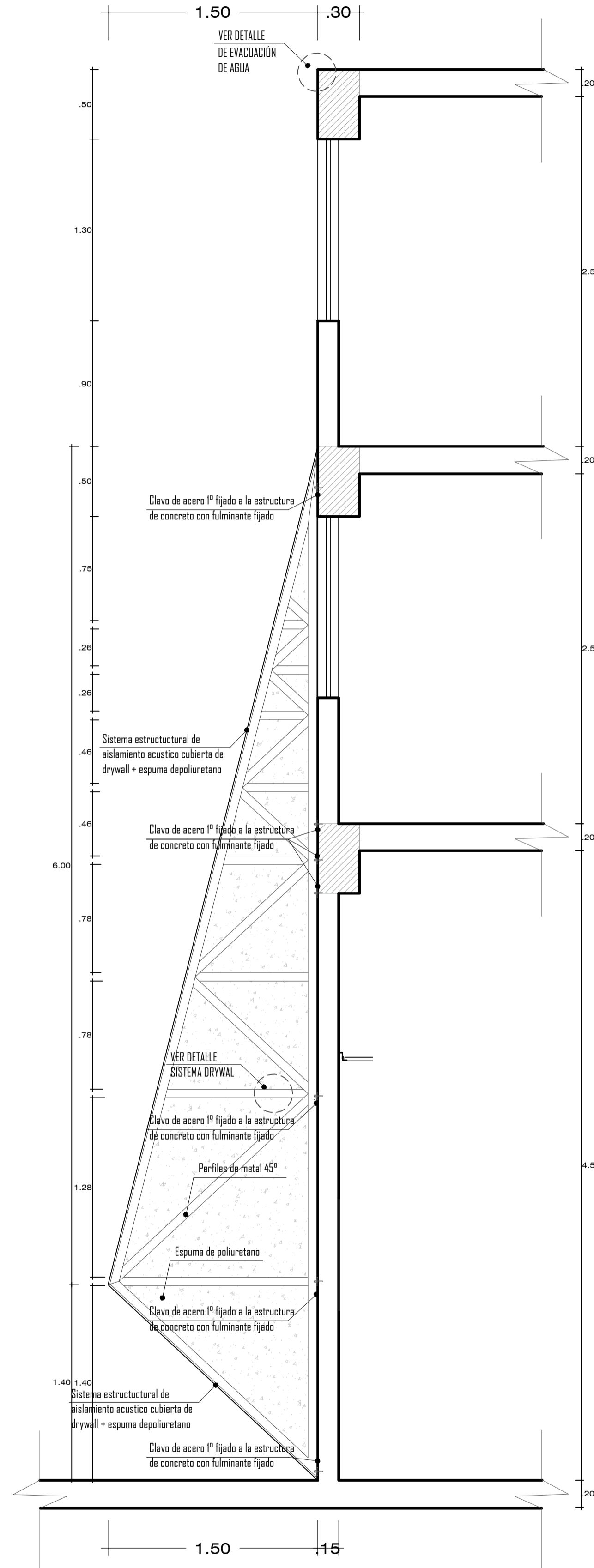
SECCION DE AISLAMIENTO ACUSTICO ESC. 1/25
