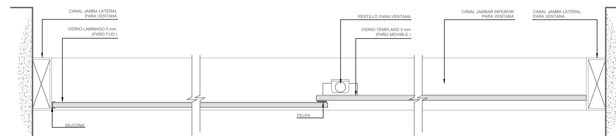
DETALLE VENTANA CORREDIZA ESC. 1/2.5
