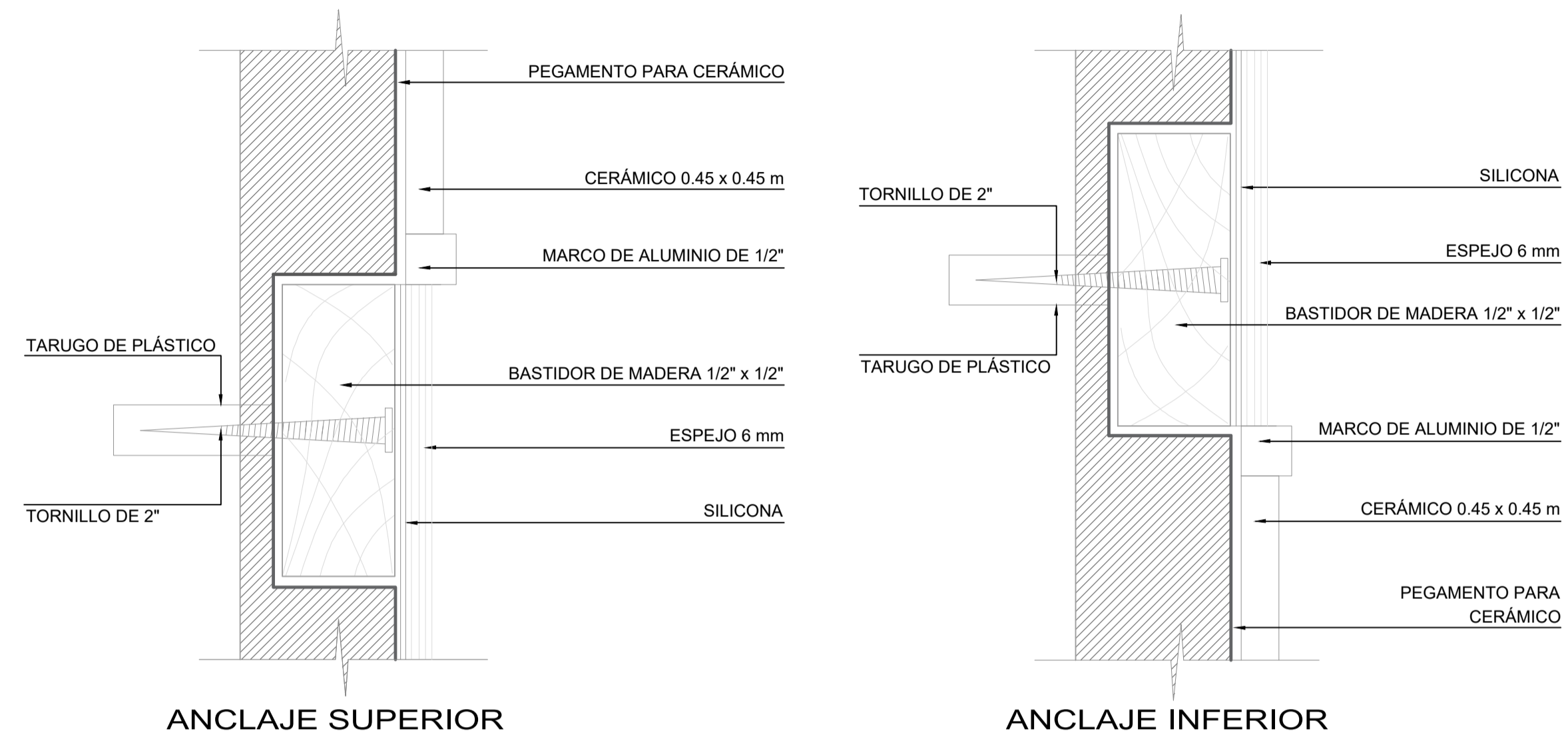
DETALLE DE FIJACION DE ESPEJO ESC. 1/5
