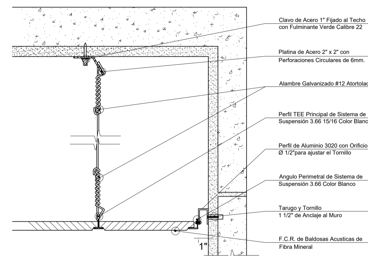
DETALLE - FALSO CIELO RASO ESC. 1/10
