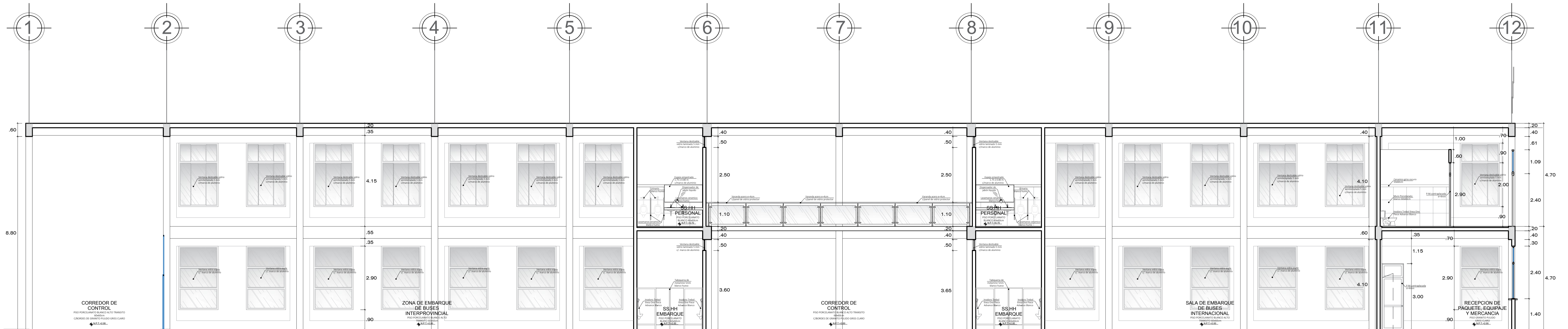
CORTE A-A
