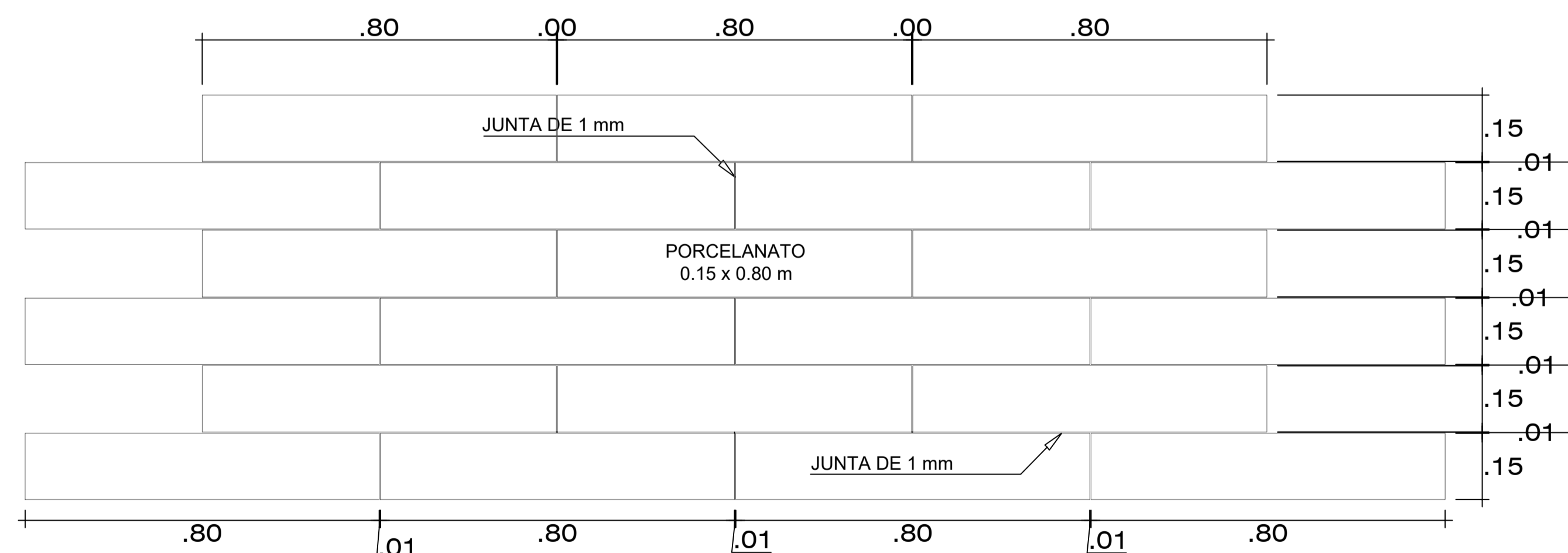
DETALLE DE PISO PORCELANATO MADERADO CLARO ESC. 1/10
