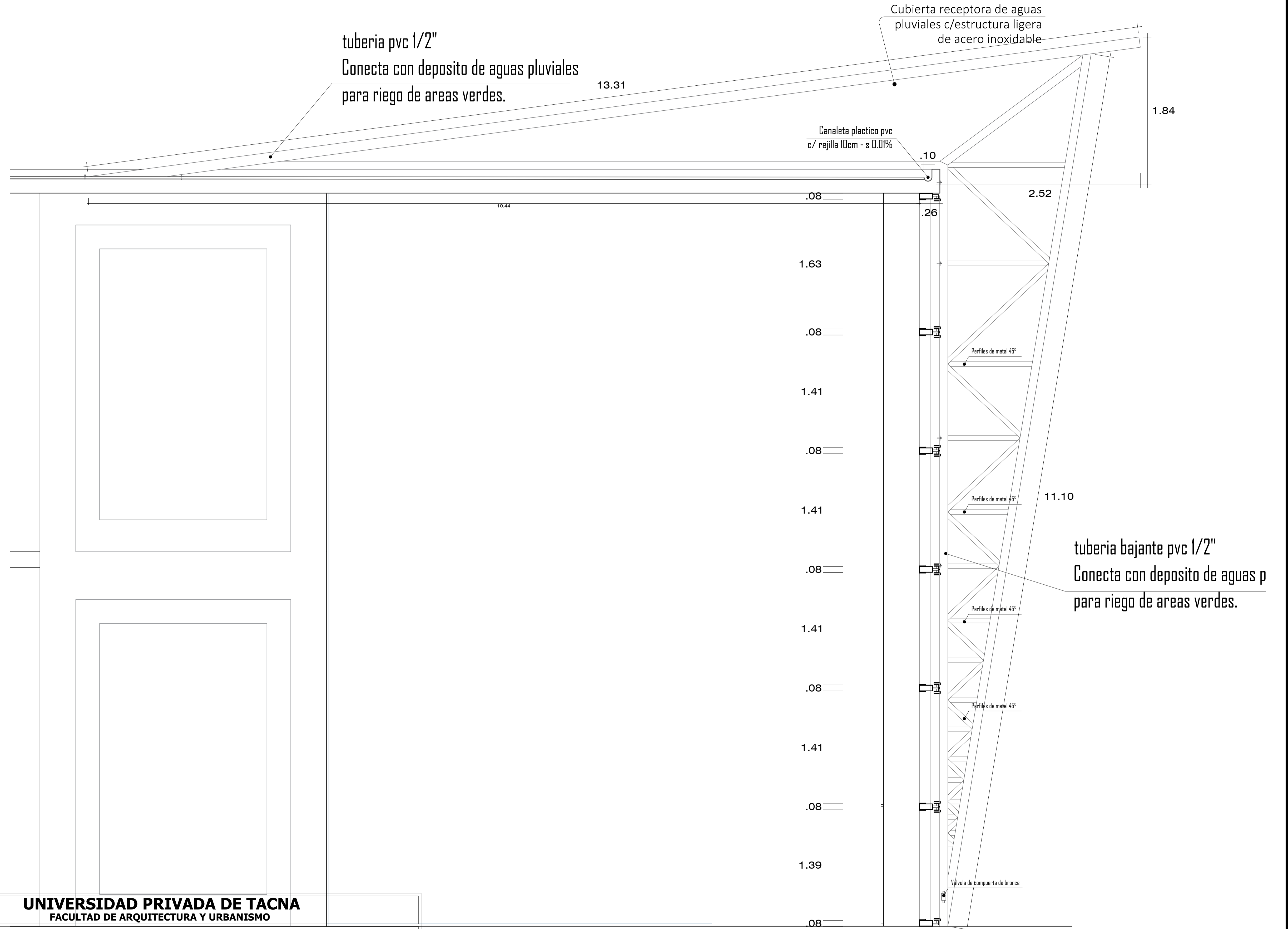
CORTE B-B ESC. 1/25
