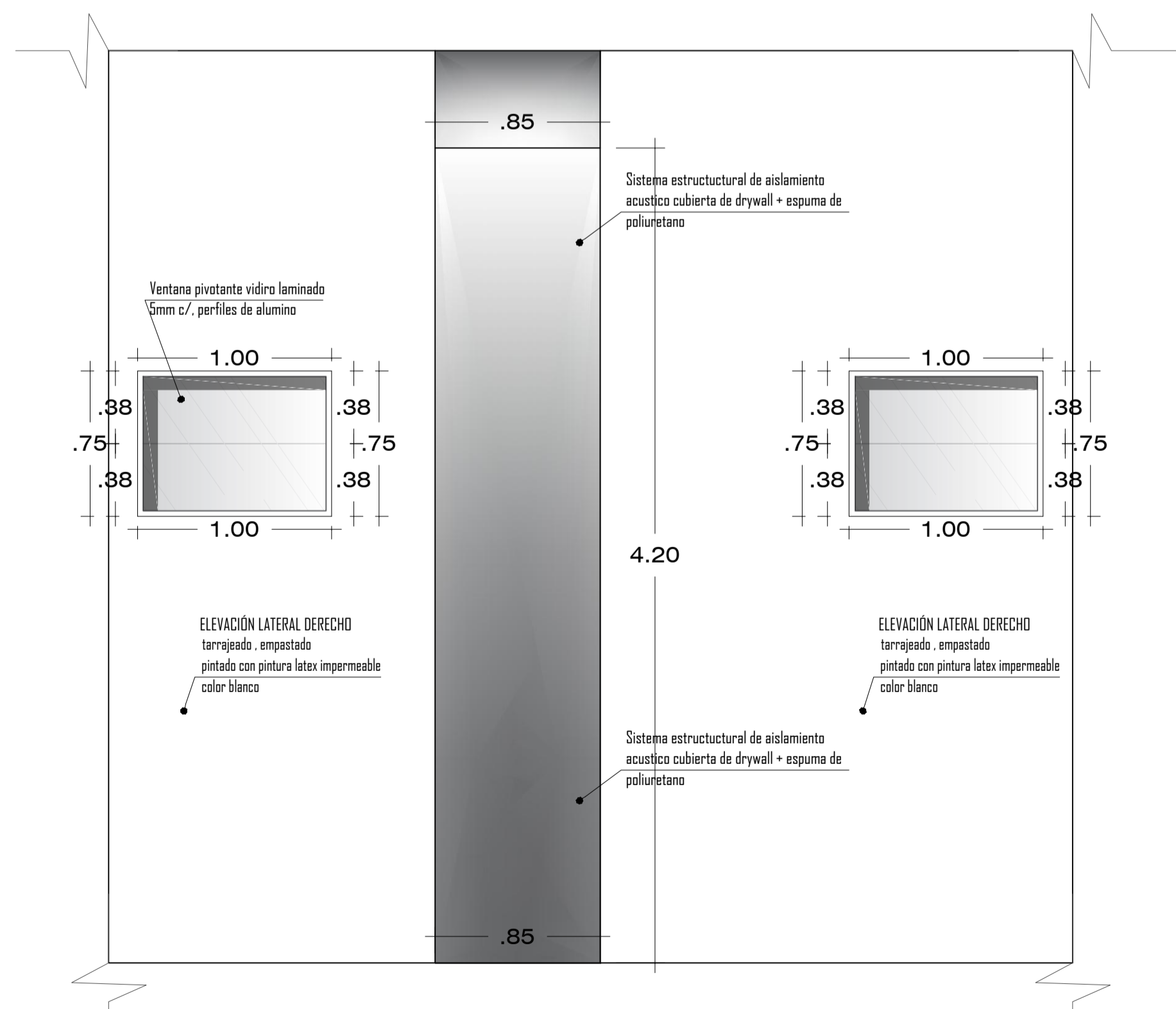
SECTOR - 1: PRIMER NIVEL PLANO DE DETALLES
