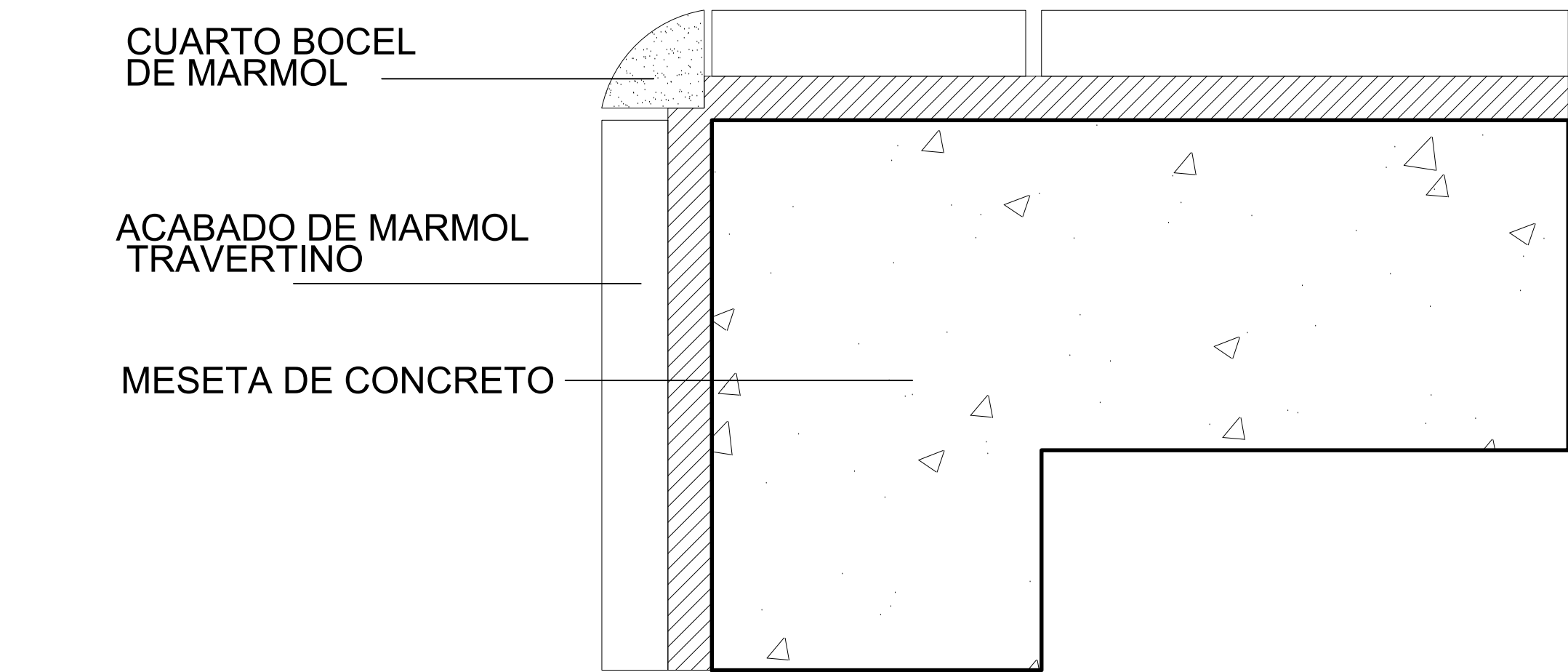
DETALLE X-BANCA DE CONCRETO ESCALA 1/5
