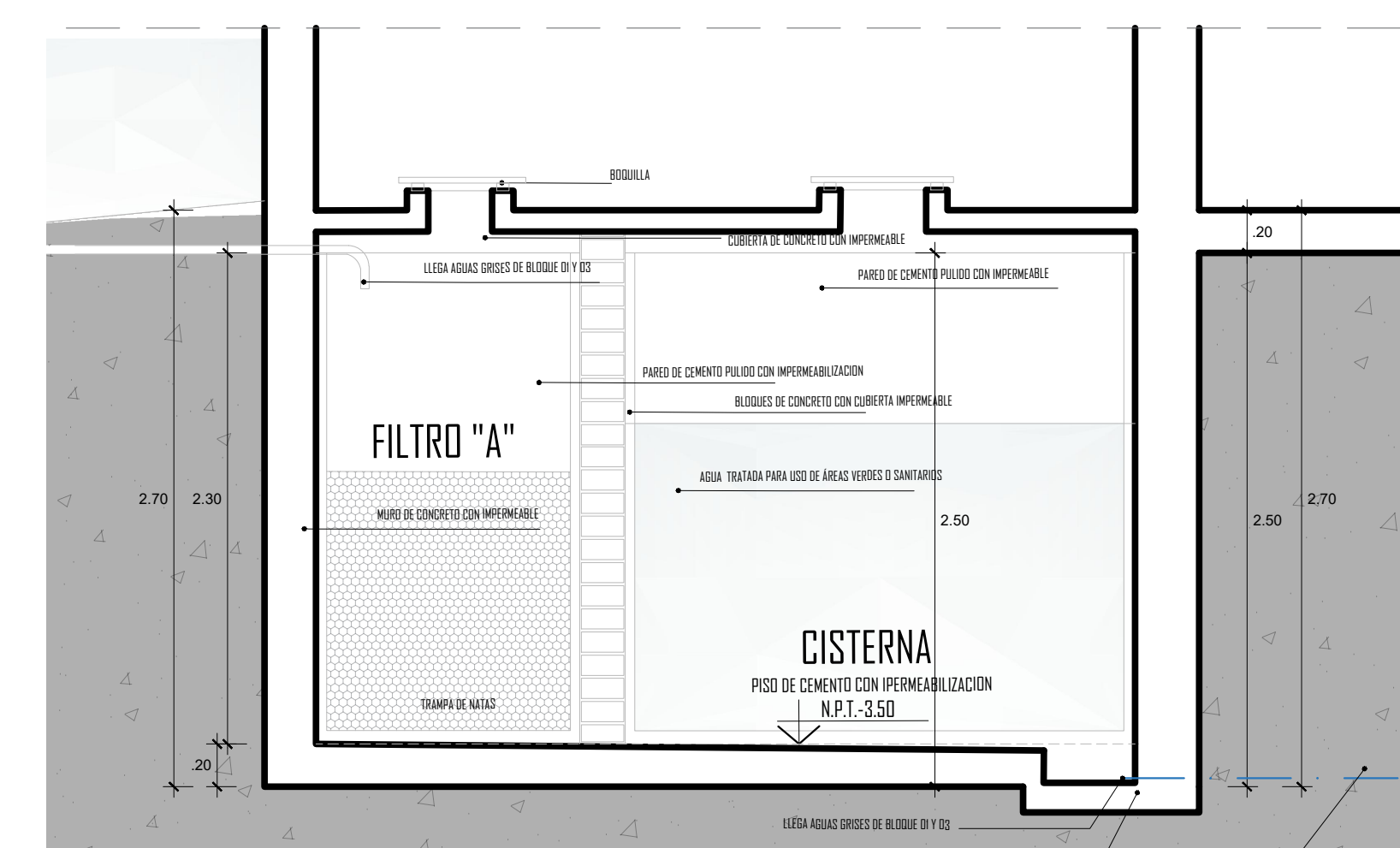
DETALLE 04 - CORTE A-A ESCALA 1/10
