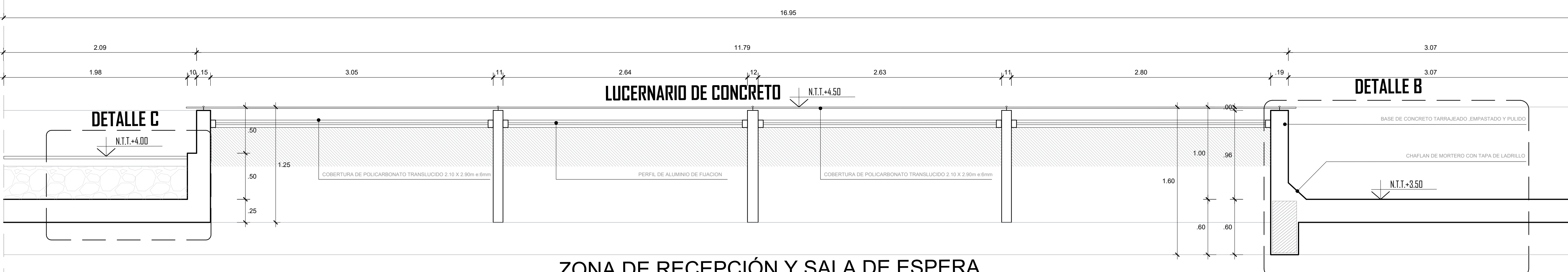
DETALLE 01 / CORTE A-A ESCALA 1/25 CENTRO DE INTERPRETACIÓN E INVESTIGACIÓN ARQUEOLÓGICA MICULLA
