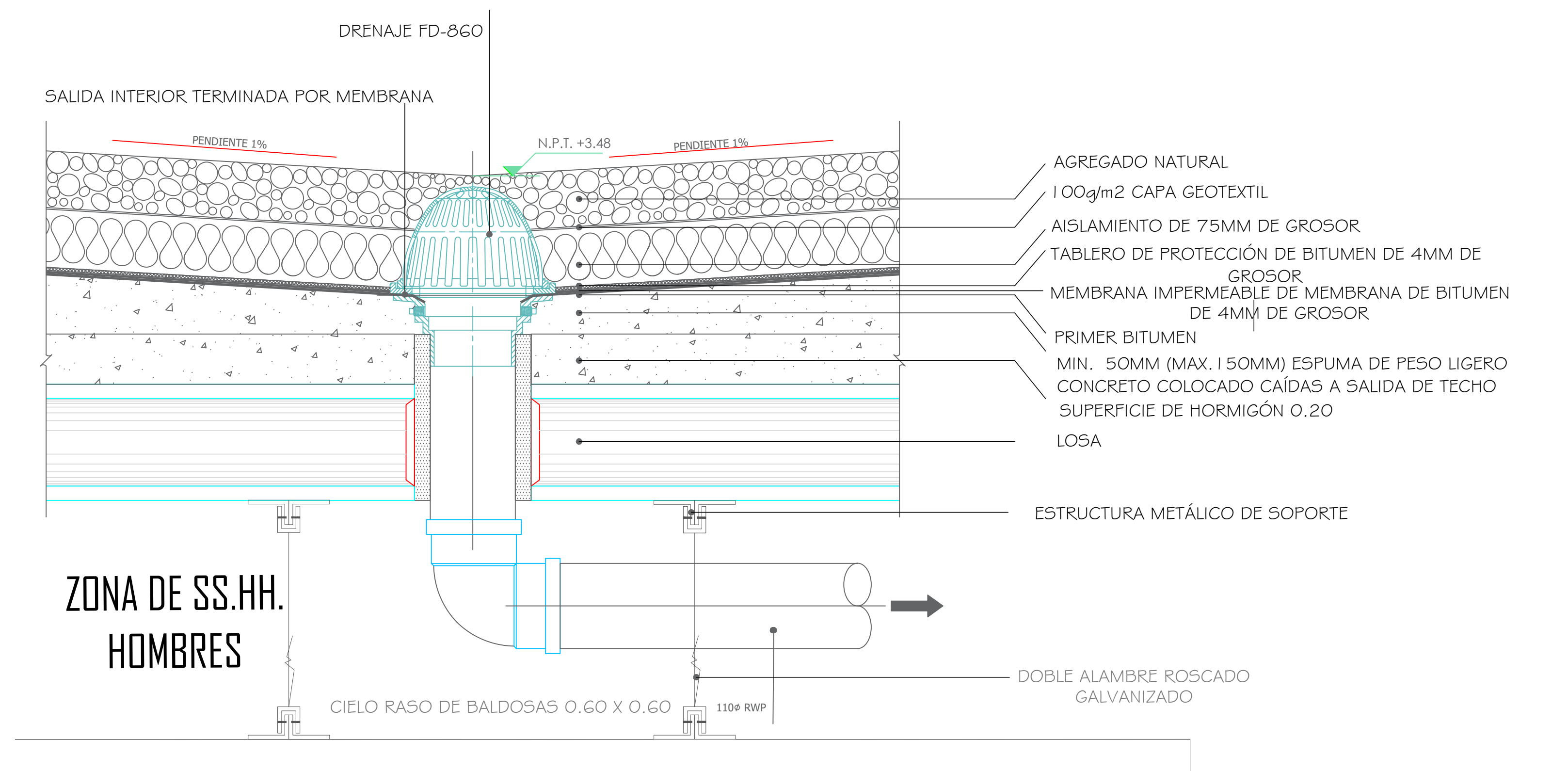
DETALLE A DE COLADERA DE AZOTEA ESCALA 1/3
