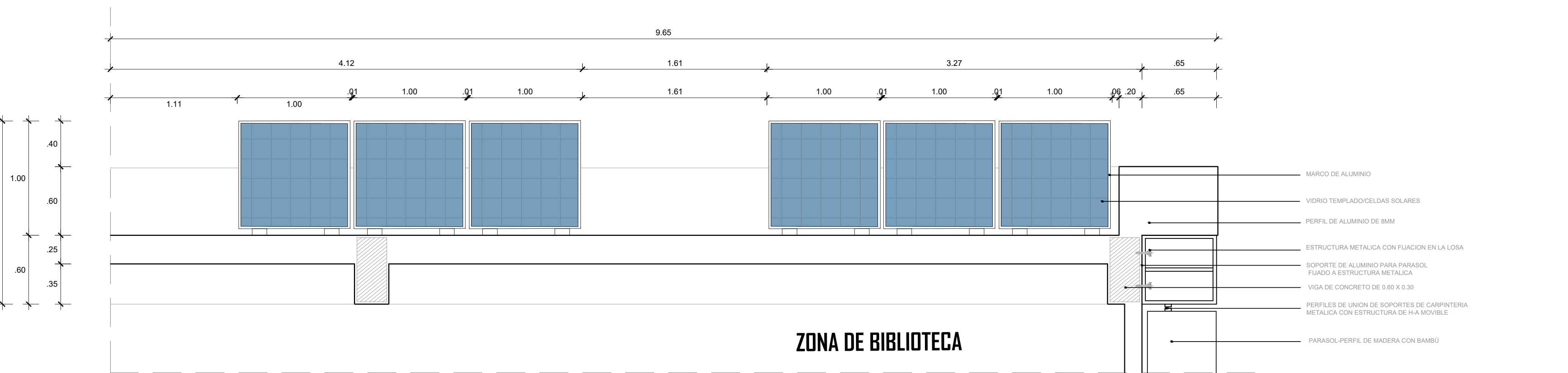
DETALLE 01 / CORTE B-B CENTRO DE INTERPRETACIÓN E INVESTIGACIÓN ARQUEOLÓGICA MICULLA ESCALA 1 / 25
