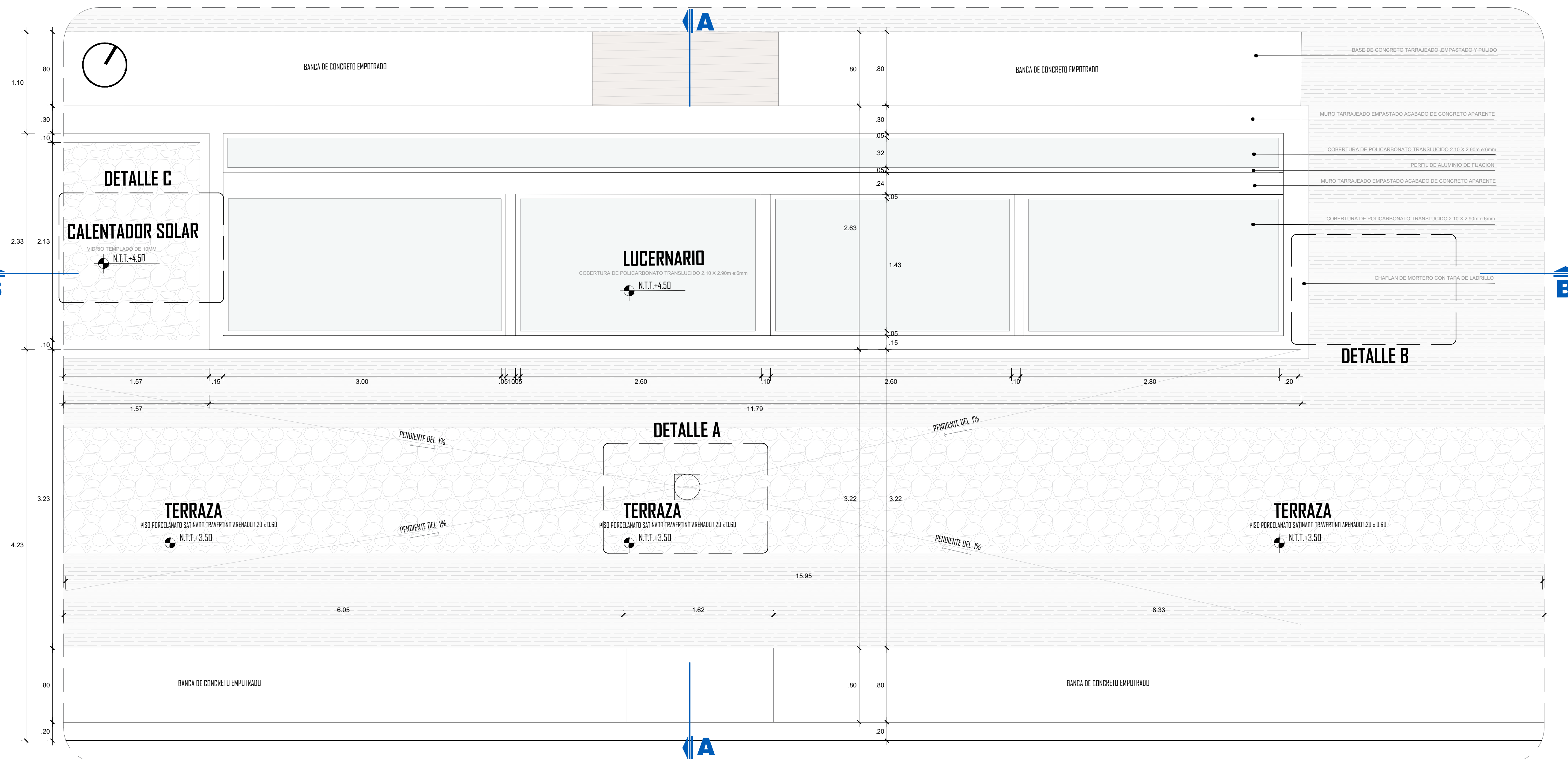
DETALLE 01-PLANTA ESCALA 1/25 CENTRO DE INTERPRETACIÓN E INVESTIGACIÓN ARQUEOLÓGICA MICULLA
