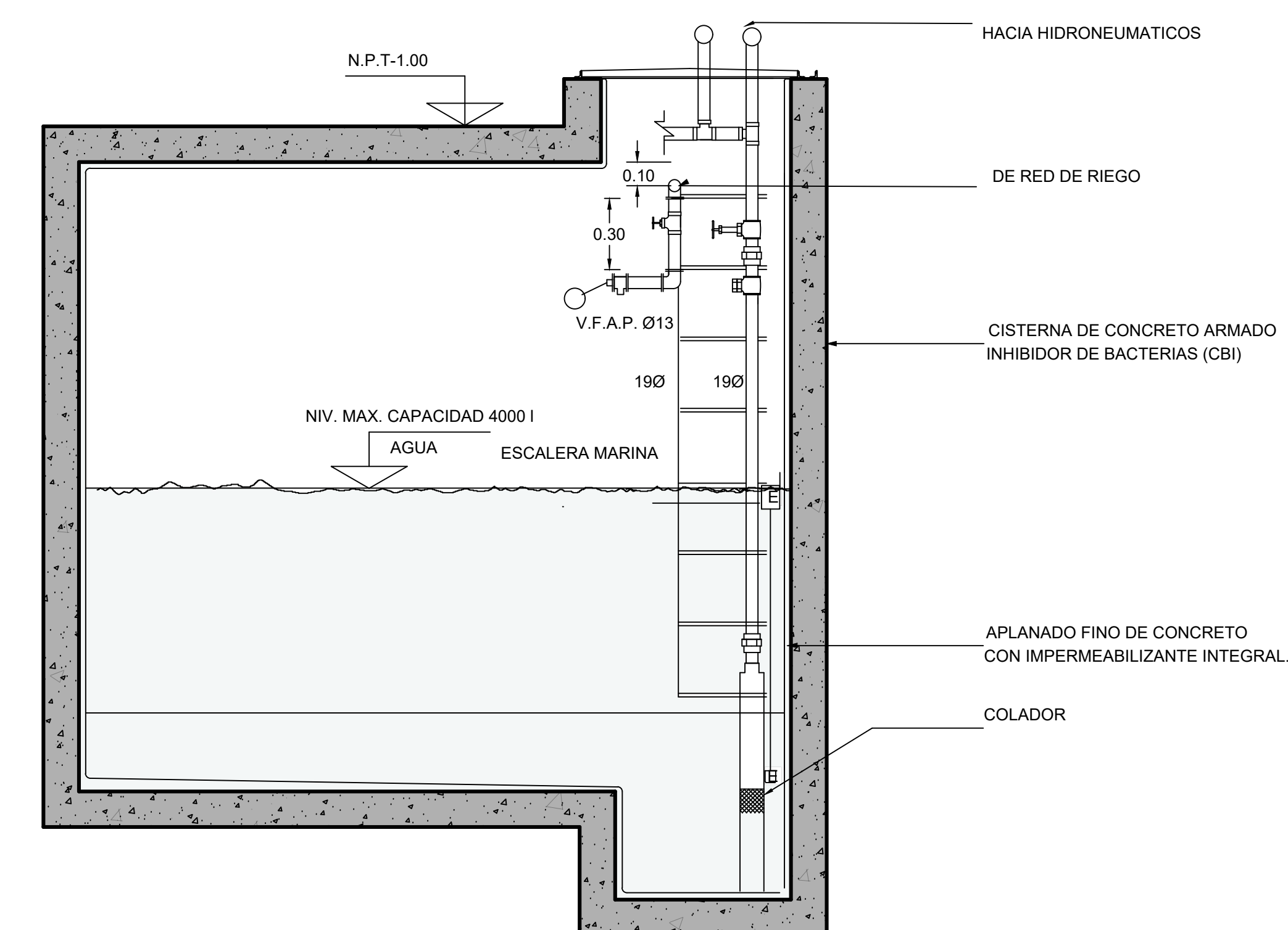
DETALLE A-CISTERNA DE AGUAS GRISES ESCALA 1/10
