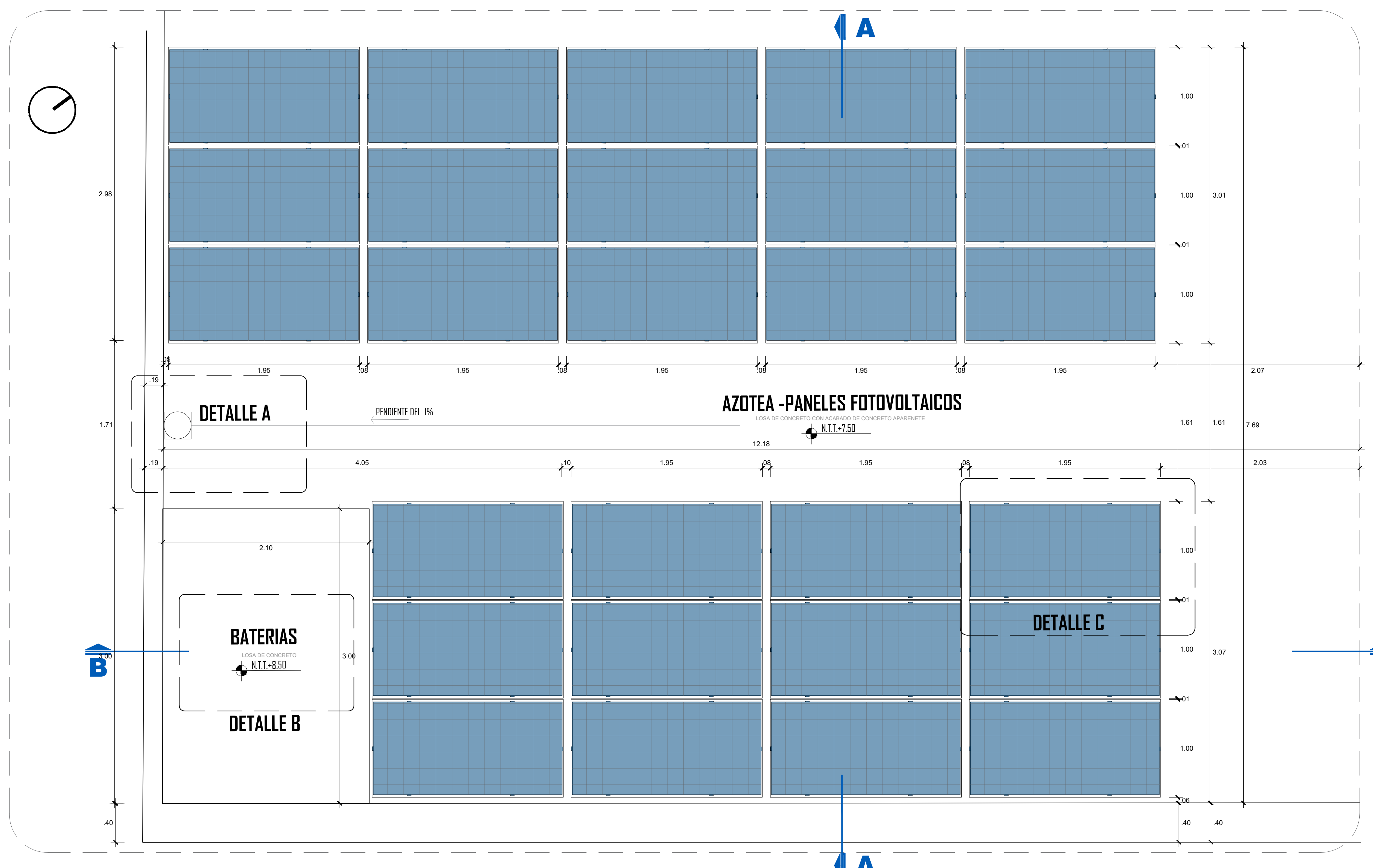
DETALLE 01-PLANTA PANELES SOLARES CENTRO DE INTERPRETACIÓN E INVESTIGACIÓN ARQUEOLÓGICA MICULLA ESCALA 1 / 25
