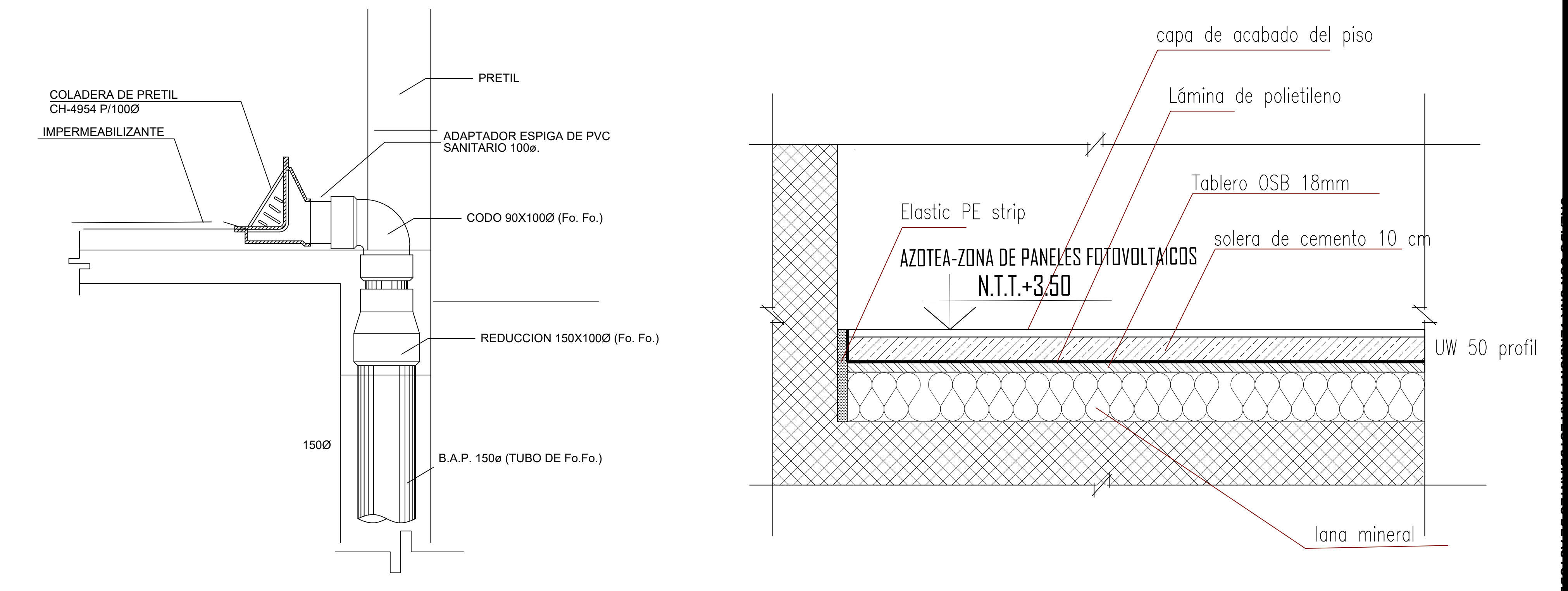
DETALLE B DE COLADERO Y PISO IMPERMEABILIZABLE ESCALA 1 / 5
