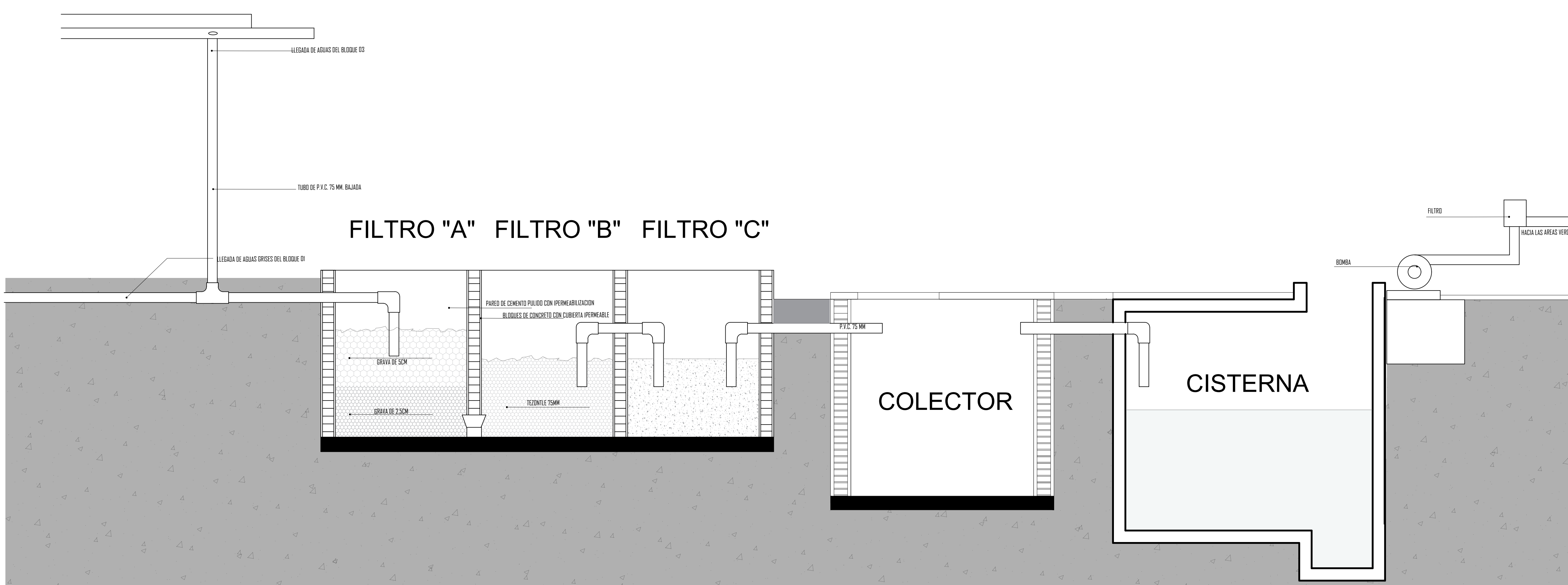
ESQUEMA FUNCIONAL DE AGUAS GRISES CENTRO DE INTERPRETACION ARQUEOLÓGICO MICULLA ESCALA 1/25
