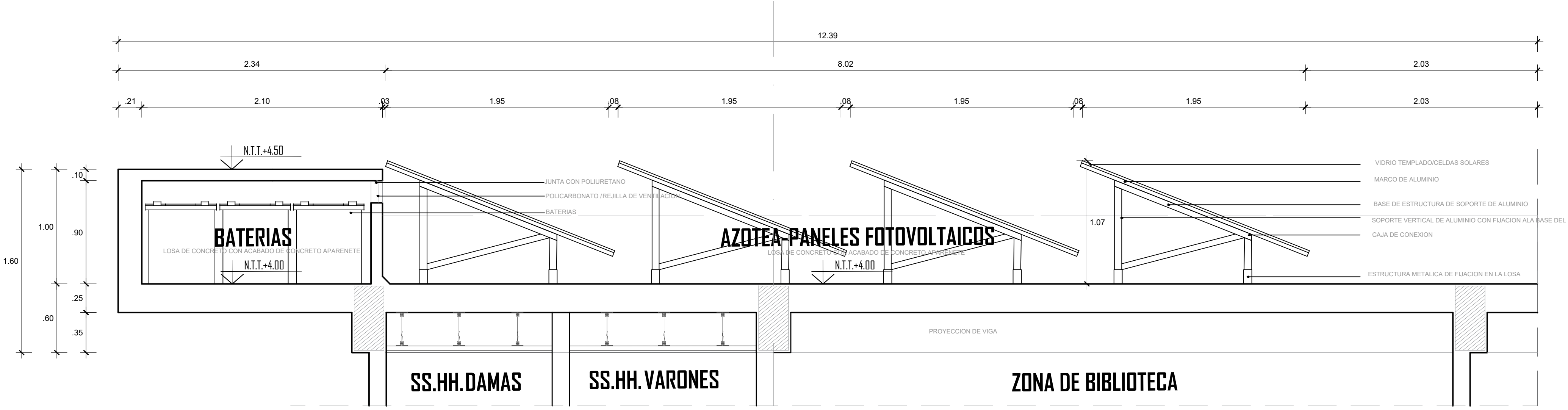
DETALLE 01 / CORTE A-A CENTRO DE INTERPRETACIÓN E INVESTIGACIÓN ARQUEOLÓGICA MICULLA ESCALA 1 / 25
