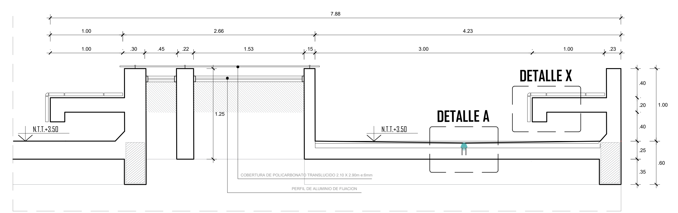
DETALLE 01 / CORTE B-B ESCALA 1/25 CENTRO DE INTERPRETACIÓN E INVESTIGACIÓN ARQUEOLÓGICA MICULLA
