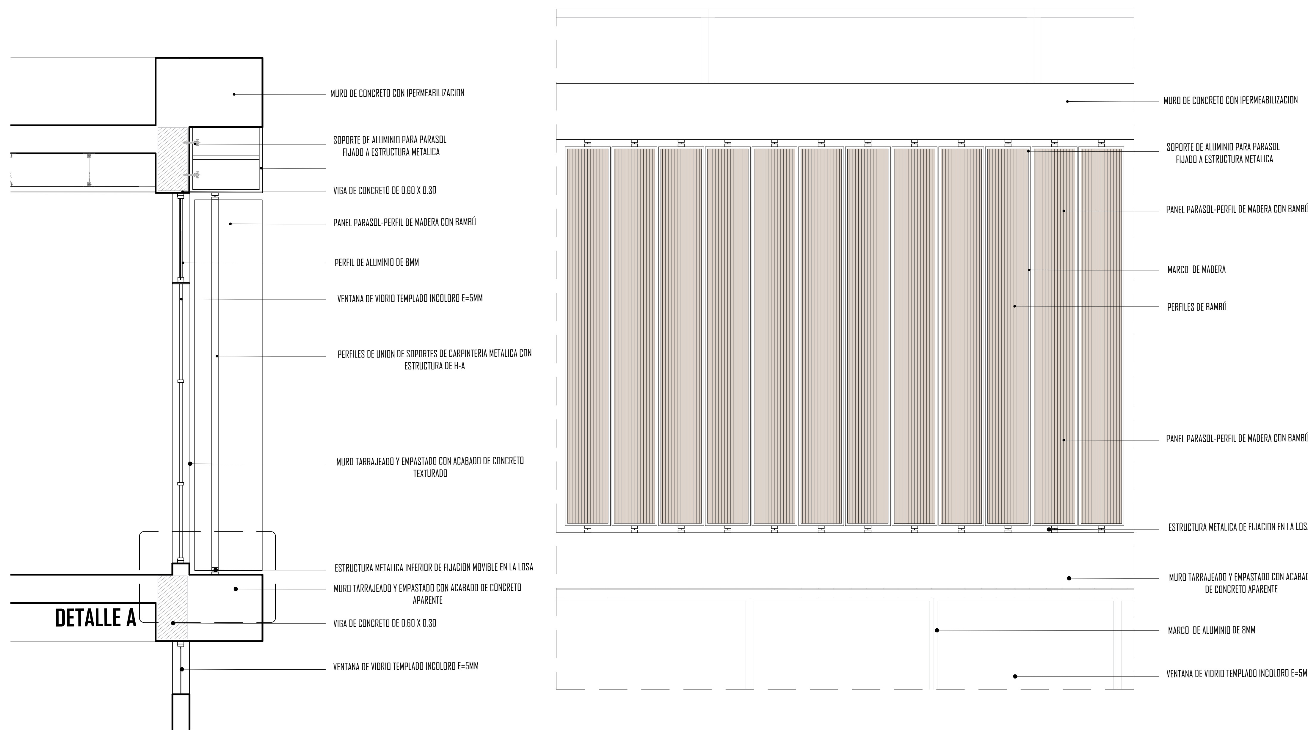
DETALLE 03 / ELEVACIÓN 01 ESCALA 1/25 CENTRO DE INTERPRETACIÓN E INVESTIGACIÓN ARQUEOLÓGICA MICULLA
