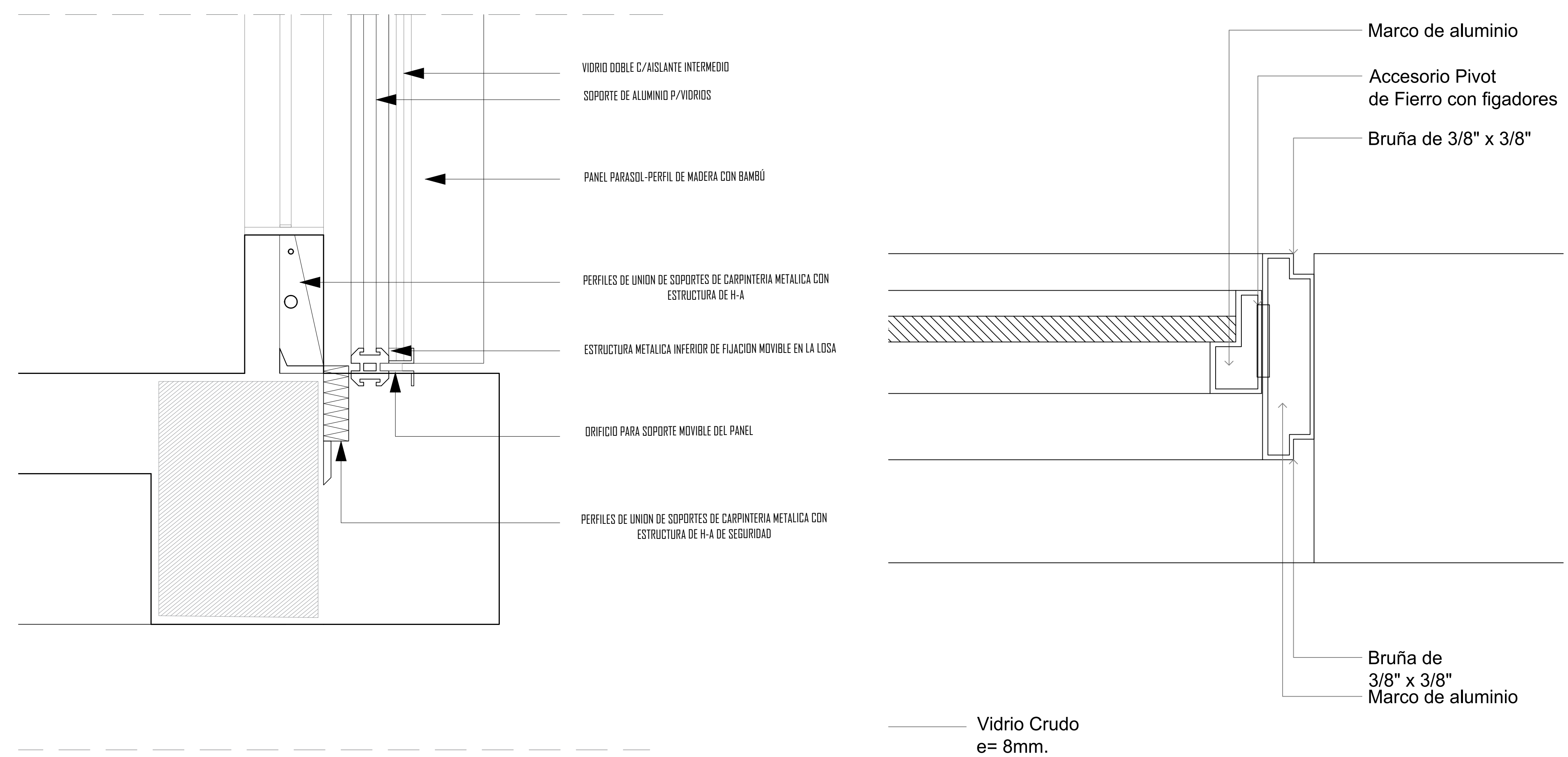
DETALLE A -PARASOL ESCALA 1/10
