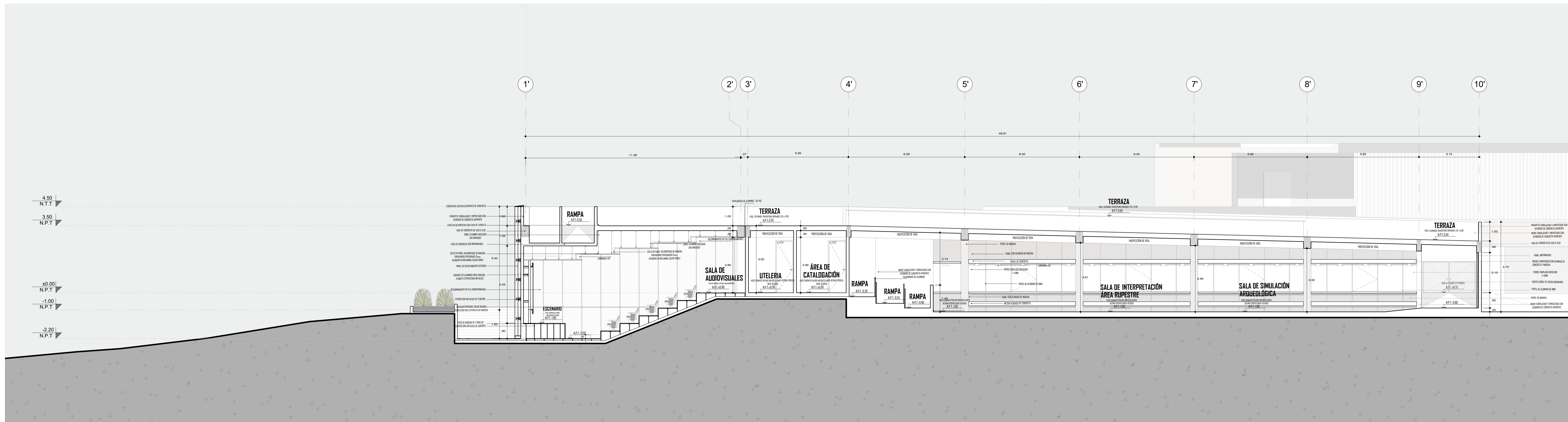
BLOQUE 02-CORTE A-A ESCALA 1/75 CENTRO DE INTERPRETACIÓN E INVESTIGACIÓN ARQUEOLÓGICA MICULLA
