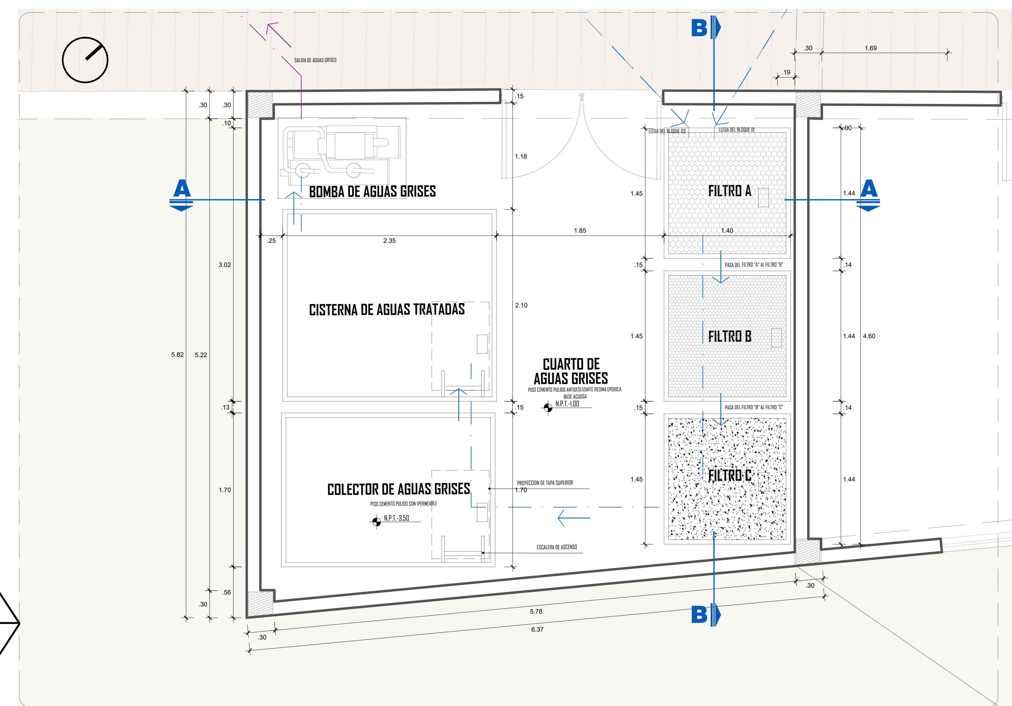
DETALLE 04-PLANTA DE AGUAS GRISES CENTRO DE INTERPRETACION E INVESTIGACION ARQUEOLÓGICA MICULLA ESCALA 1/25
