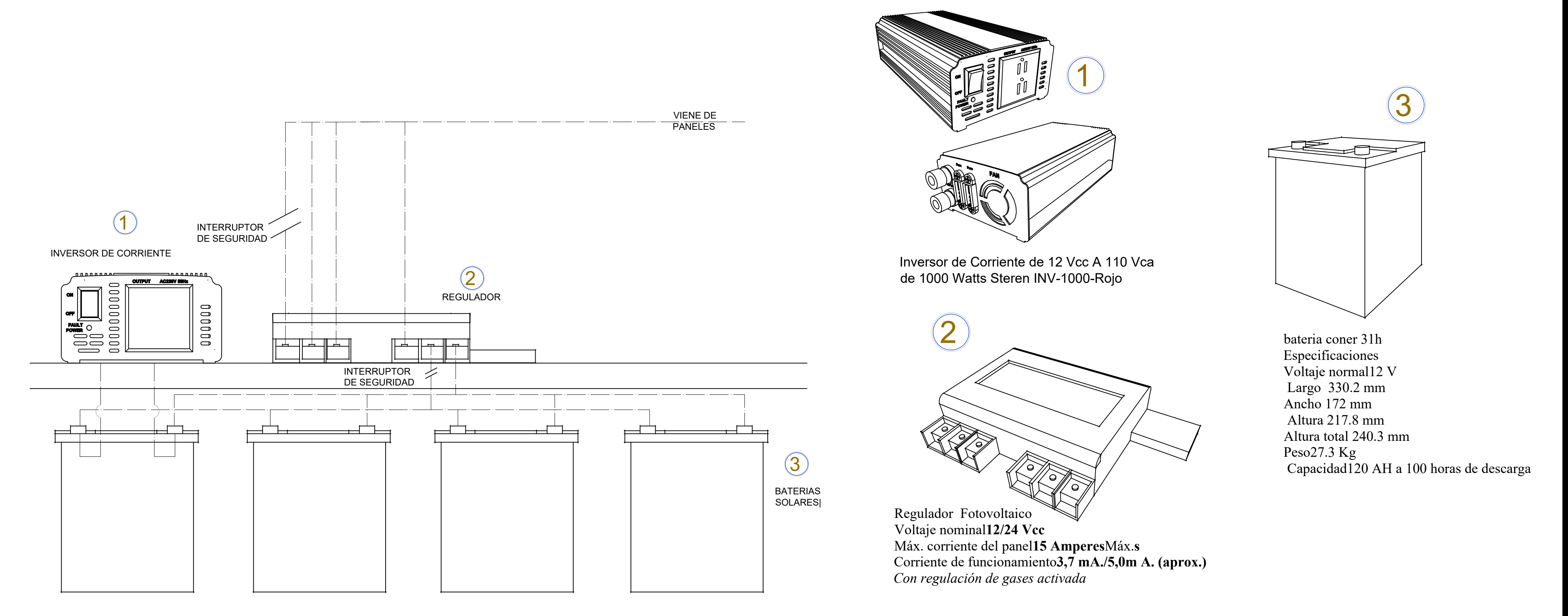
DETALLE C -BATERIAS ESCALA 1 / 5
