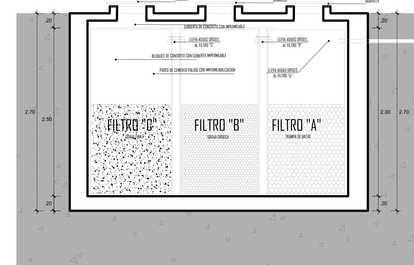
DETALLE 04 - CORTE B-B ESCALA 1/10
