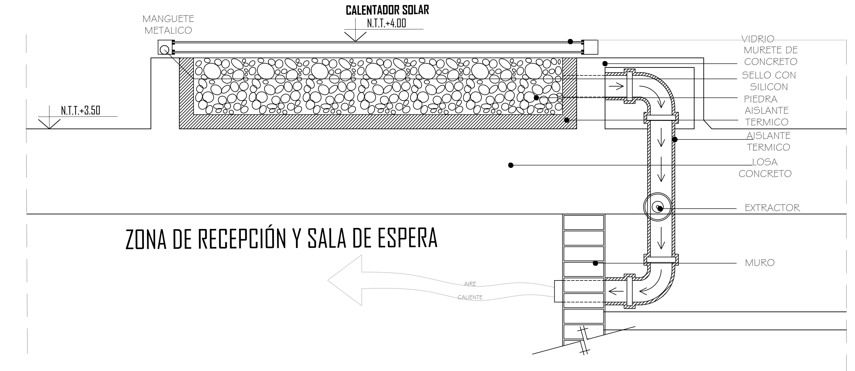
DETALLE C -CALENTADOR SOLAR DE AIRE PARA ACONDICIONAMIENTO DE CLIMA INTERIOR ESCALA 1/5
