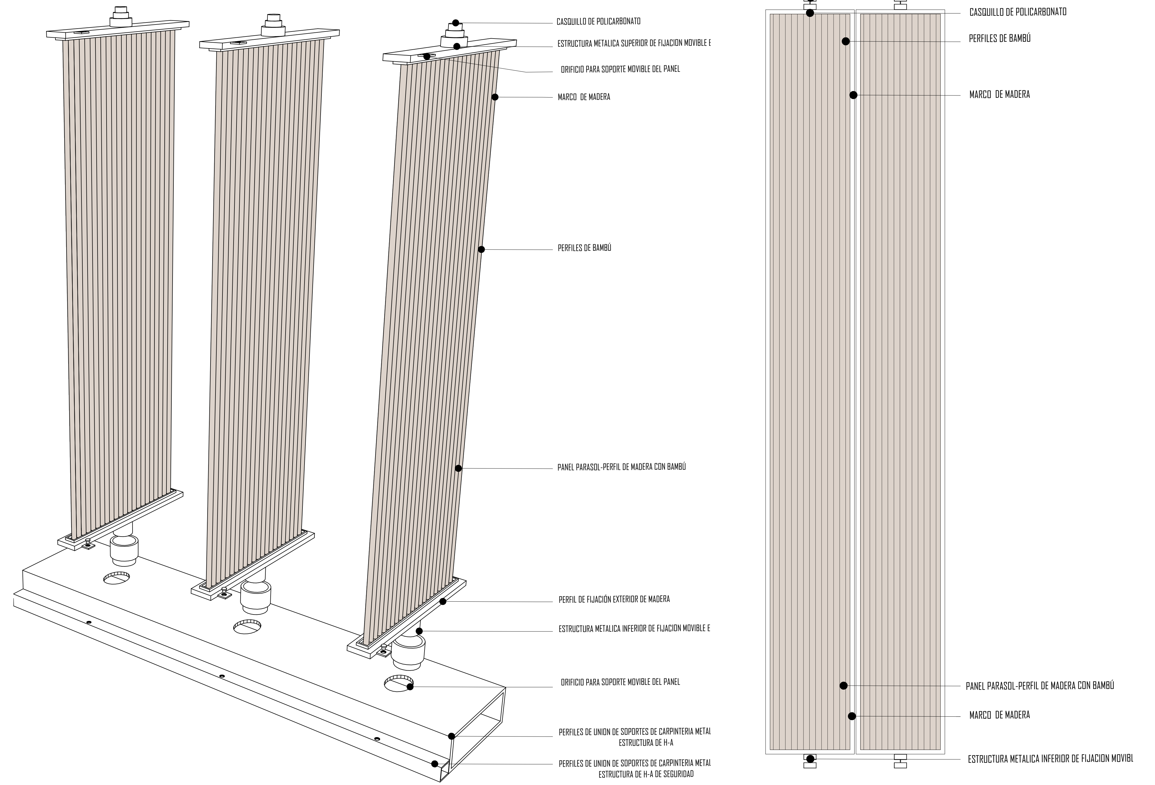
DETALLE DE PARASOL-PANEL CON PERFILES DE BAMBÚ ESCALA 1/10
