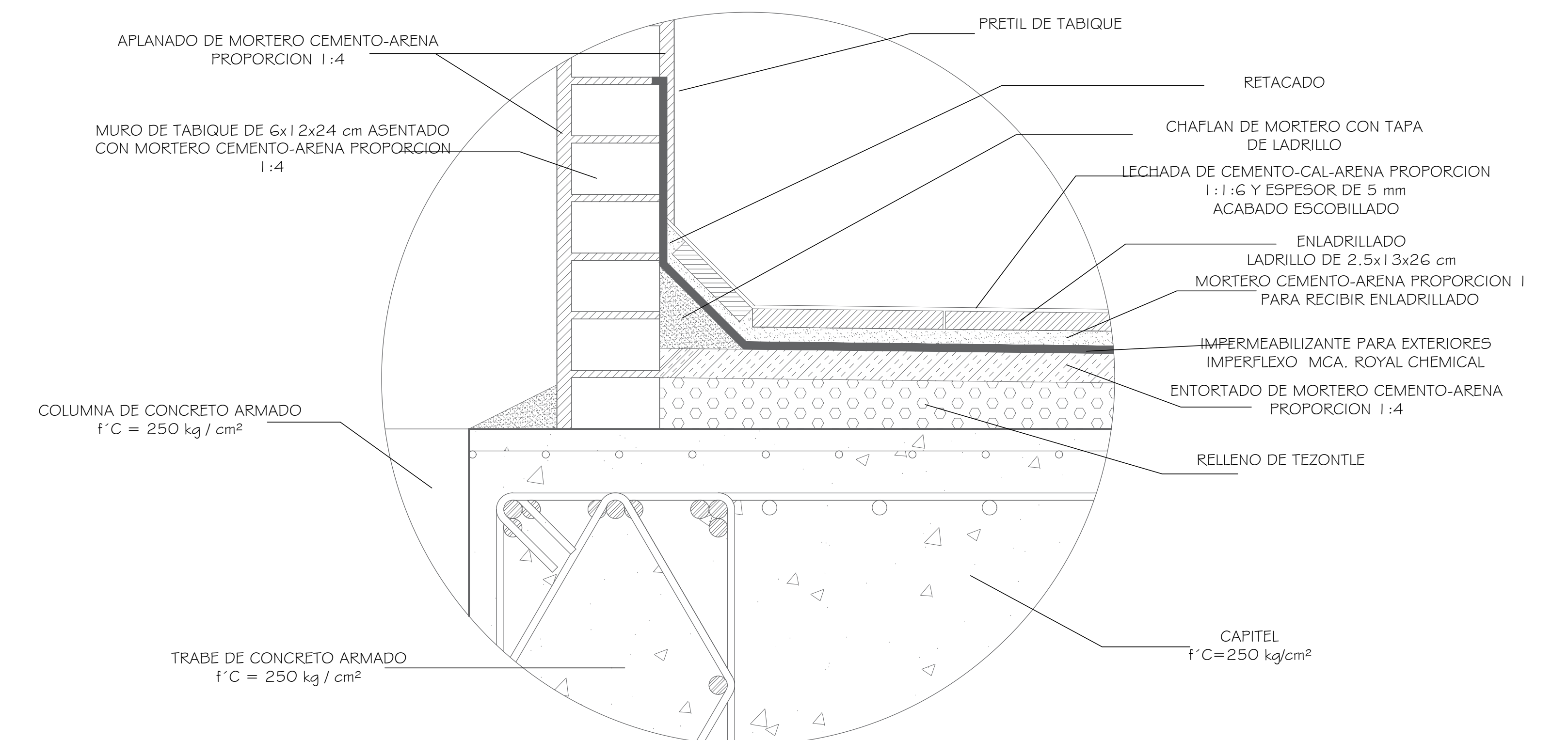
DETALLE B DE CHAFLAN Y PISO IMPERMEABILIZABLE ESCALA 1/5
