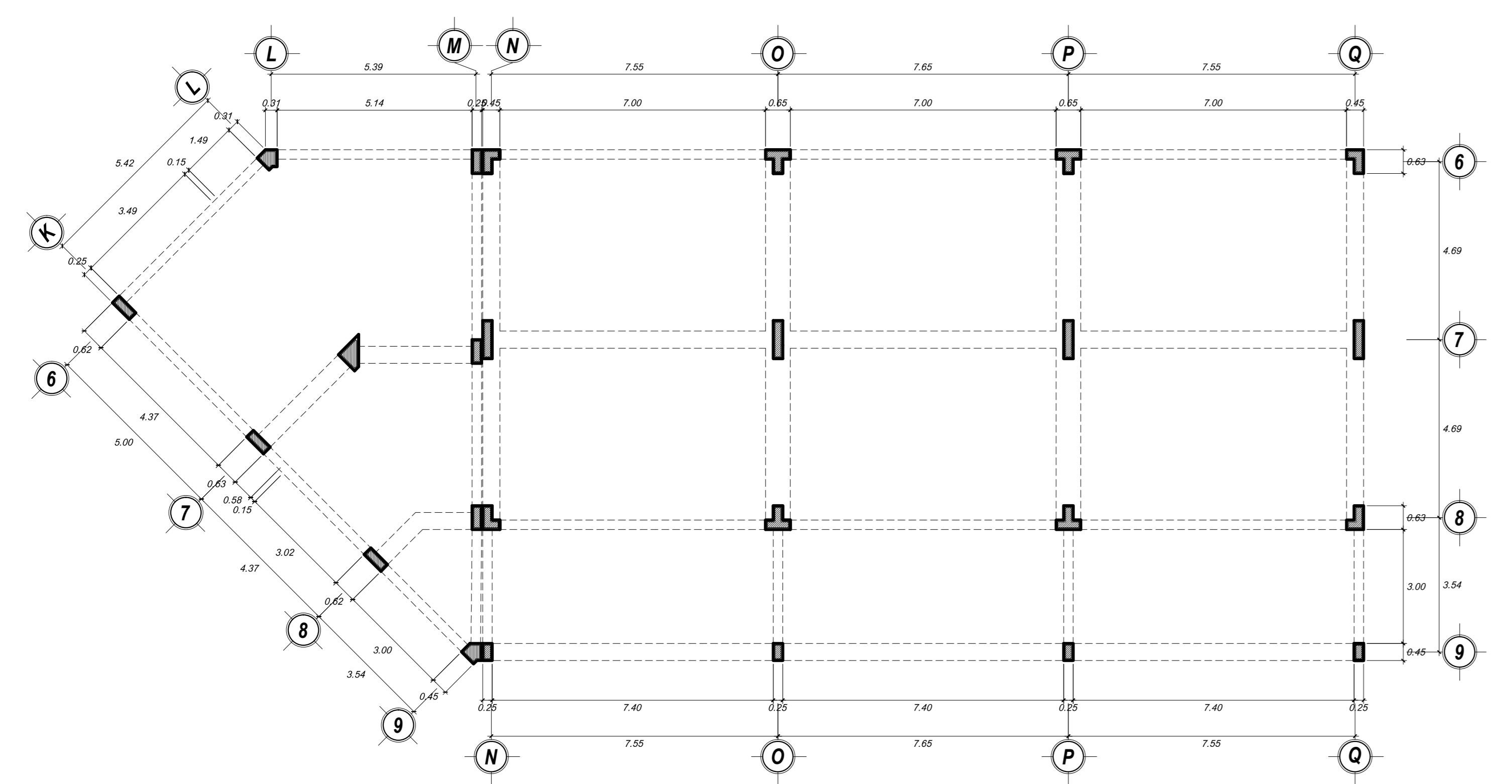
ESQUEMA ESTRUCTURAL PABELLON ESCALA 1/100
