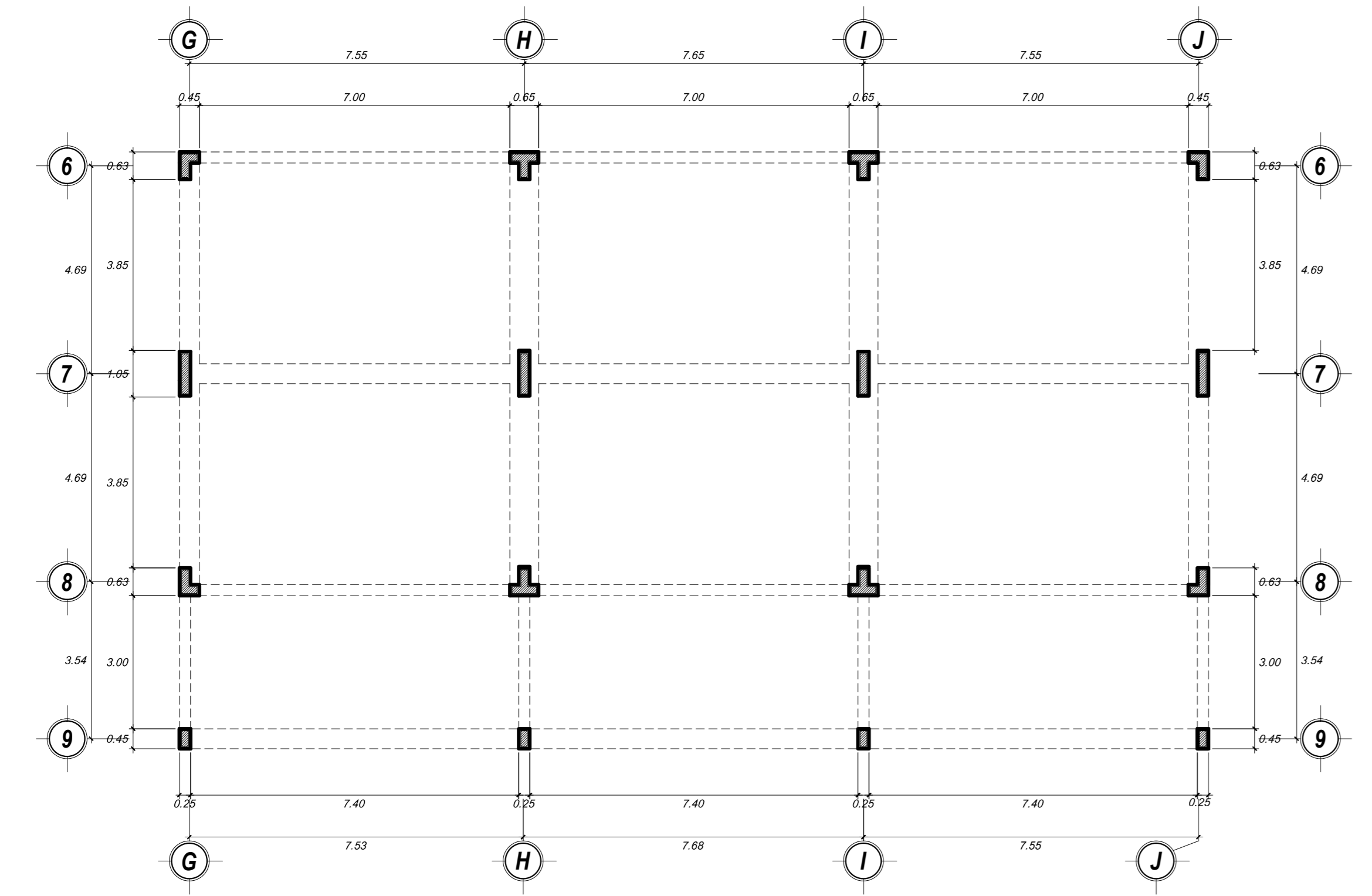
ESQUEMA ESTRUCTURAL PABELLON ESCALA 1/100
