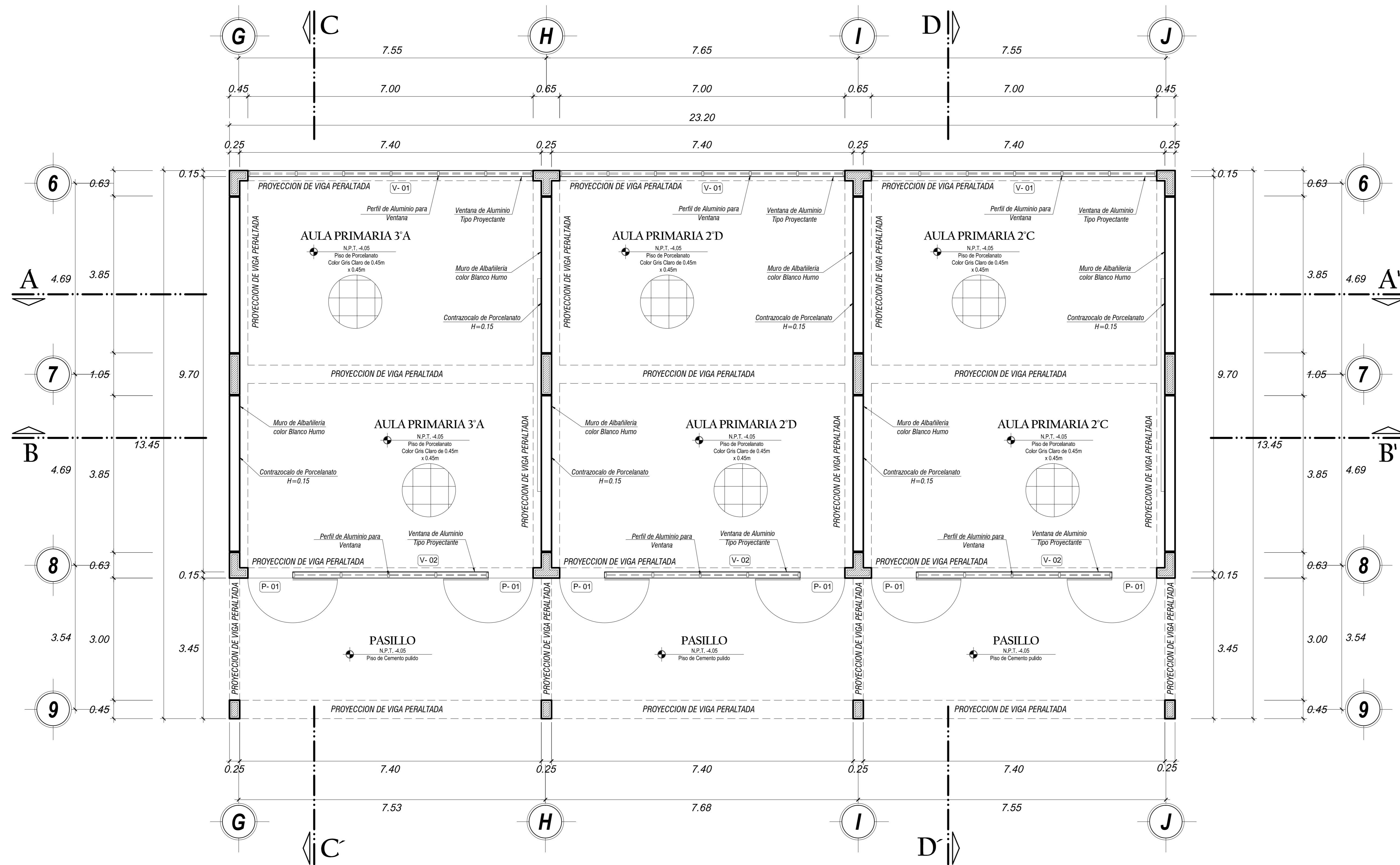
SEGUNDO NIVEL BLOQUE PABELLON ESCALA 1/50
