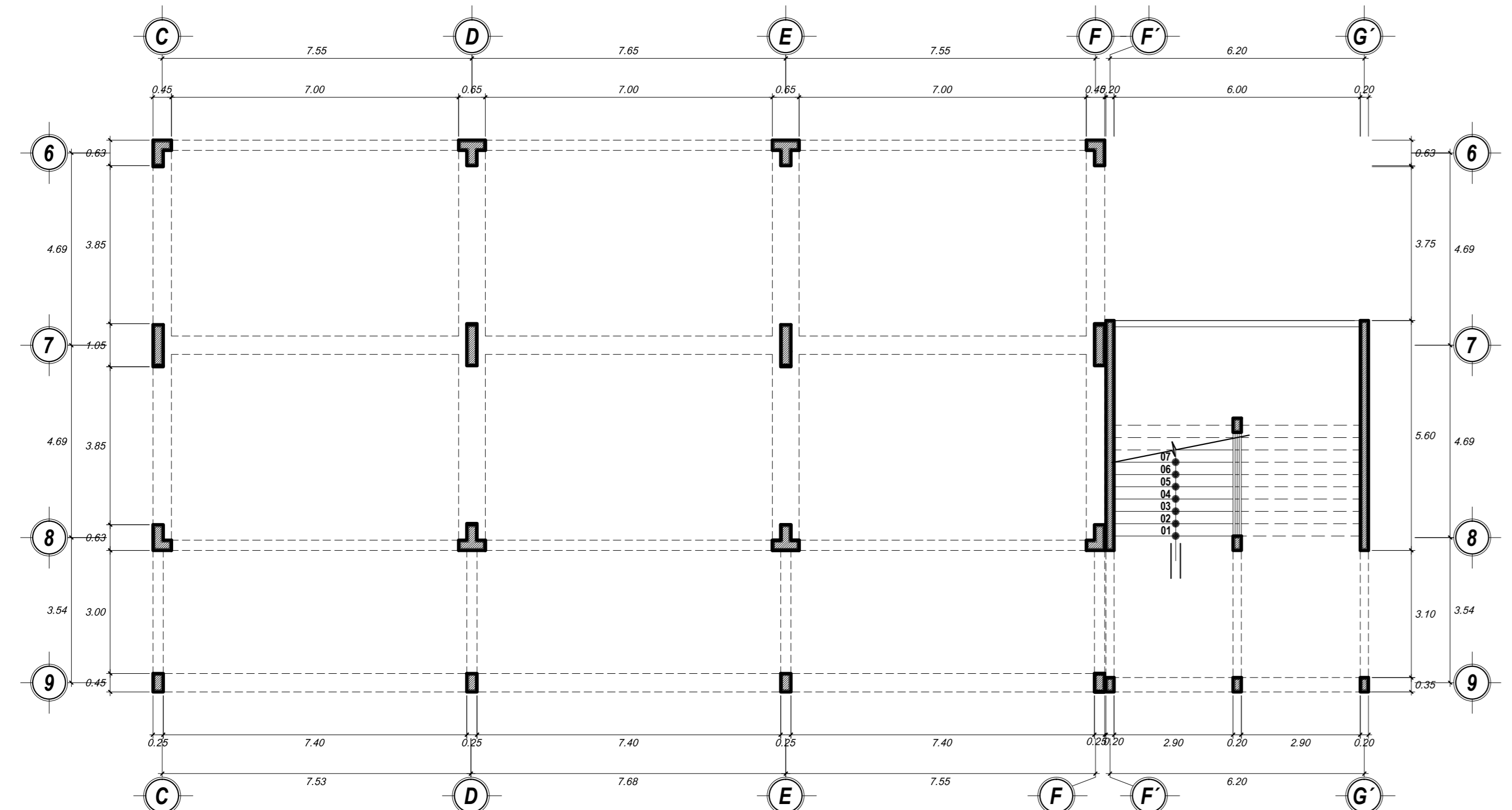
ESQUEMA ESTRUCTURAL PABELLON ESCALA 1/100
