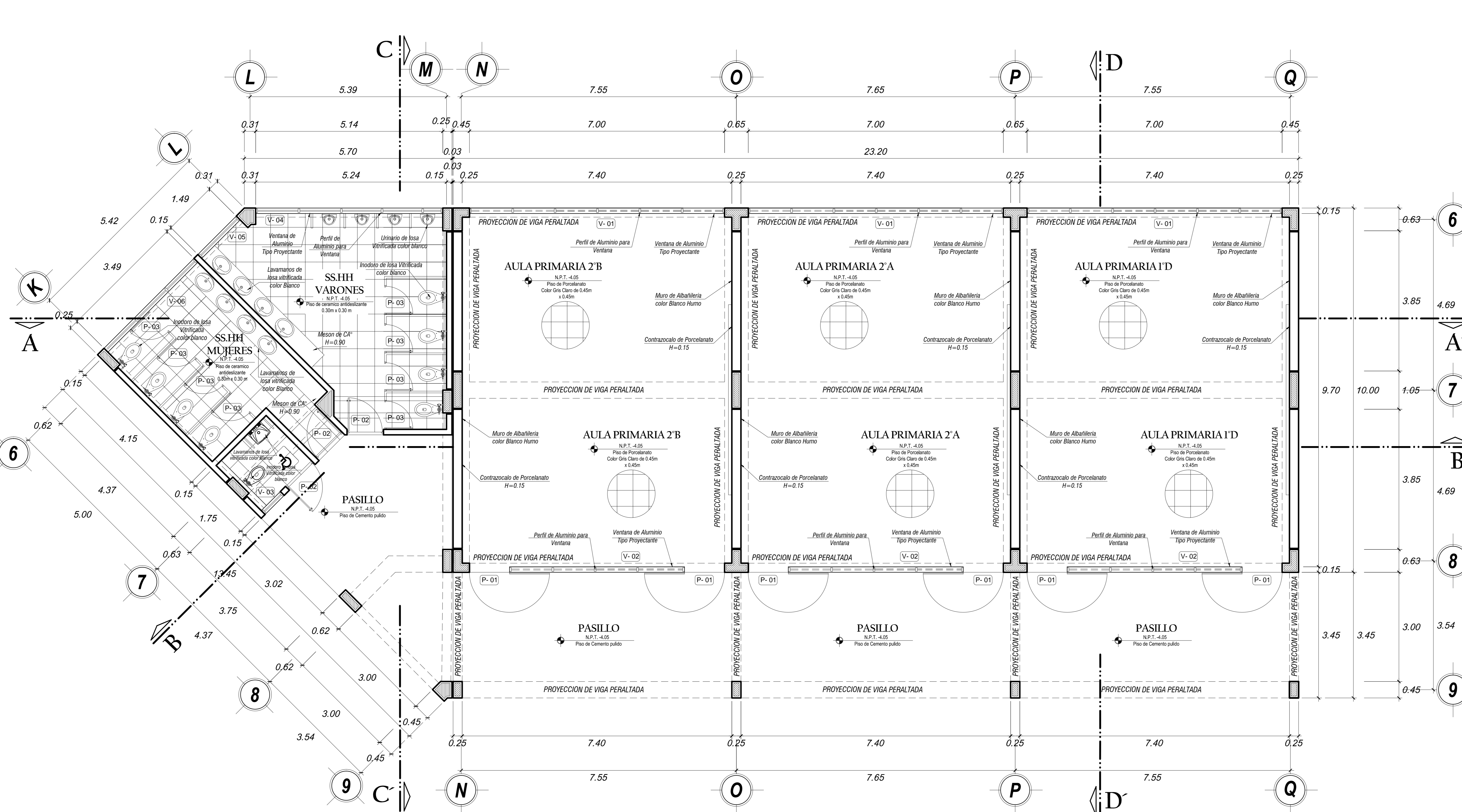
TERCER NIVEL BLOQUE PABELLON ESCALA 1/50
