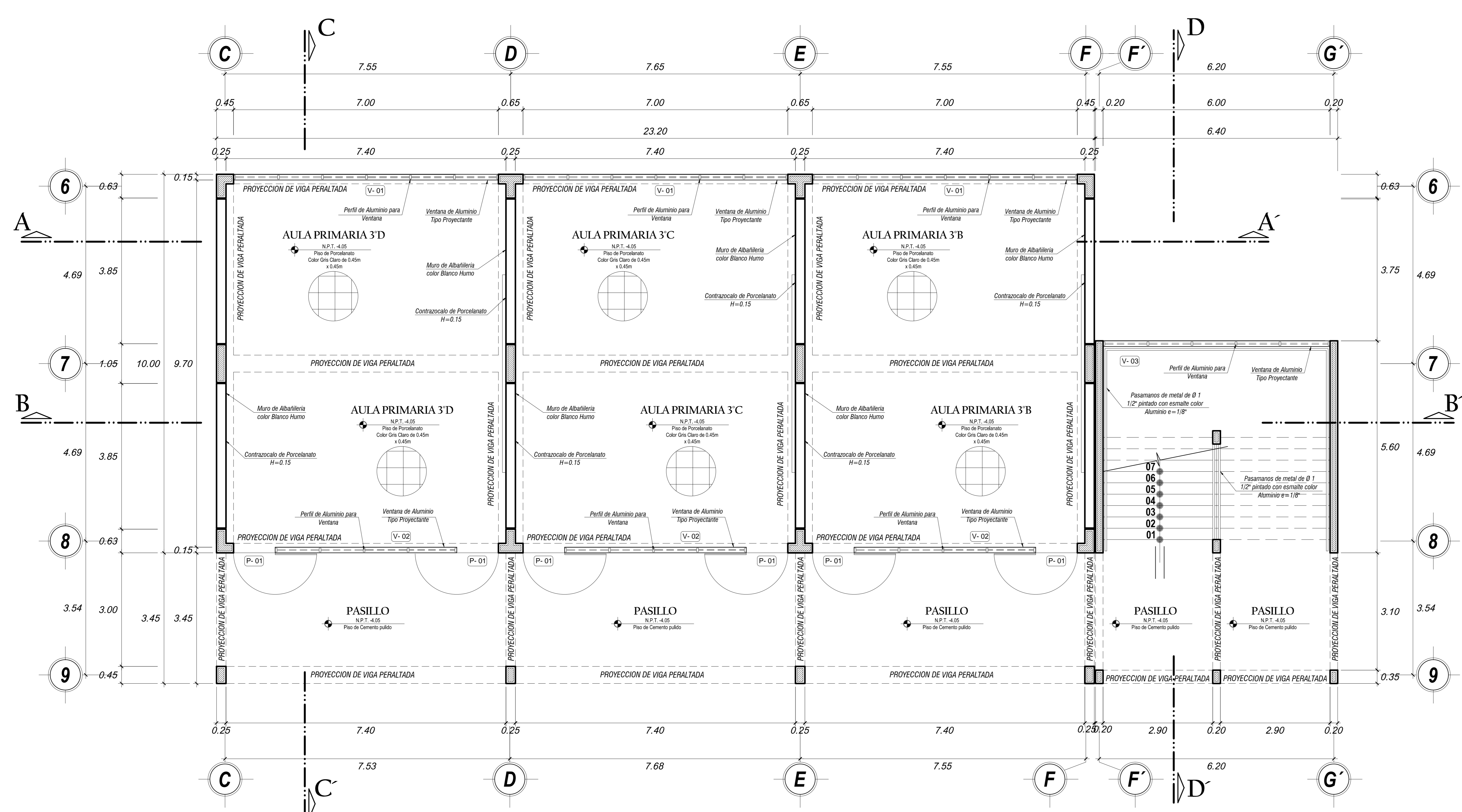
PRIMER NIVEL BLOQUE PABELLON ESCALA 1/50
