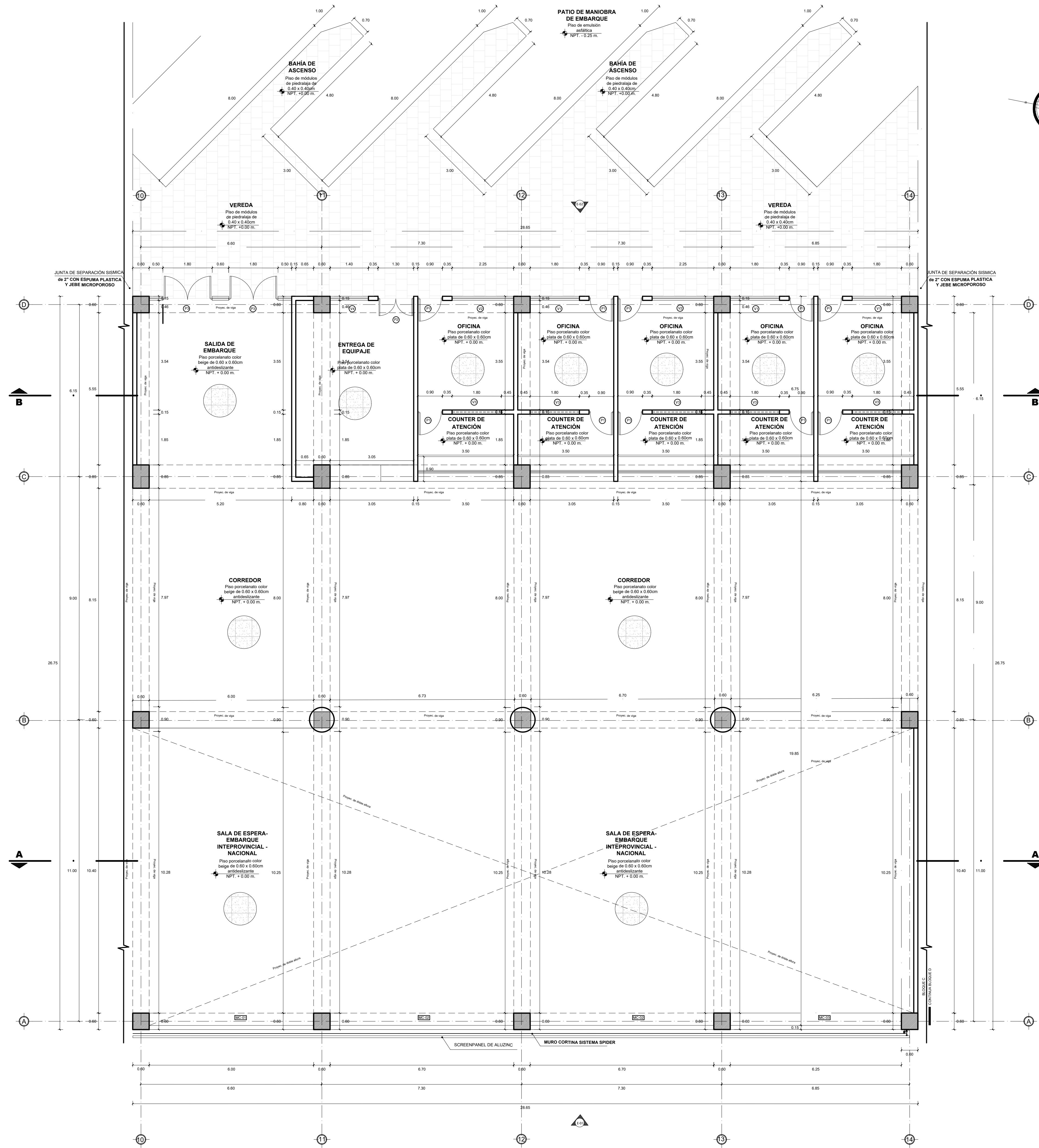
PLANTA DE DISTRIBUCIÓN - 1ER NIVEL - BLOQUE C ZONA DE EMBARQUE ESCALA 1 / 75
