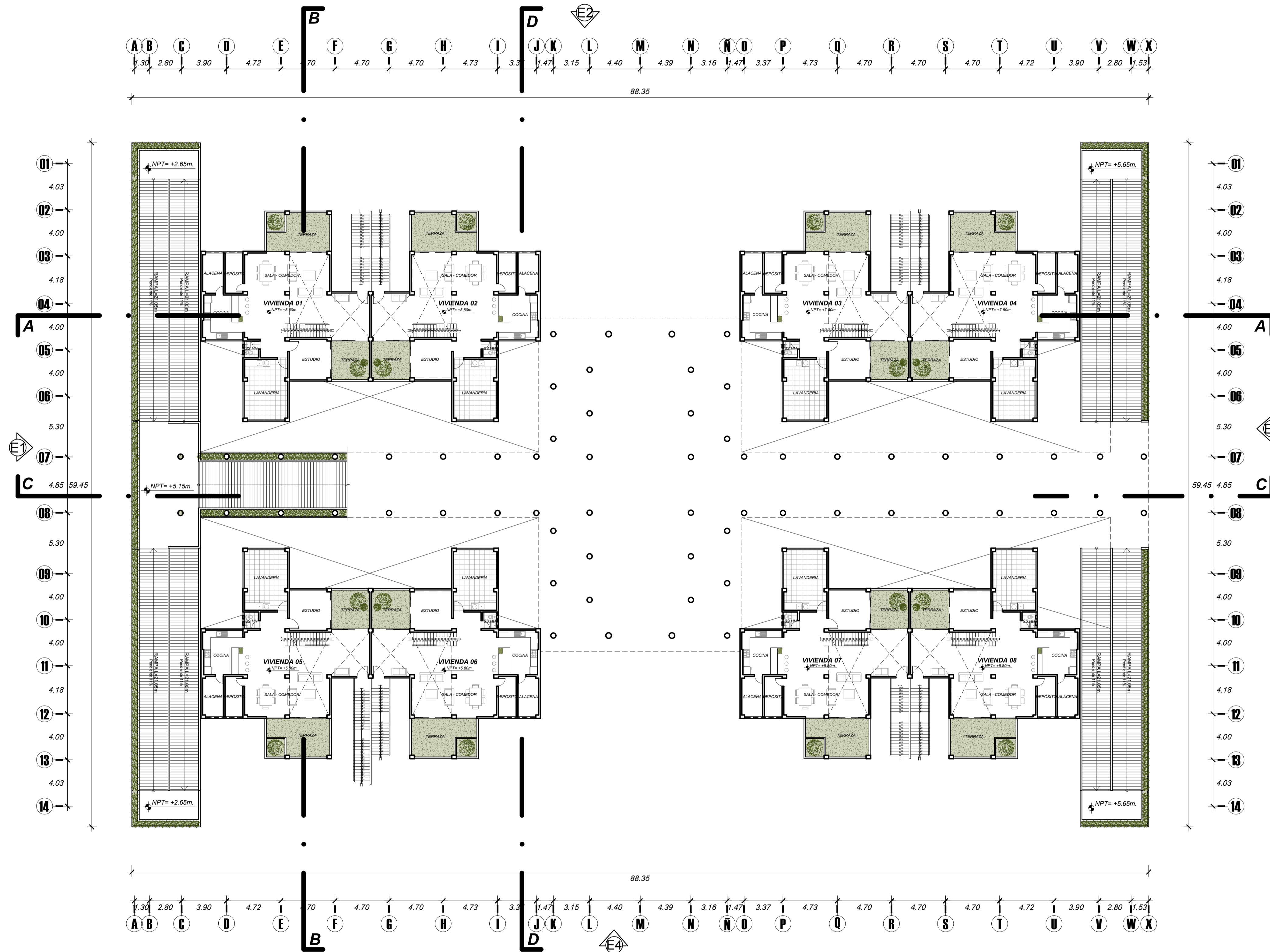
PLANO DE DISTRIBUCION PROYECTO DE VIVIENDA TALLER 2do Nivel Esc. 1/200
