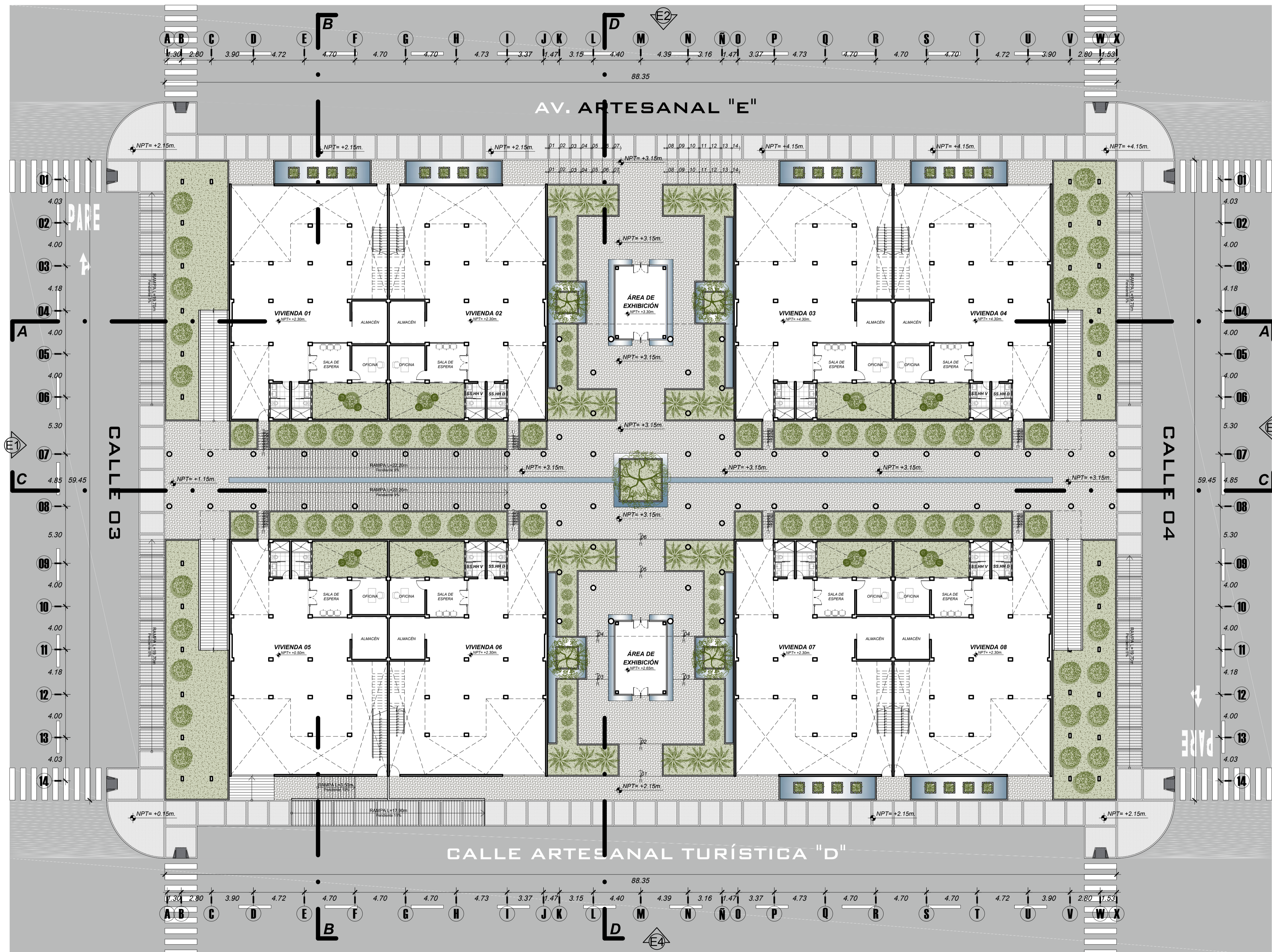
ARQUITECTURA PLANIMETRÍA GENERAL PROYECTO DE VIVIENDA TALLER Esc. 1/200
