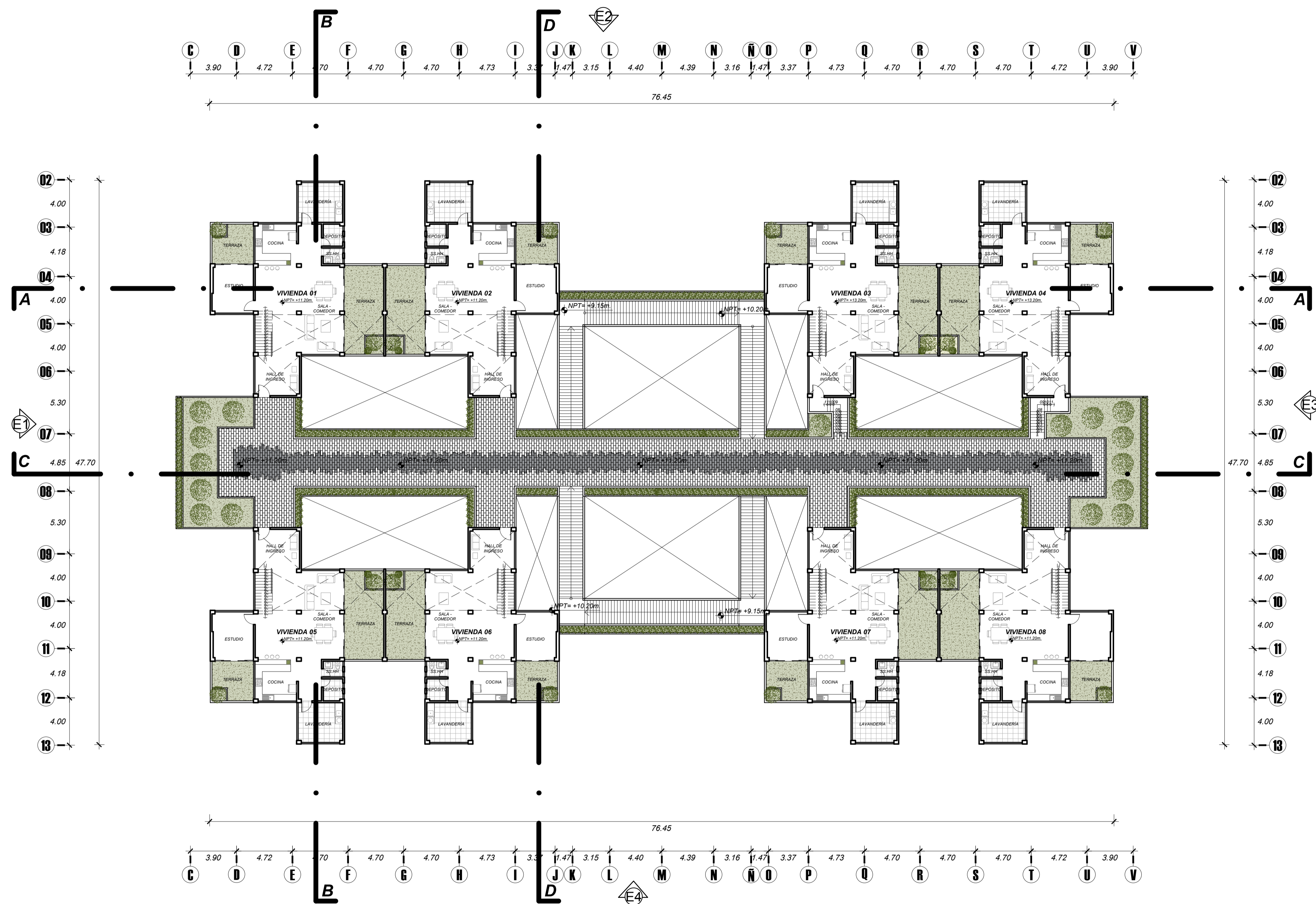
PLANO DE DISTRIBUCION PROYECTO DE VIVIENDA TALLER 4to Nivel Esc. 1/200
