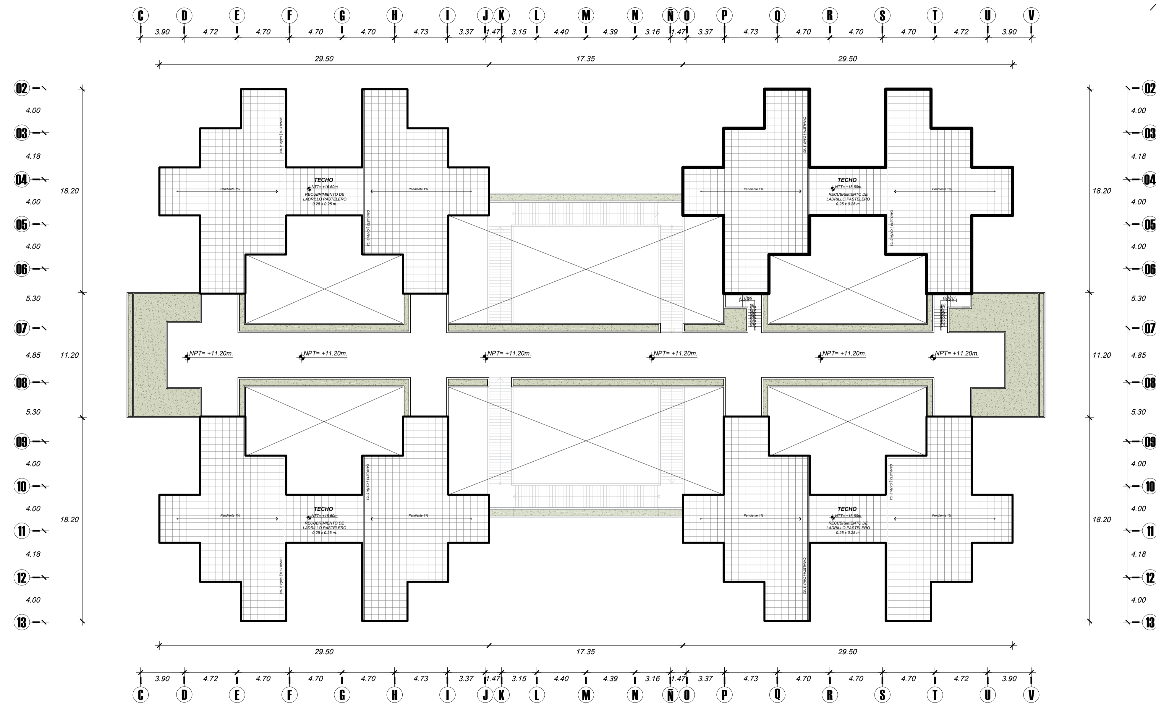
PLANO DE TECHOS esc. 1/200
