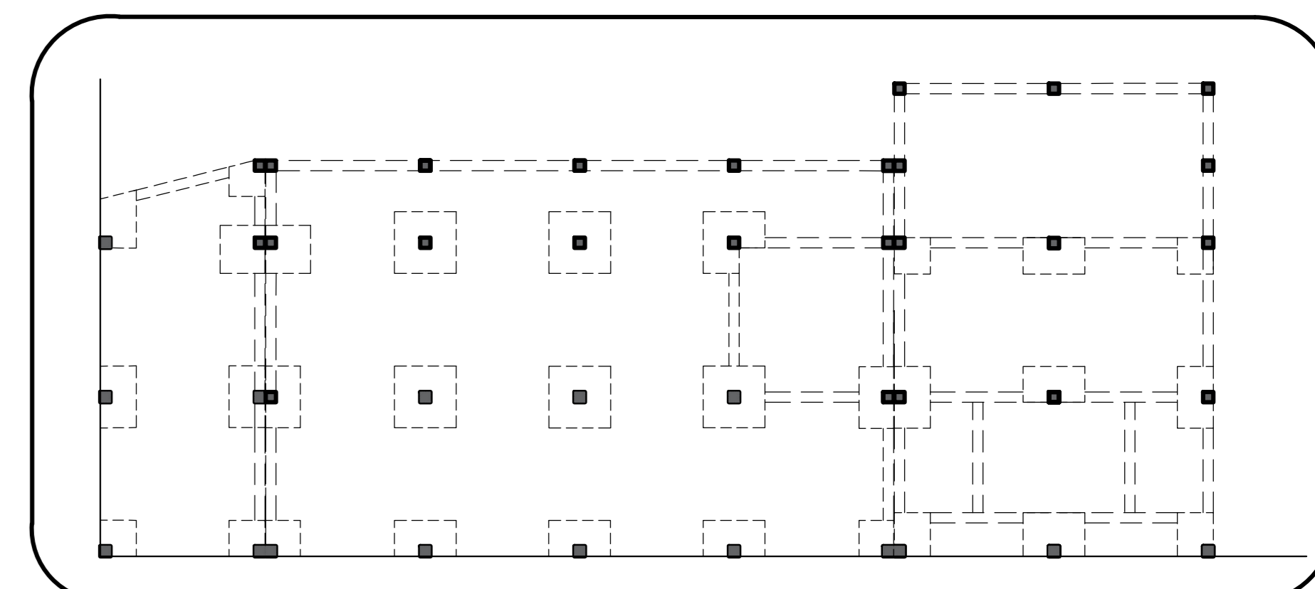
ESQUEMA ESTRUCTURAL DEL PROYECTO COMPONENTE: SALA DE DESEMBARQUE
