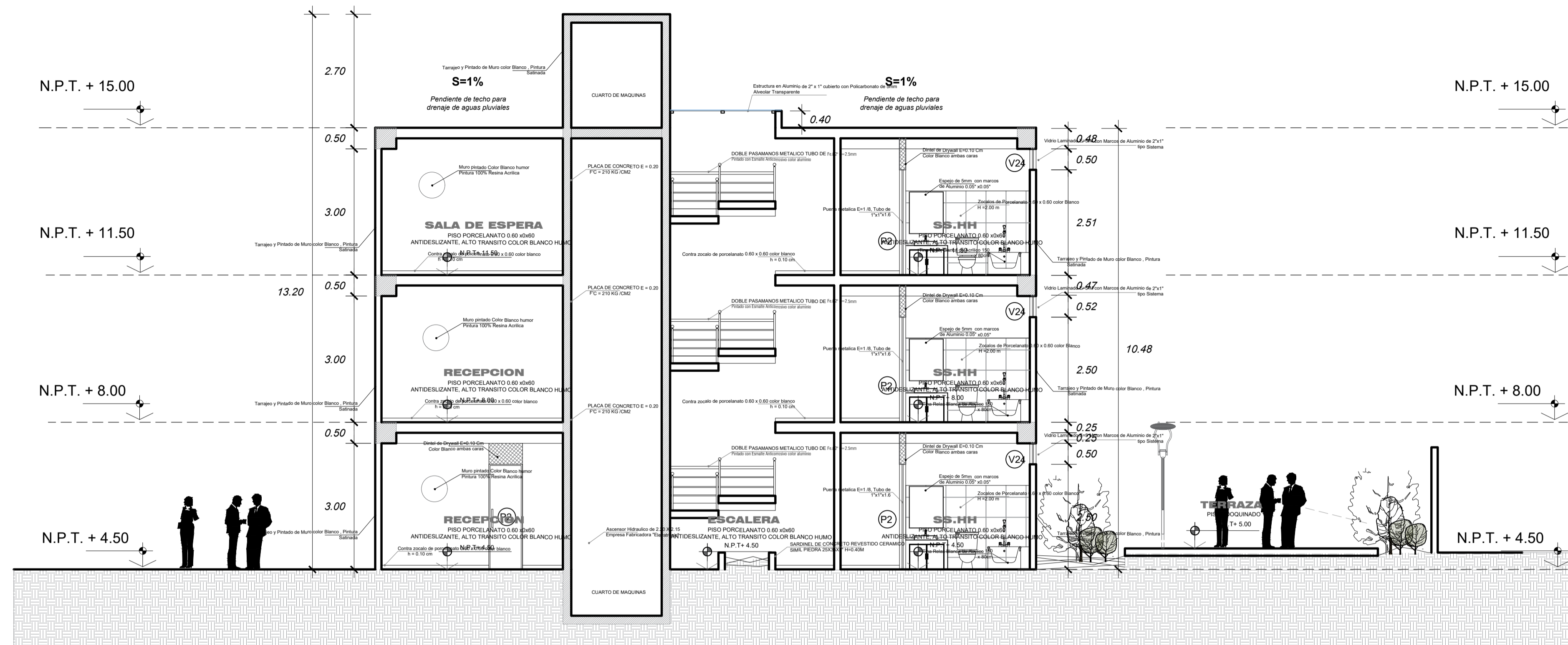
CORTE 5-A escala 1:75 BLOQUE
