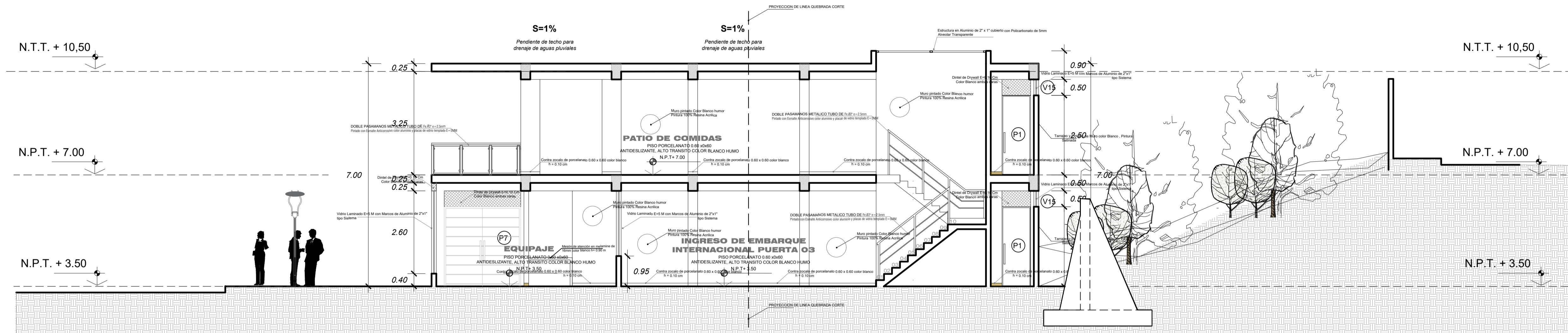
CORTE 3-A escala 1:75 BLOQUE
