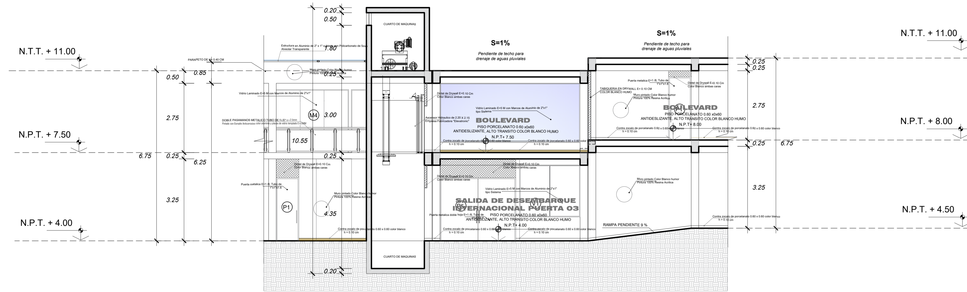
CORTE 4-A escala 1:75 BLOQUE
