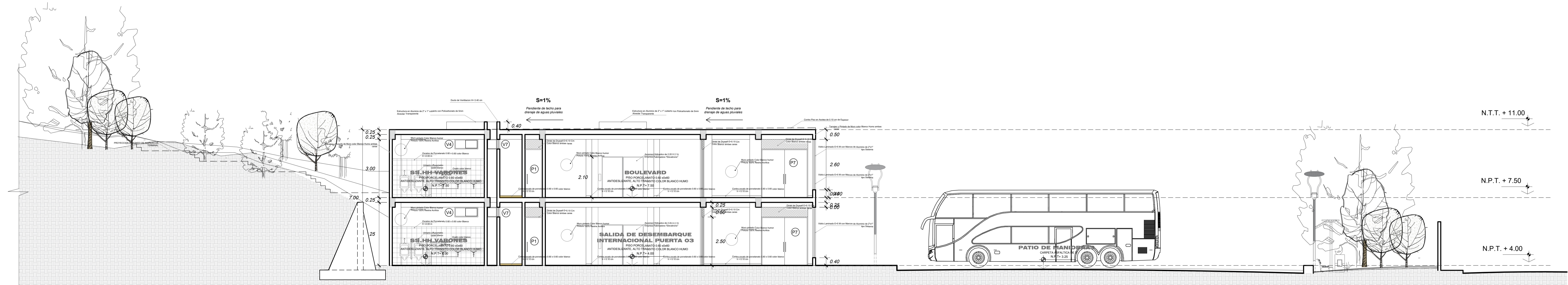
CORTE 4-B escala 1:75 BLOQUE
