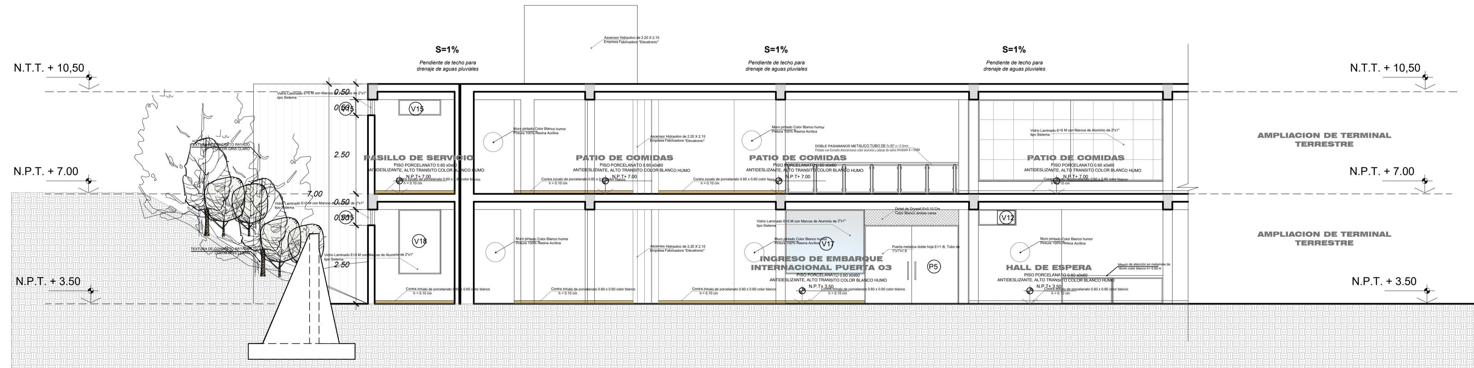
CORTE 3-B escala 1:75 BLOQUE
