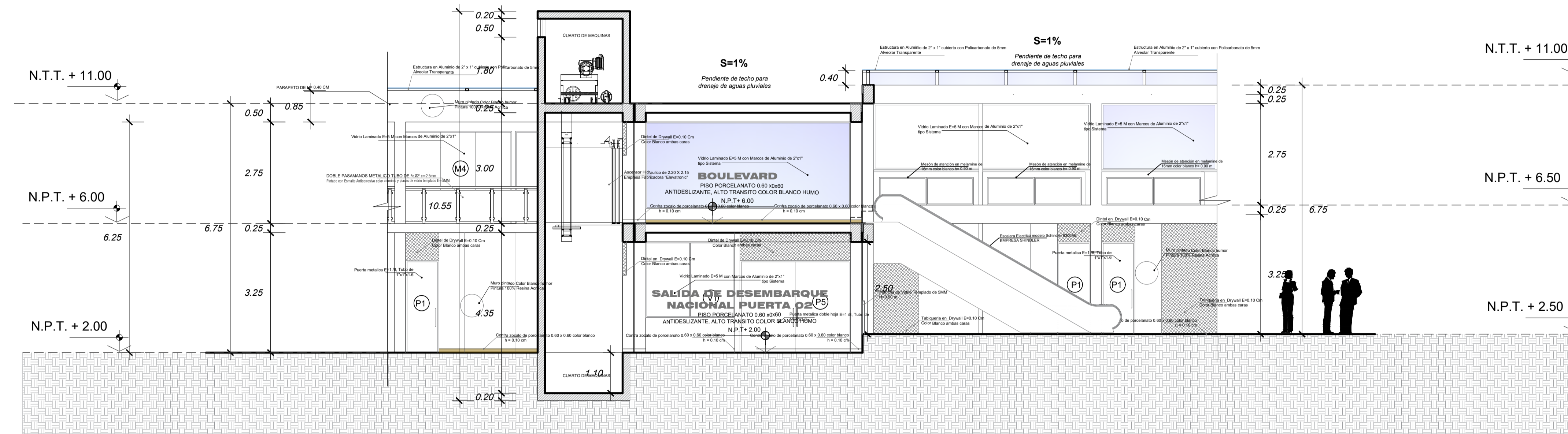
CORTE 2-A ARQUITECTURA escala 1:75 BLOQUE
