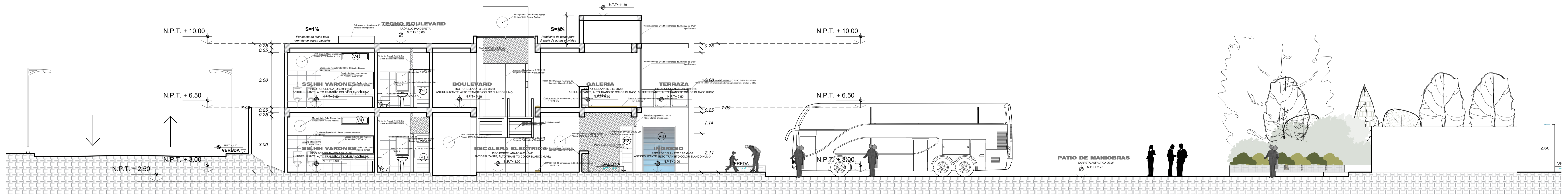
CORTE 2-B ARQUITECTURA escala 1:75 BLOQUE
