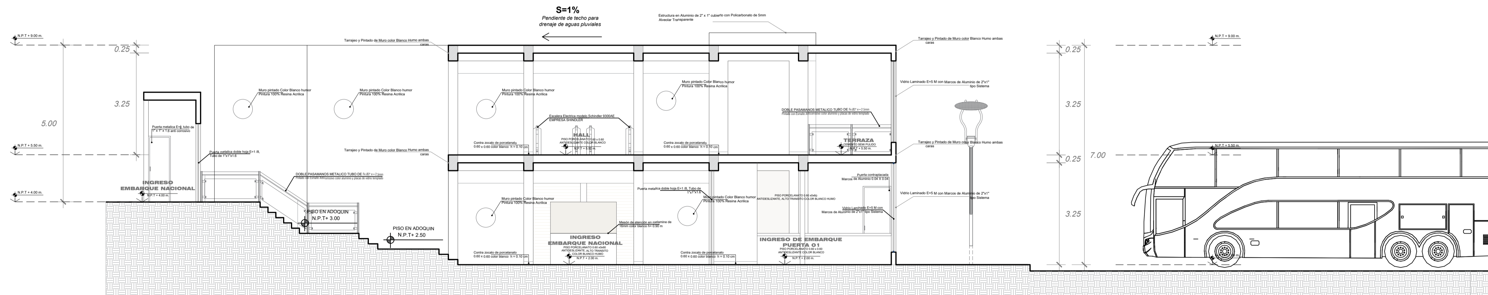
CORTE 1-B escala 1:75 BLOQUE
