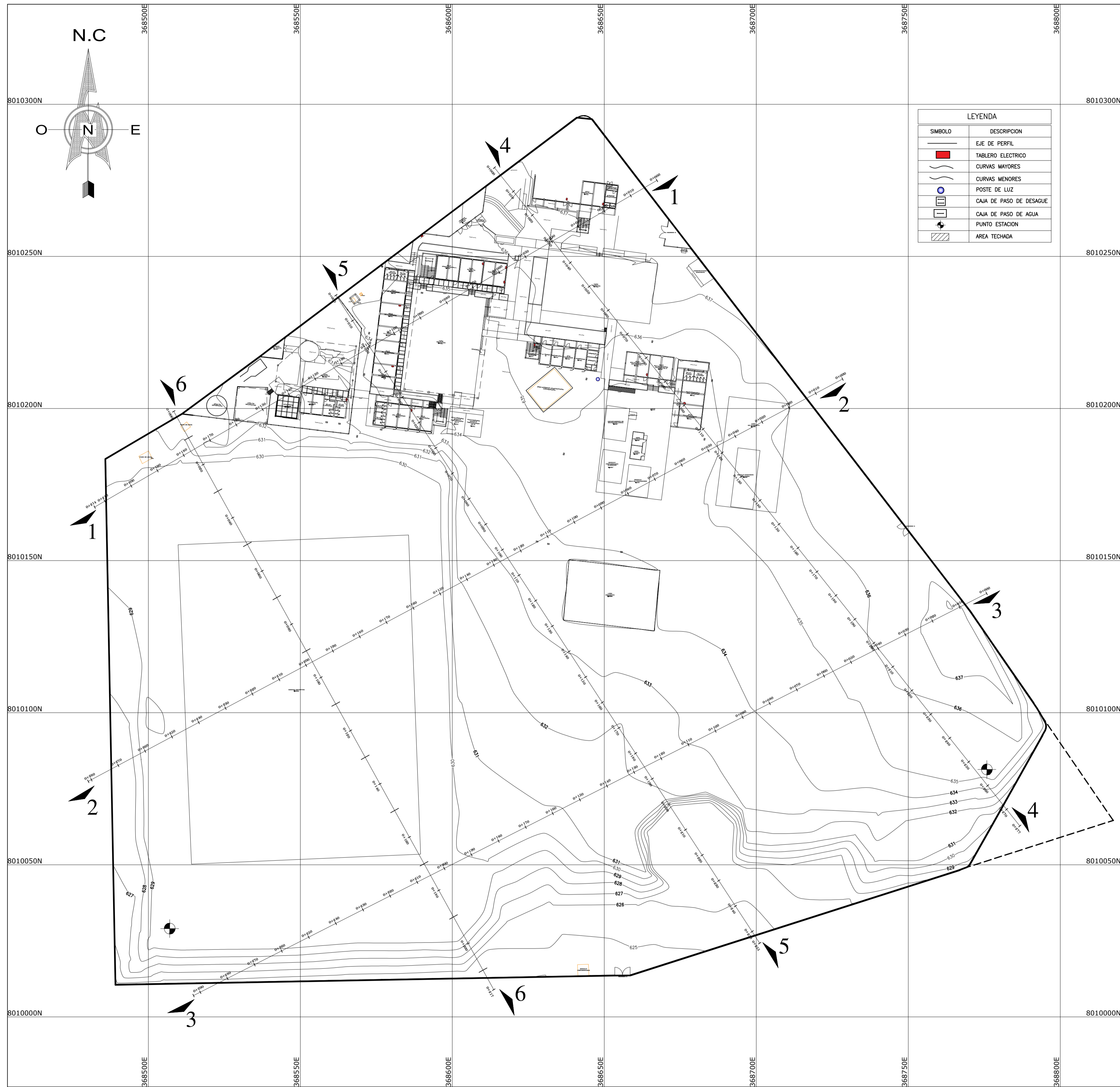
PLANO DE TOPOGRAFICO Esc. 1:750
