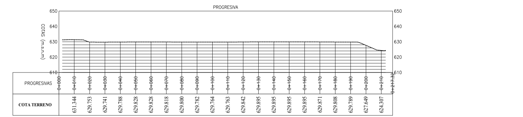
PERFIL 6 Esc. 1:1500
