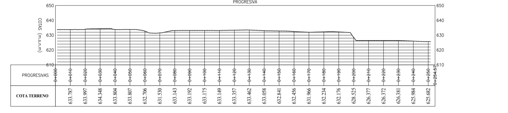
PERFIL 5 Esc. 1:1500
