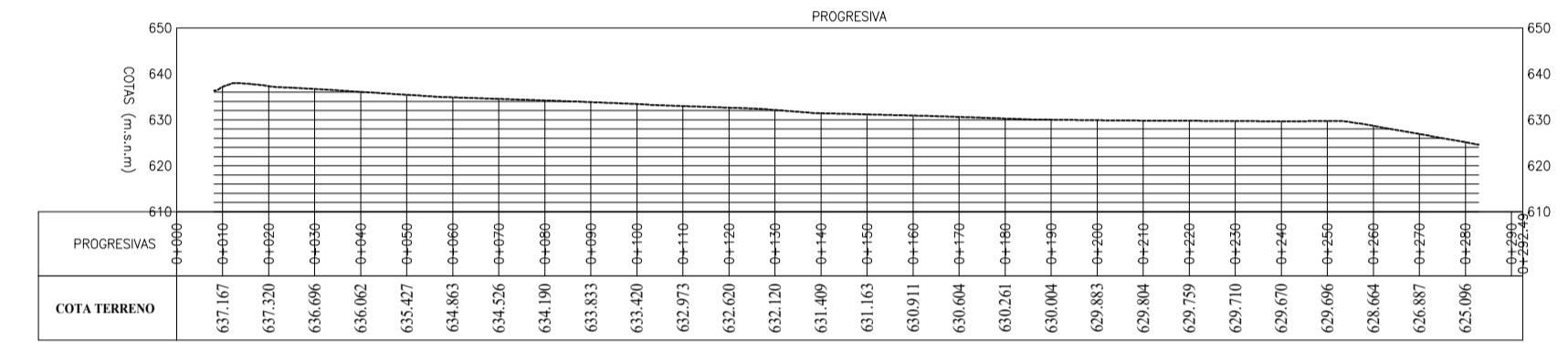
PERFIL 3 Esc. 1:1500
