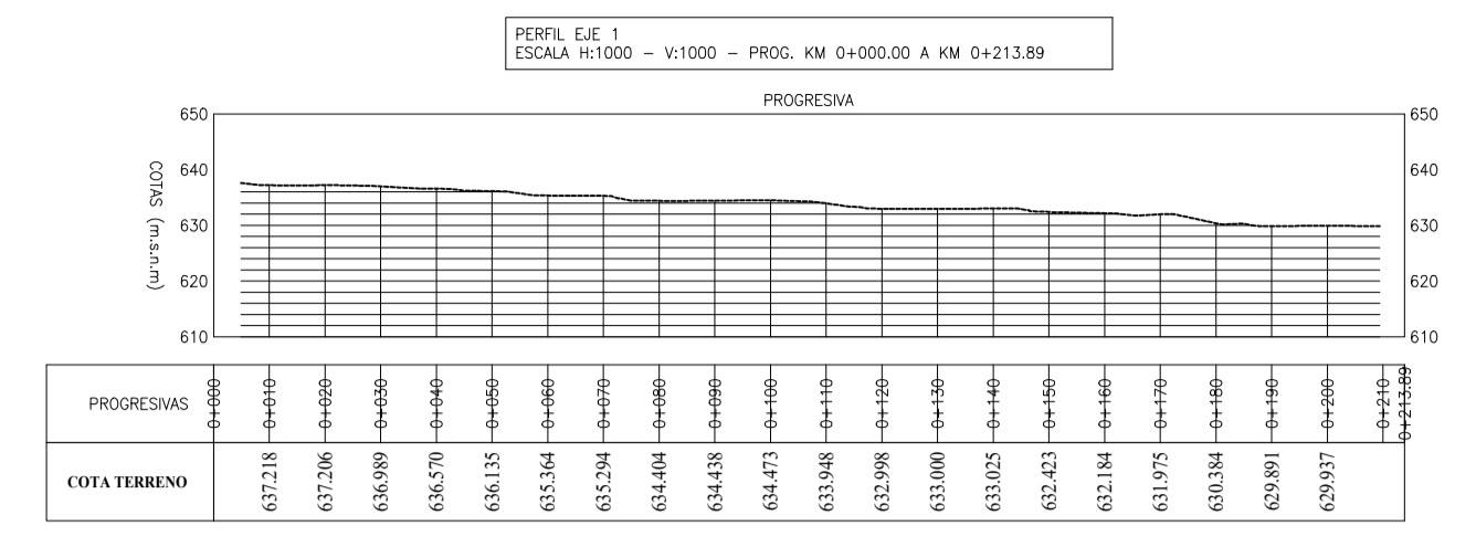
PERFIL 1 Esc. 1:1500
