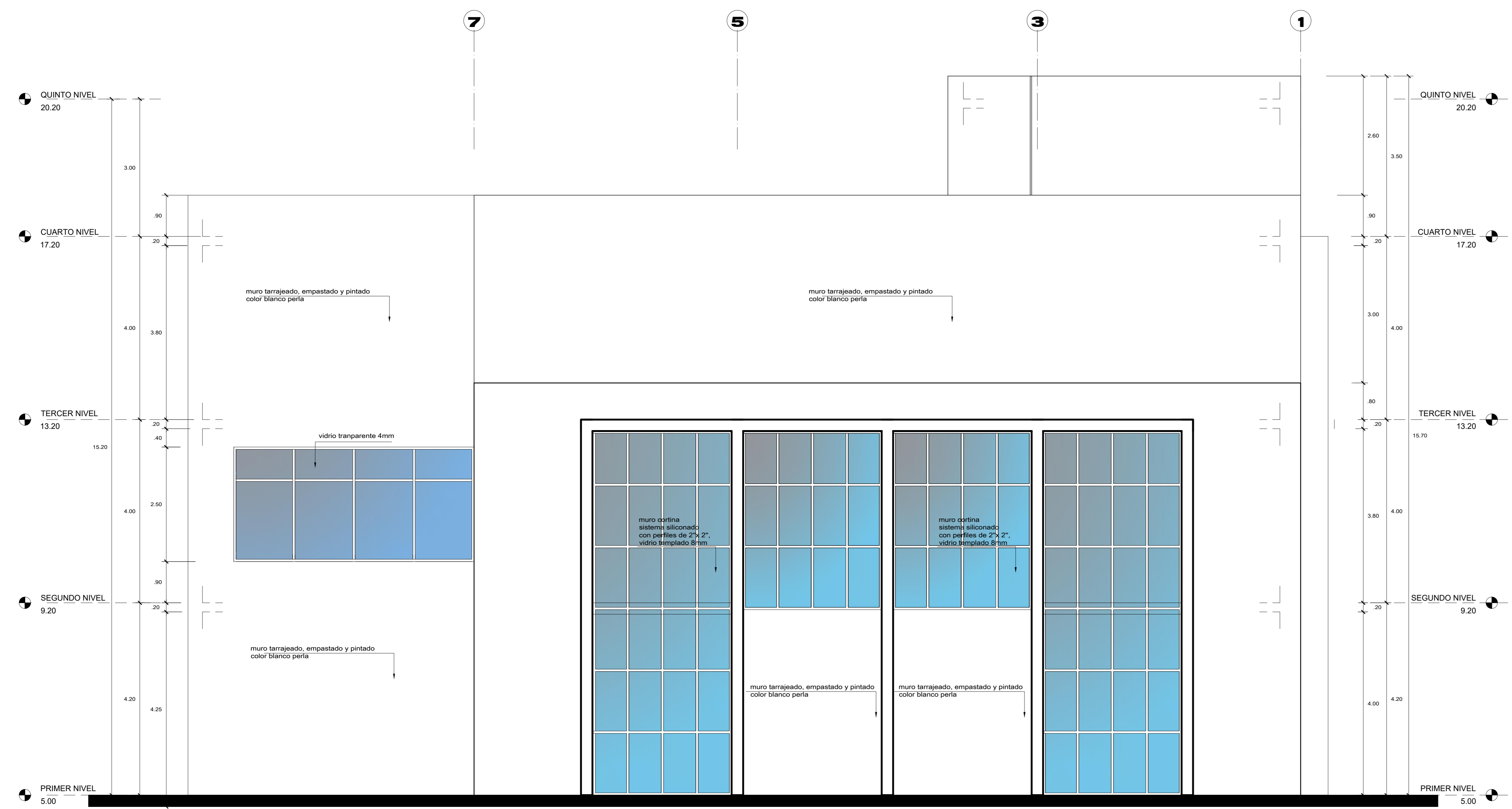
ELEVACION LATERAL E-4 ESCALA 1/50
