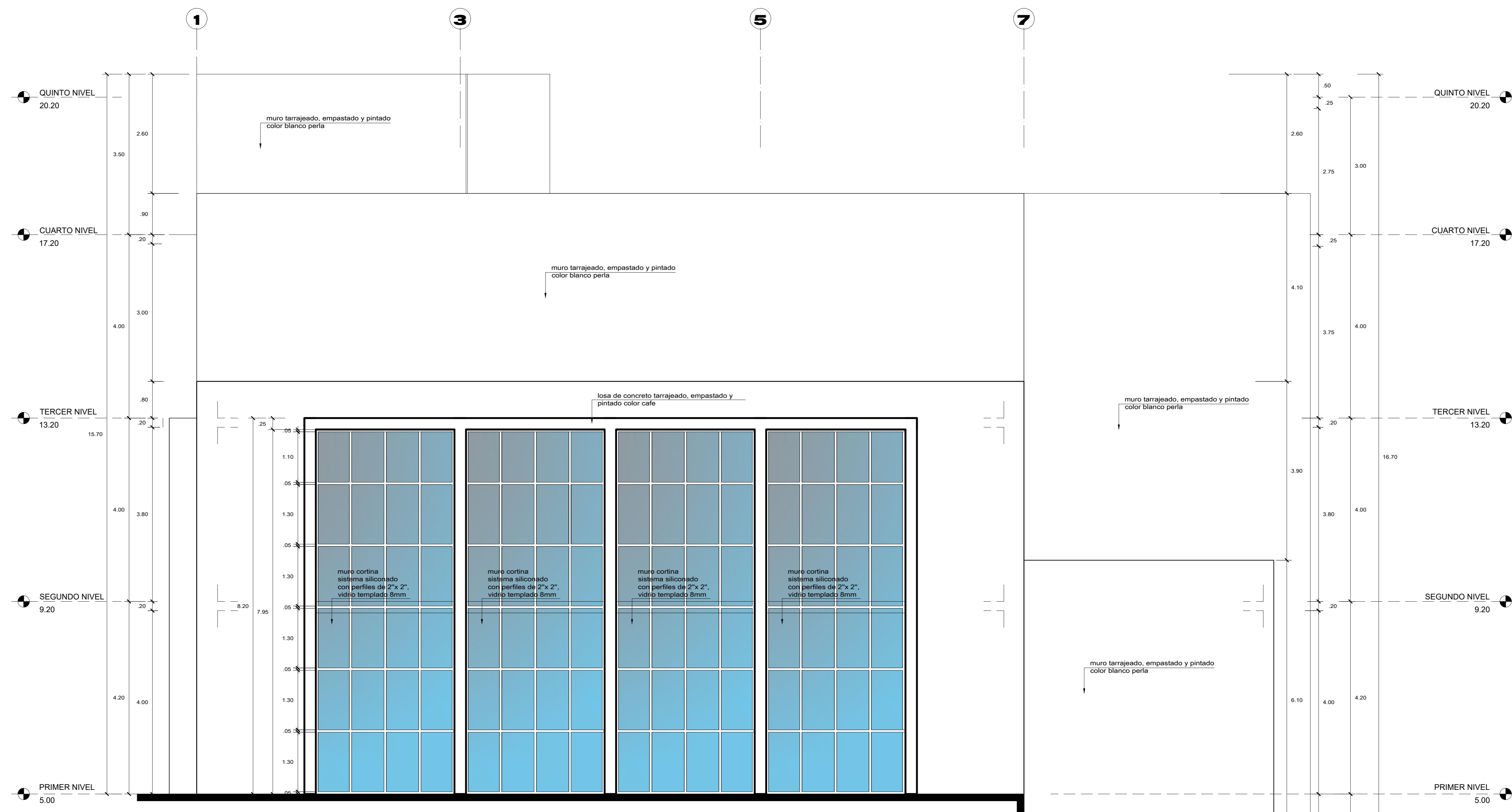
ELEVACION LATERAL E-3 ESCALA 1/50
