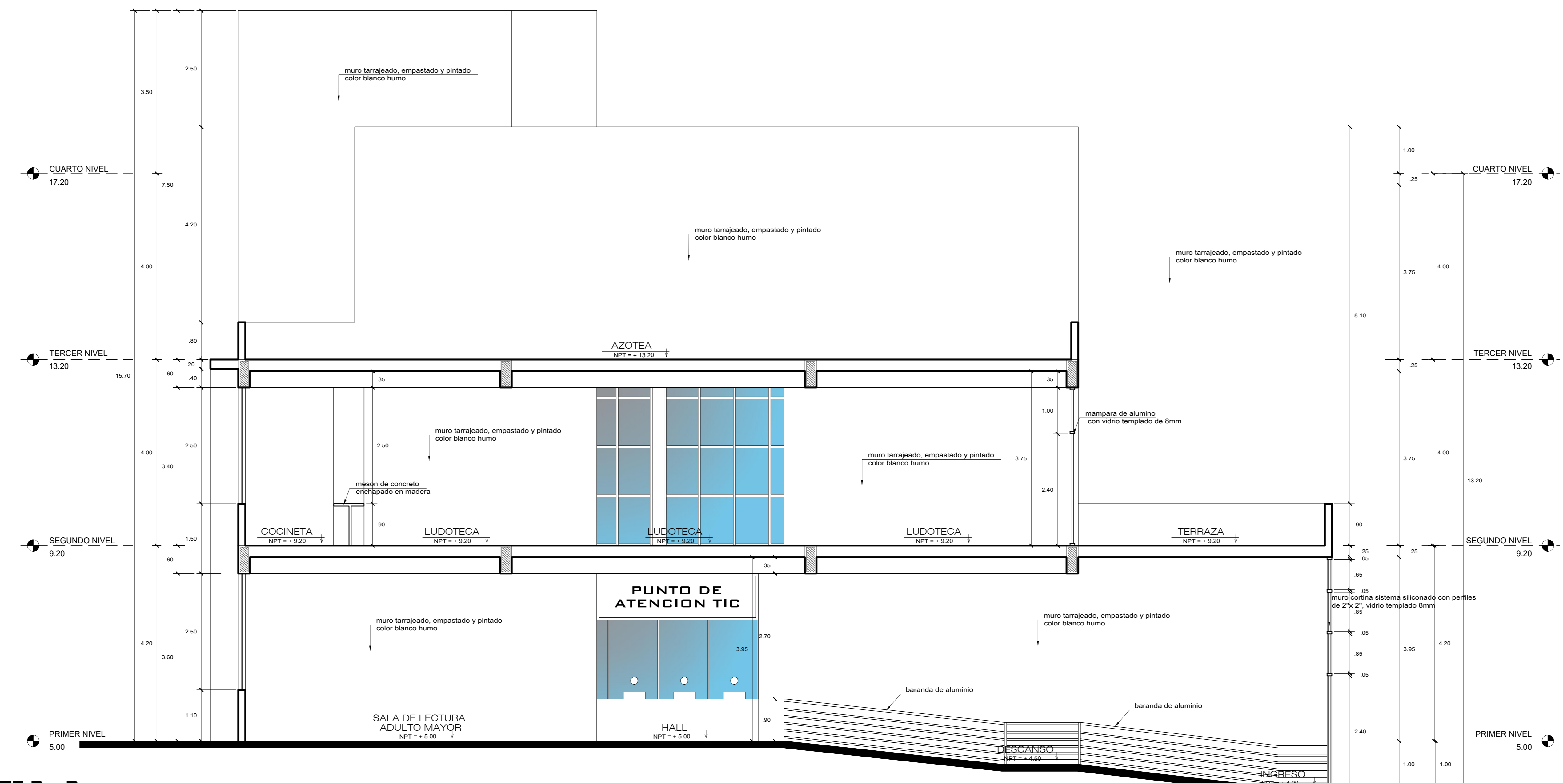
CORTE B - B ESCALA 1/50
