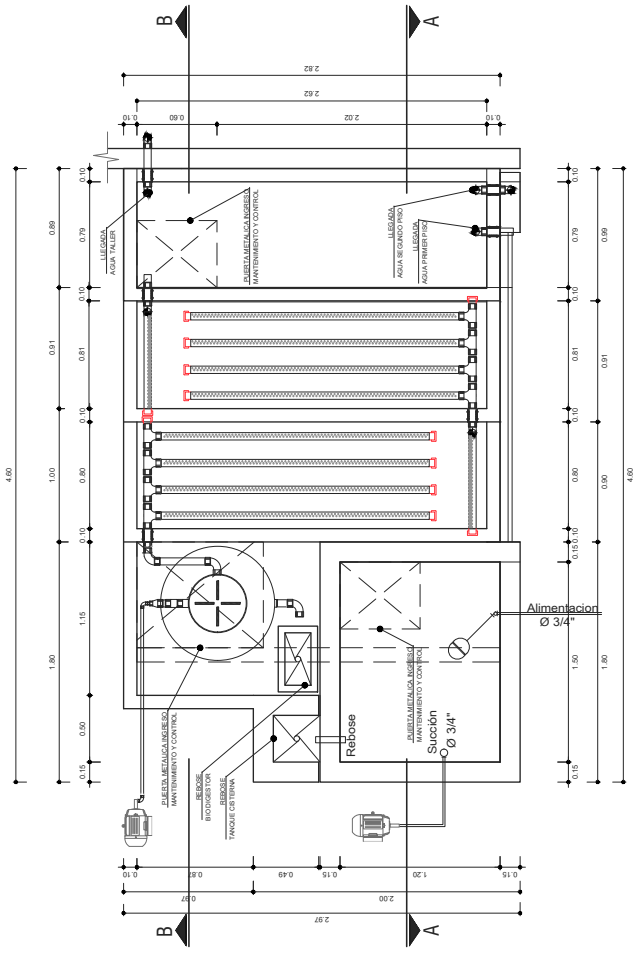
PLANTA DETALLE DE FILTRO BIOLÓGICO RECICLADO DE AGUAS GRISAS MÓDULO II ESC: 1/20
