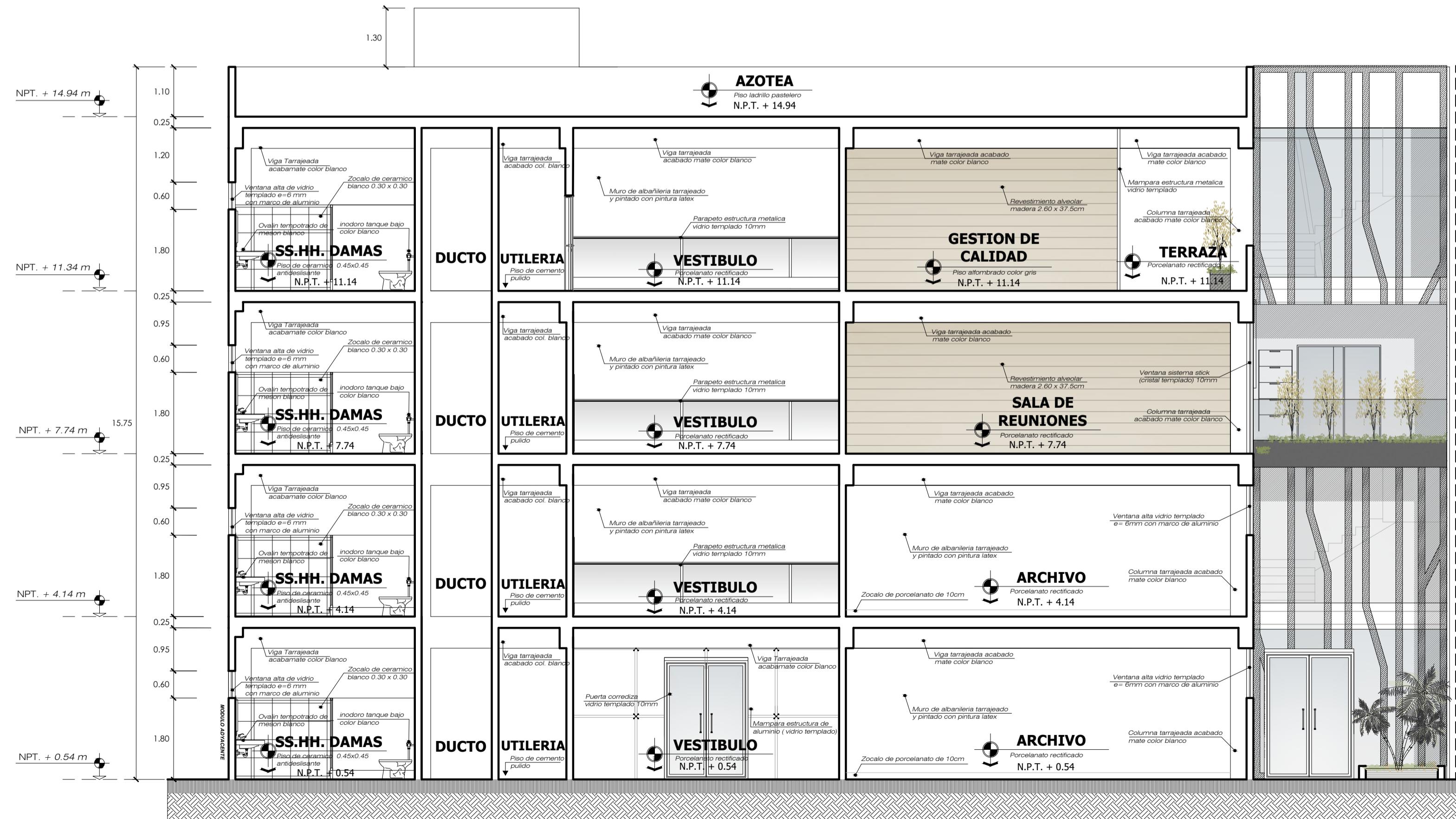
CORTE : LONGITUDINAL C - C' SECTOR 2 ESC.: 1 / 75
