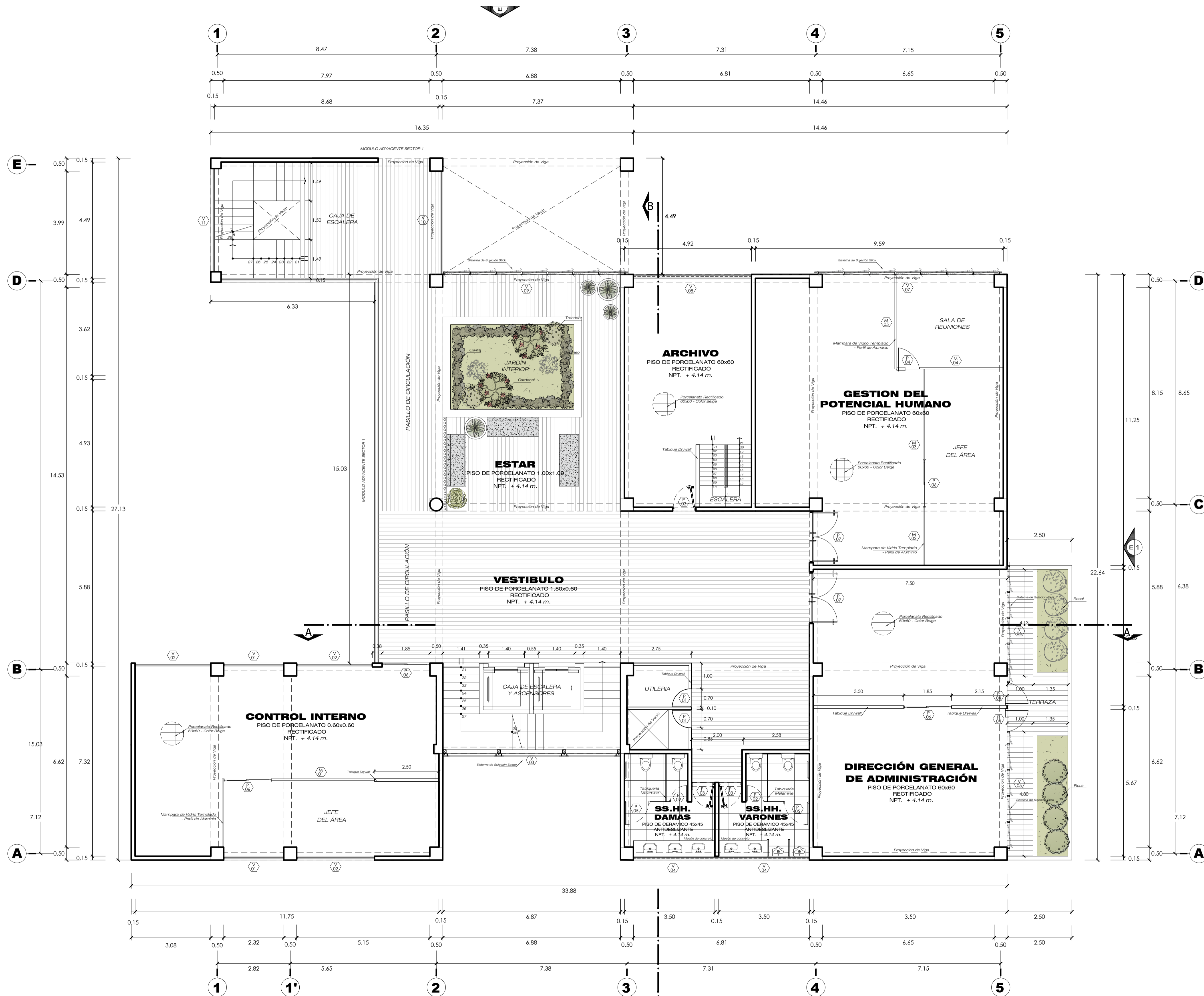
DISTRIBUCIÓN : SEGUNDO NIVEL SECTOR 2 ESC.: 1 / 75
