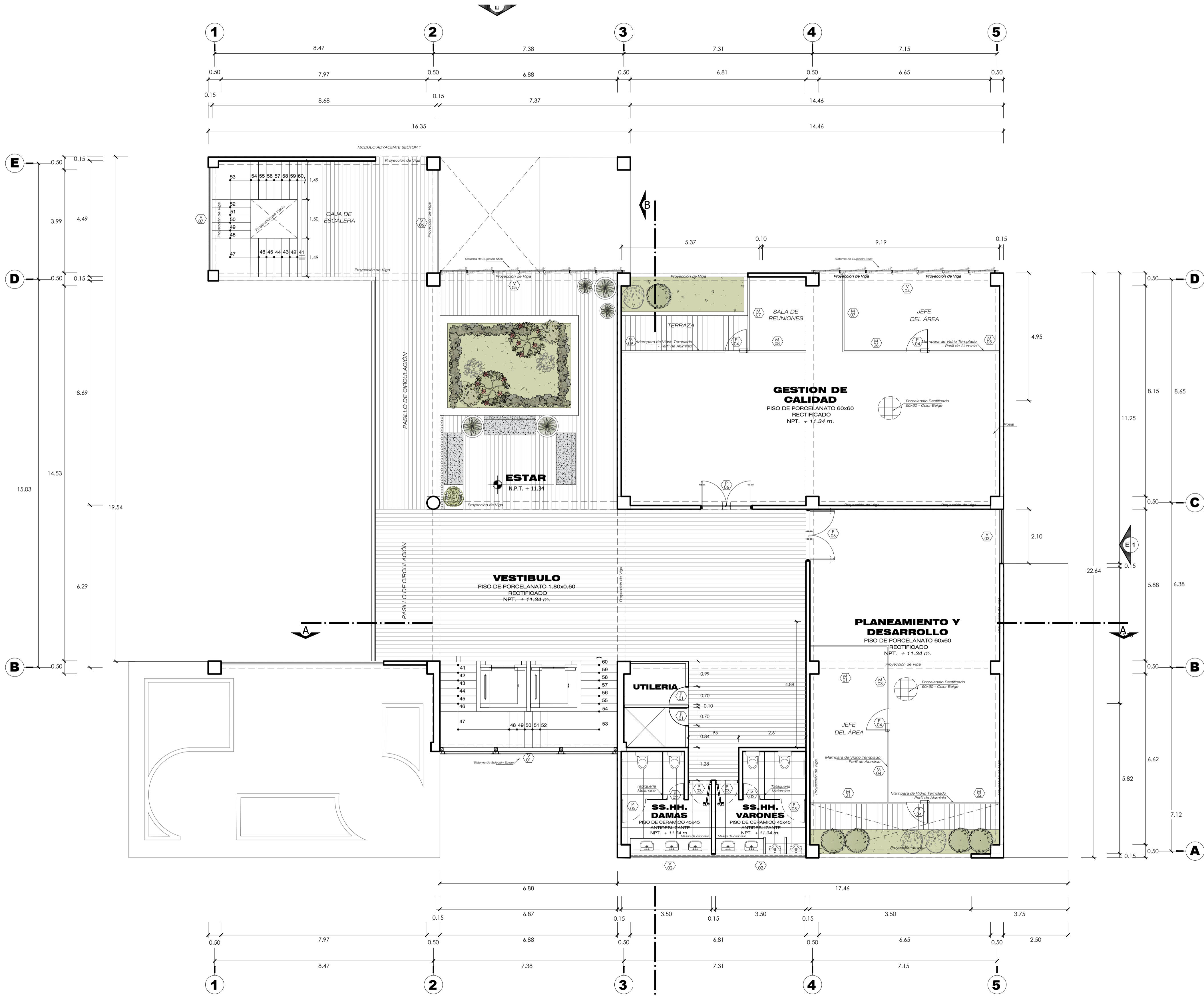
DISTRIBUCIÓN : CUARTO NIVEL SECTOR 2 ESC.: 1 / 75
