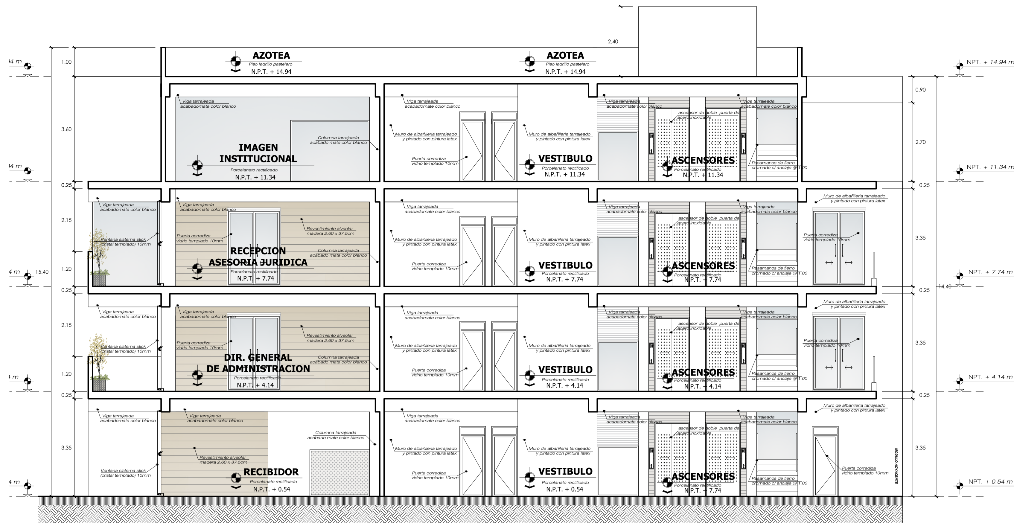
CORTE : TRANSVERSAL B - B' SECTOR 2 ESC.: 1 / 75
