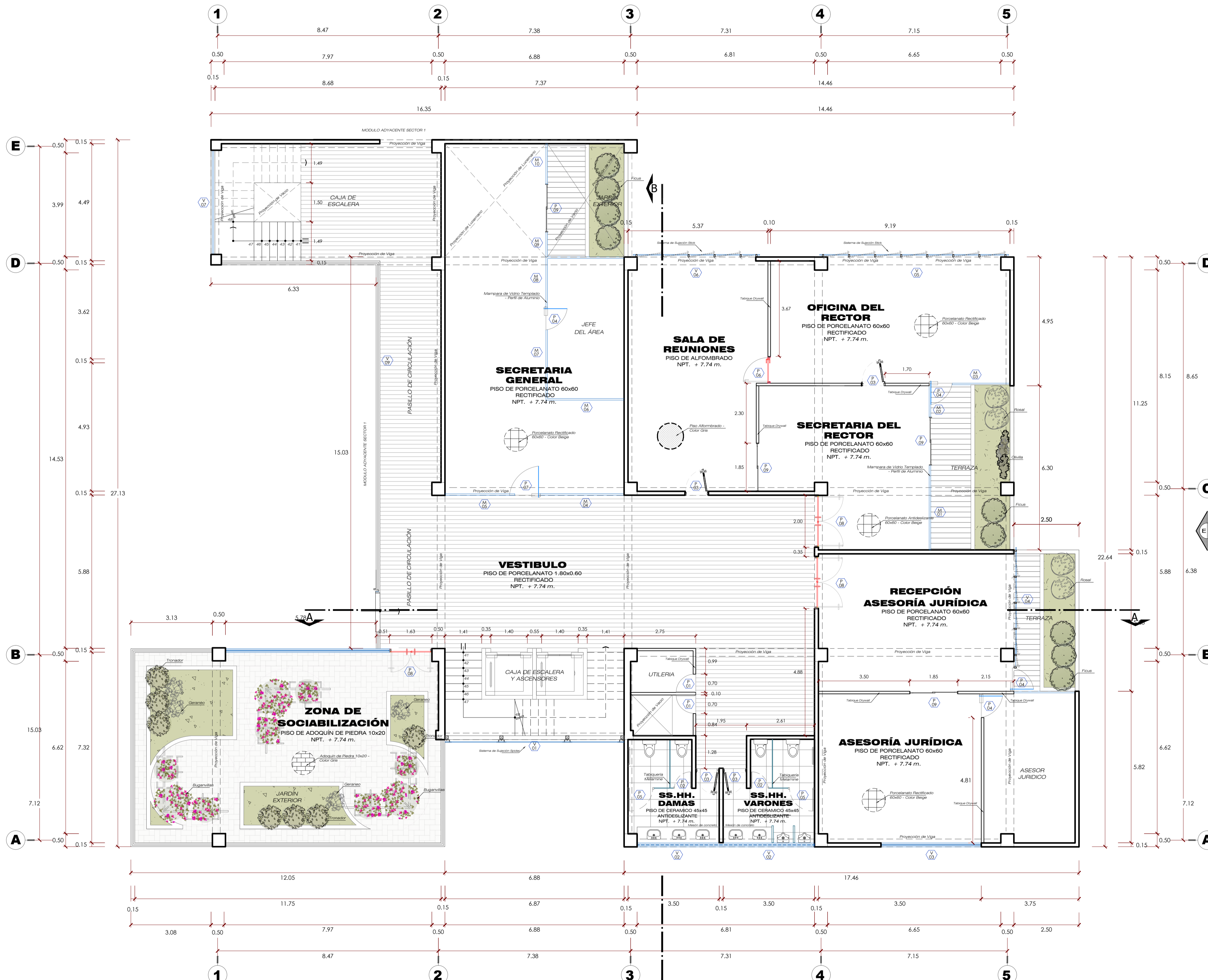
DISTRIBUCIÓN : TERCER NIVEL SECTOR 2 ESC.: 1 / 75
