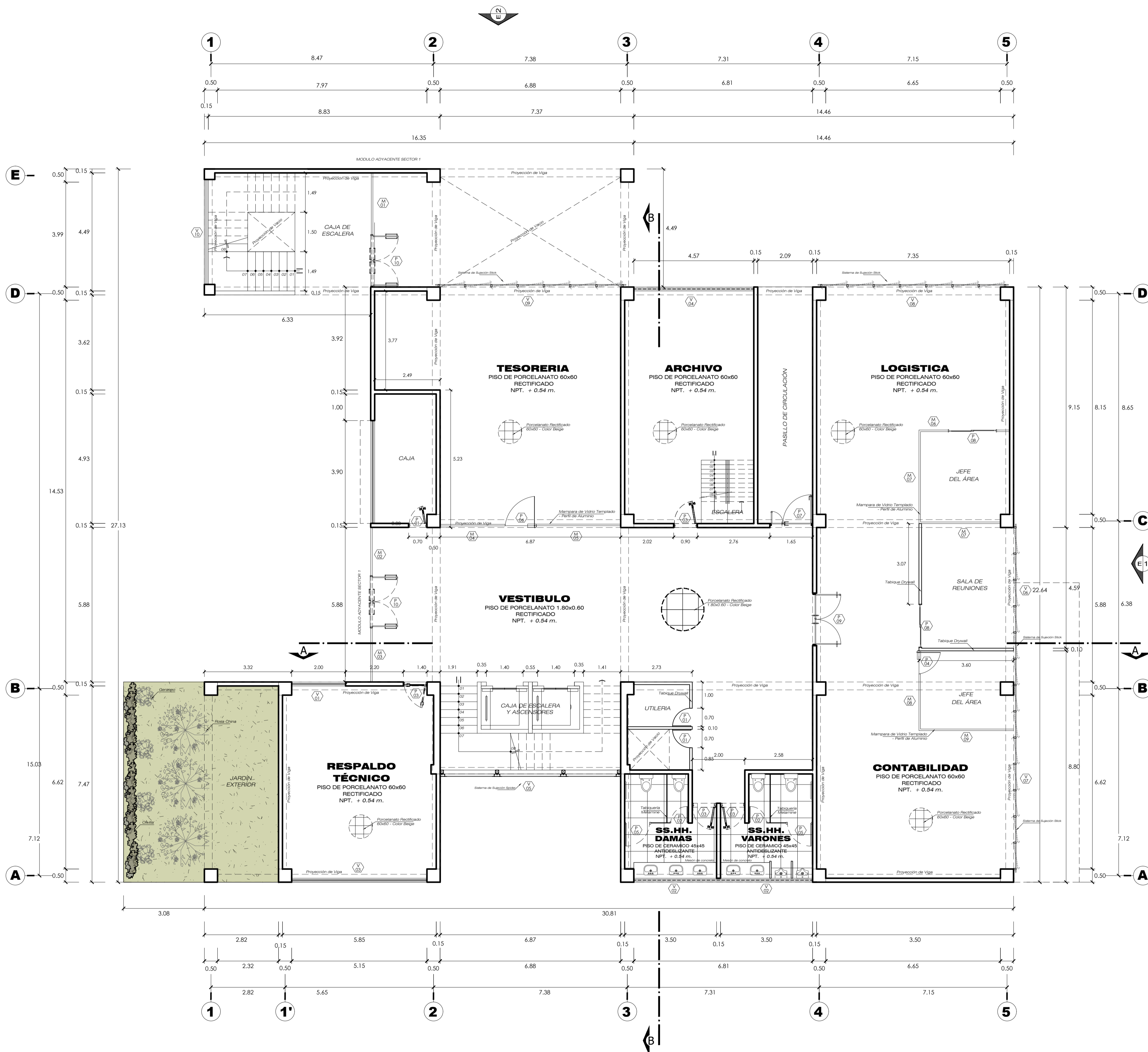
DISTRIBUCIÓN : PRIMER NIVEL SECTOR 2 ESC.: 1 / 75
