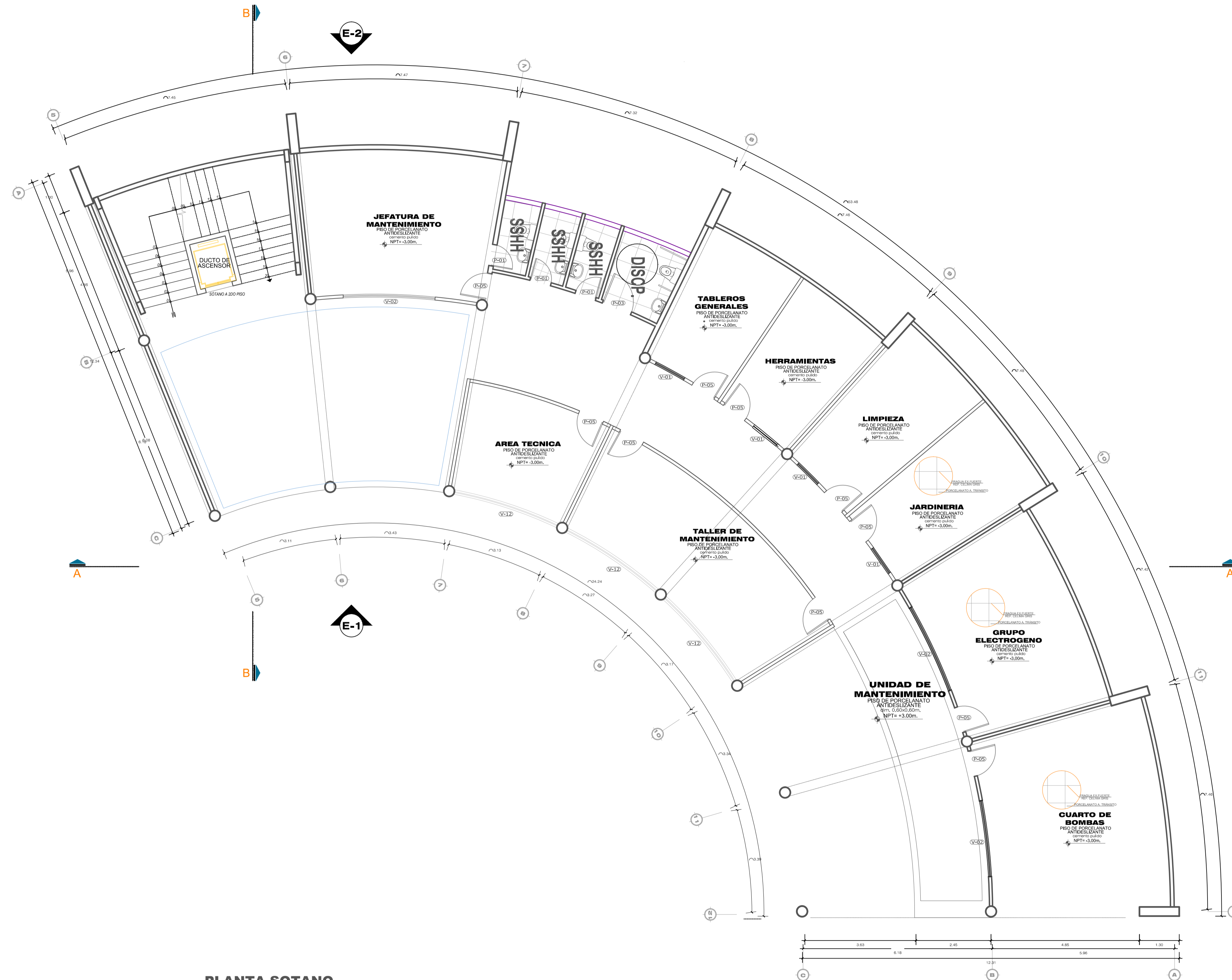
PLANTA SOTANO ESC:1/75
