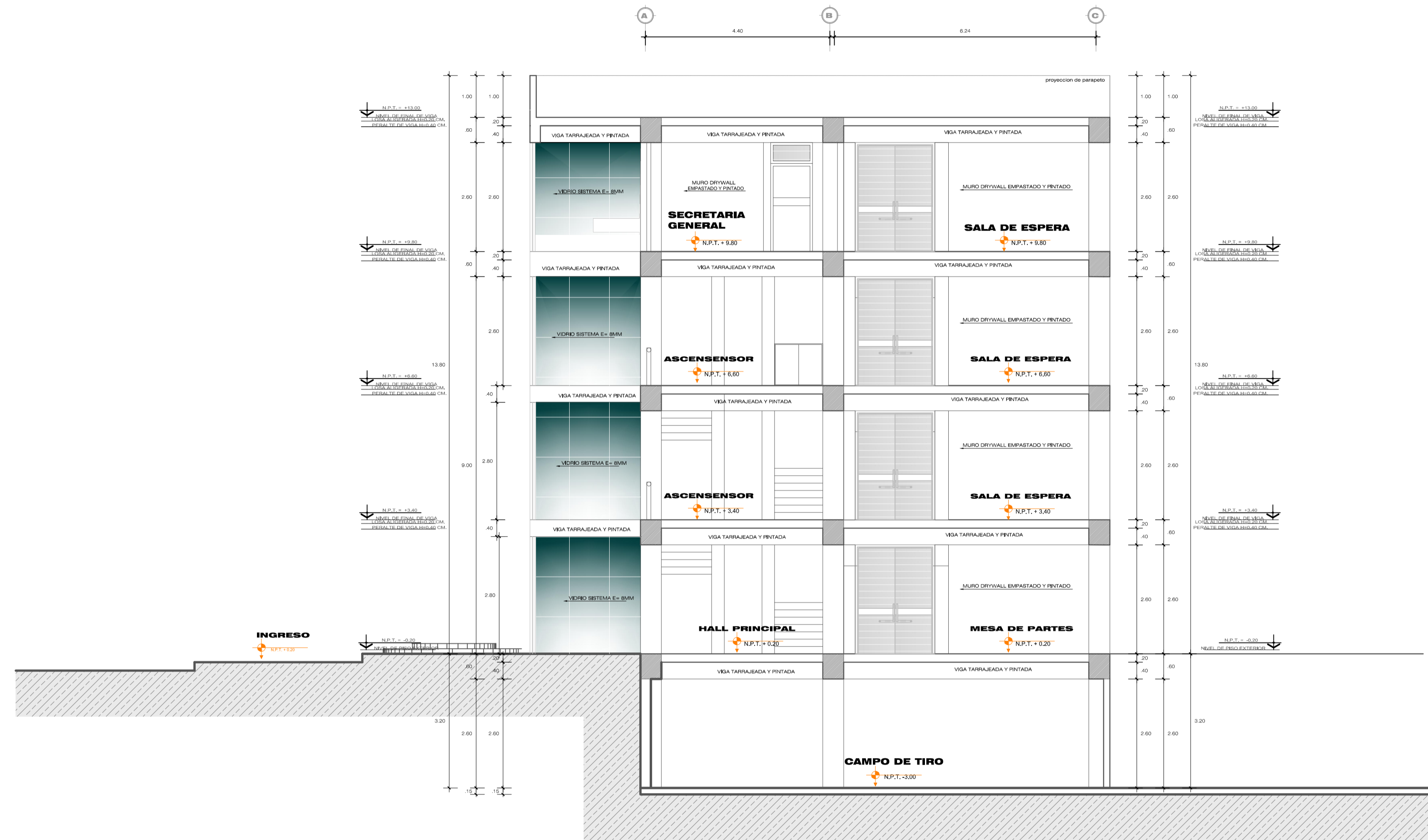
CORTE B - B ESC:1/75
