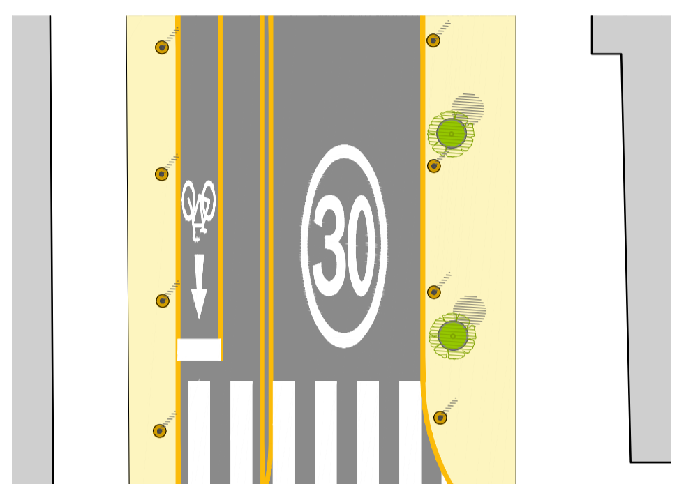
PLANTA DE INTERVENCIÓN TEMPORAL Pasaje Libertad (Próximo a Avenida Bolognesi) 1:125
