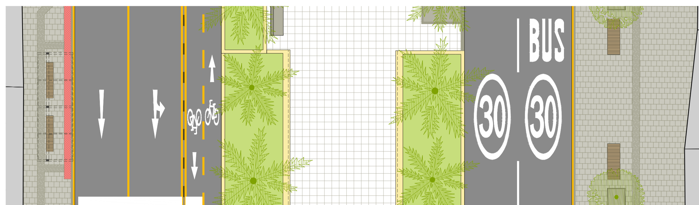
PLANTA DE INTERVENCIÓN DEFINITIVA Avenida Bolognesi 1:125
