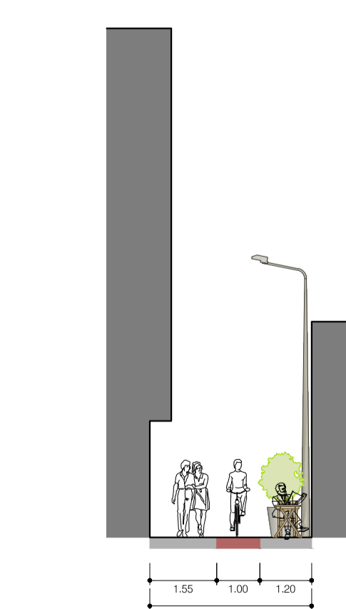
CORTE 08 - TIPO C. P. EXCLUSIVA (CPEX3) Pasaje Libertad 1:125
