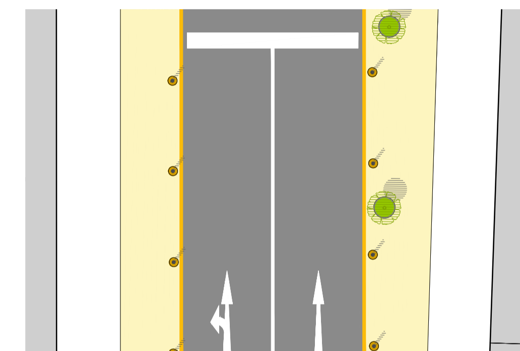
PLANTA DE INTERVENCIÓN TEMPORAL Calle Junín (Prolongación Av. Patricio Meléndez) 1:125
