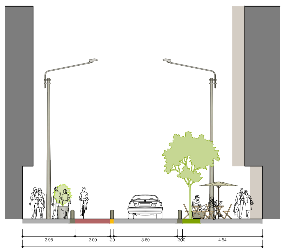
CORTE 05 - TIPO CALLE PEATONAL EVENTUAL (CPEV3) Pasaje Libertad (Próximo a Avenida Bolognesi) 1:125
