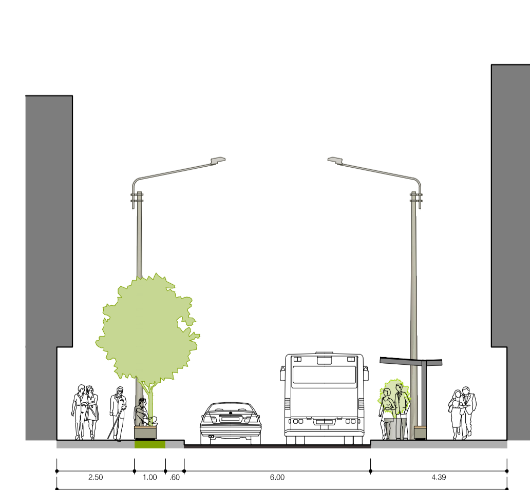
CORTE 03 - TIPO CALLE DE CONVIVENCIA (CC1) Calle Junín (Prolongación Avenida Patricio Meléndez) 1:125
