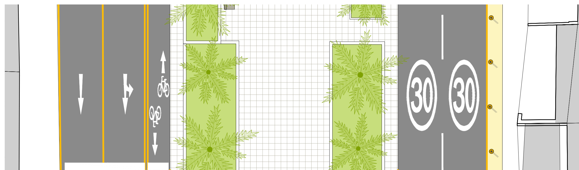
PLANTA DE INTERVENCIÓN TEMPORAL Avenida Bolognesi 1:125
