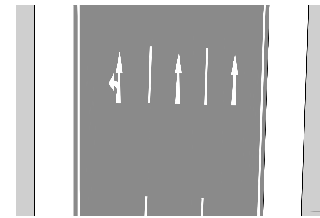
PLANTA DE ESTADO ACTUAL Calle Junín (Prolongación Av. Patricio Meléndez) 1:125
