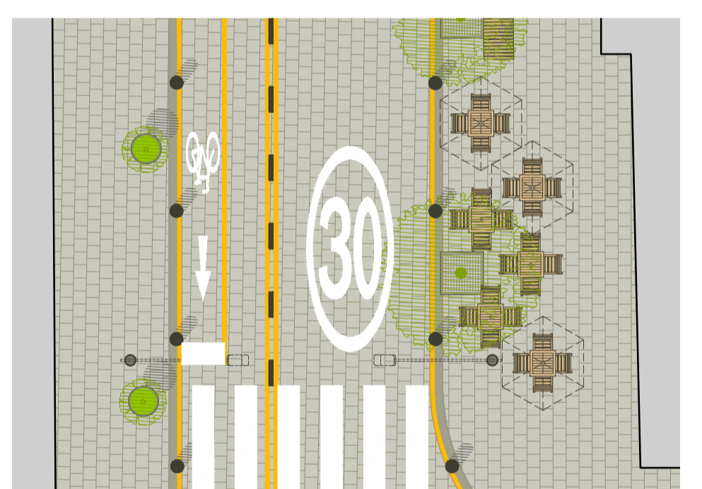
PLANTA DE INTERVENCIÓN DEFINITIVA Pasaje Libertad (Próximo a Avenida Bolognesi) 1:125
