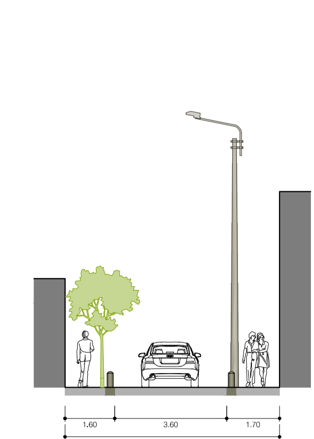
CORTE 07 - TIPO C. P. EVENTUAL (CPEV3) Calle Bolívar 1:125
