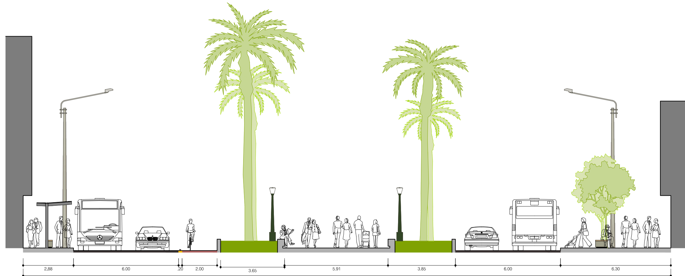
CORTE 01 - TIPO AVENIDA PARQUE (AP1) Avenida Bolognesi 1:125
