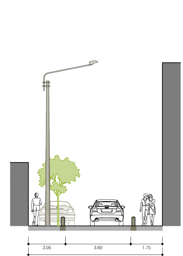
CORTE 06 - TIPO C. P. EVENTUAL (CPEV2) Calle Zela 1:125
