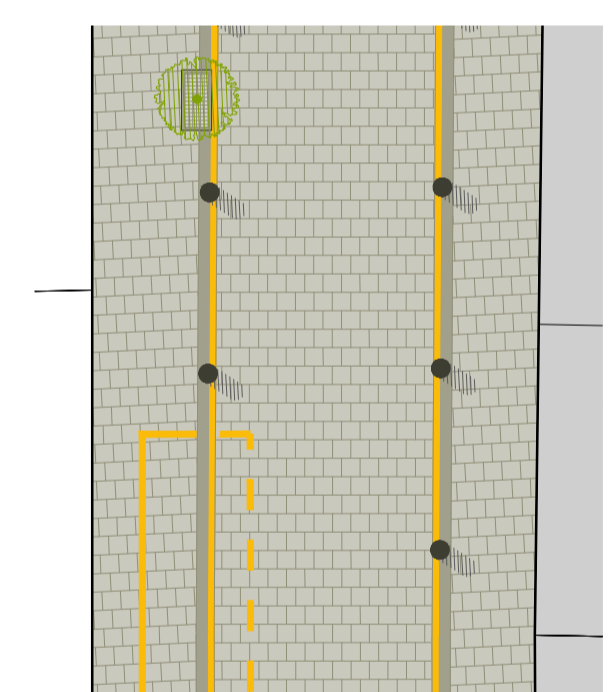
PLANTA DE INTERVENCIÓN DEFINITIVA Calle Zela 1:125
