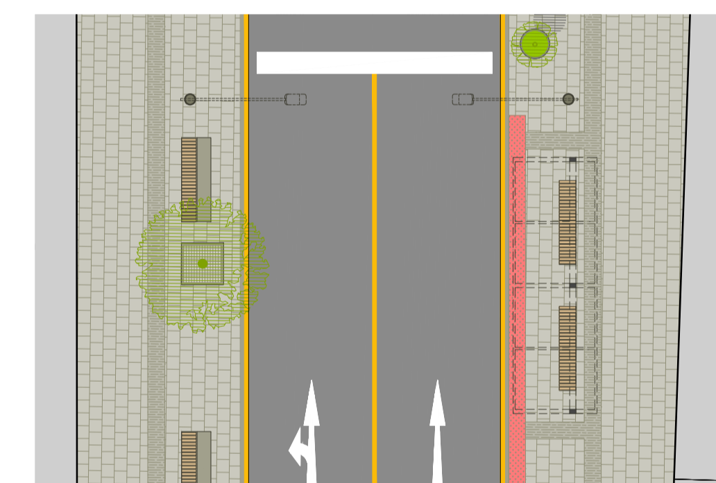
PLANTA DE INTERVENCIÓN DEFINITIVA Calle Junín (Prolongación Av. Patricio Meléndez) 1:125
