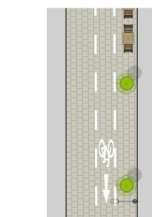
PLANTA DE INTERVENCIÓN DEFINITIVA Pasaje Libertad 1:125
