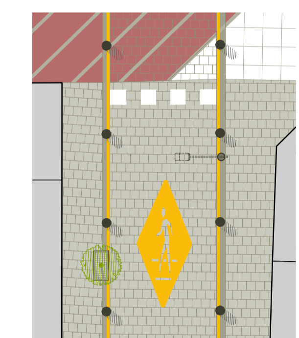
PLANTA DE INTERVENCIÓN DEFINITIVA Calle Bolívar 1:125
